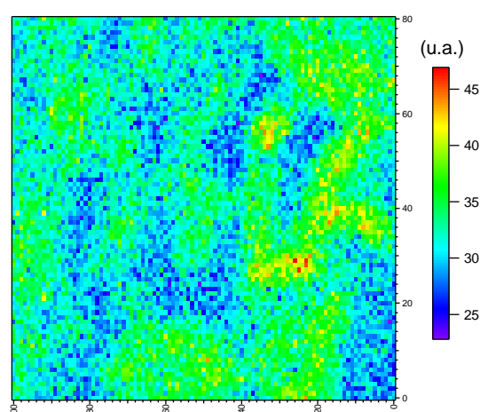
Figure 3.6: Cartographie d'intensité du niveau du cœur N1s du BN synthétisé sur Ni montrant que le BN est détecté partout sur la surface (énergie photonique 700 eV temps d'intégration 500 ms).
