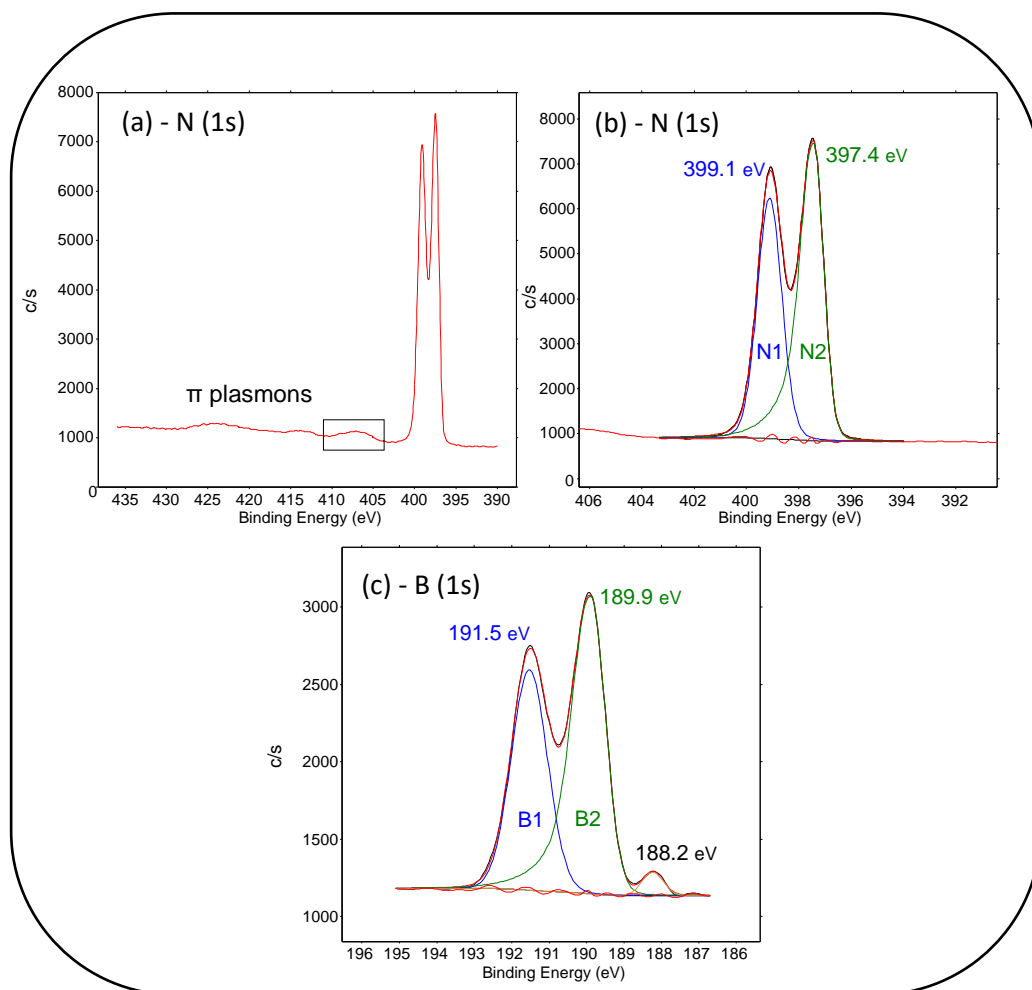
Figure 4.24: Spectres XPS des niveaux du cœur N1s (a,b) et B1s (c) obtenus après croissance de 4h à 900^{\circ}\text{C} . Le rectangle dans (a) montre la détection des \pi plasmons.
