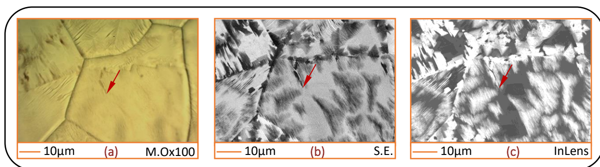
Figure 2.18: Images en microscopies optique (a) et électronique en mode S.E. (b) et InLens (c) d'une même zone après croissance de BN sur Ni. Les flèches rouges montrent le point de repère utilisé pour réaliser les mesures Raman sur les îlots de BN apparaissant avec une forte intensité en InLens (c). L'image en mode S.E. (b) permet de faire la correspondance entre images optique et électronique.
