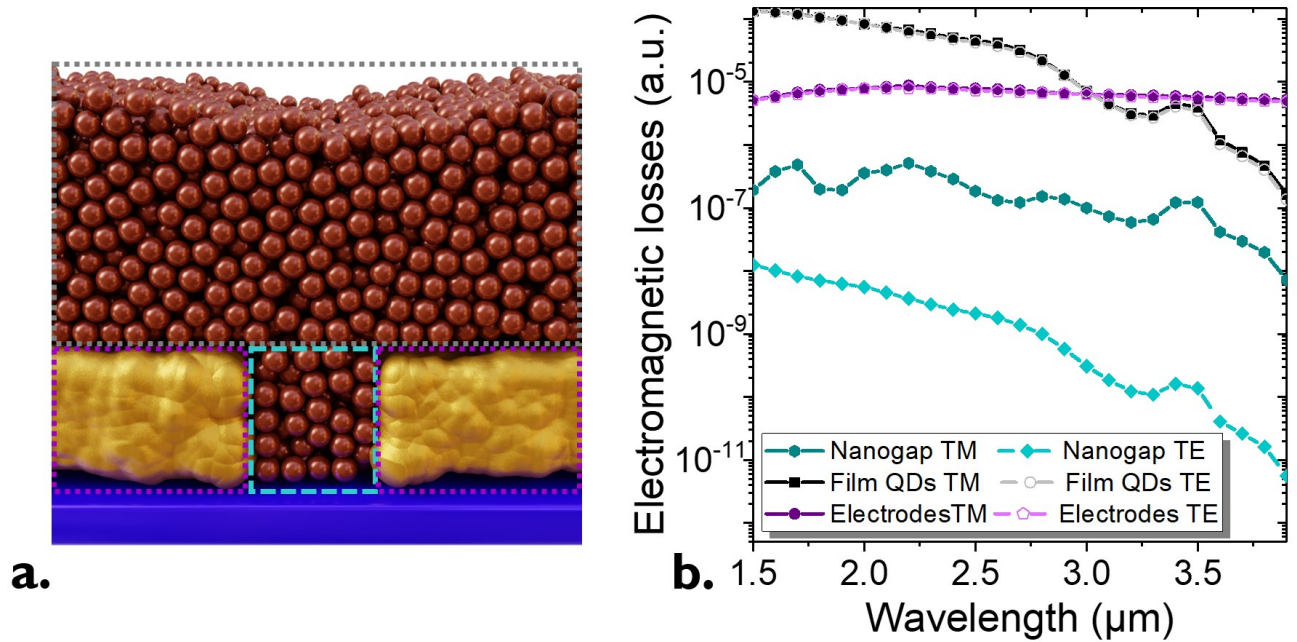
Figure 92 : Spectre d'absorption dans les différentes parties du dispositif. a. Schéma d'une nanotranchee. b. Spectre d'absorption des différents composants d'une nanotranchee de 40 nm. Les détails de cette structure sont donnés Annexe IV.
