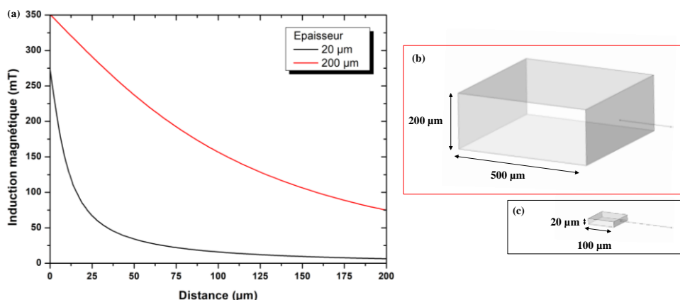
Figure 3-1 : (a) Profil de l'induction magnétique pour un aimant de largeur 100 \mu\text{m} et d'épaisseur 20 \mu\text{m} (courbe noire) représenté schématiquement sur (c) et d'un aimant de largeur 500 \mu\text{m} et d'épaisseur 200 \mu\text{m} (courbe rouge) représenté schématiquement sur (b)
