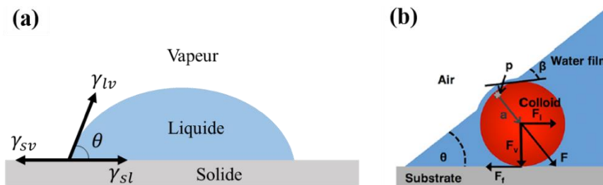
Figure 3-20 : a) Représentation schématique des énergies interfaciales mises en jeu, (b) Accumulation des particules sur un substrat due à l'évaporation d'une goutte (issu de [33])
