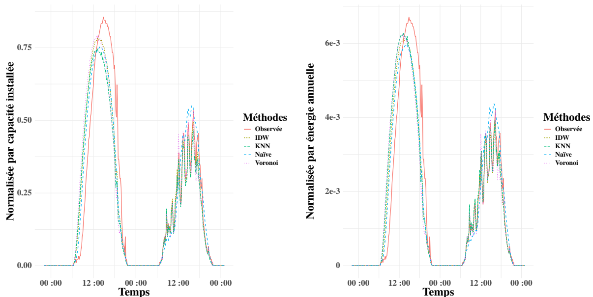
FIGURE 4.24 – Exemple d’un producteur mal estimé Sur l’axe des abscisses, nous avons les heures de deux jours d’été, et sur l’axe des ordonnées, à gauche, nous avons la production toutes les 10 minutes normalisée par la capacité installée des producteurs et à droite, nous avons la production normalisée par l’énergie annuelle
