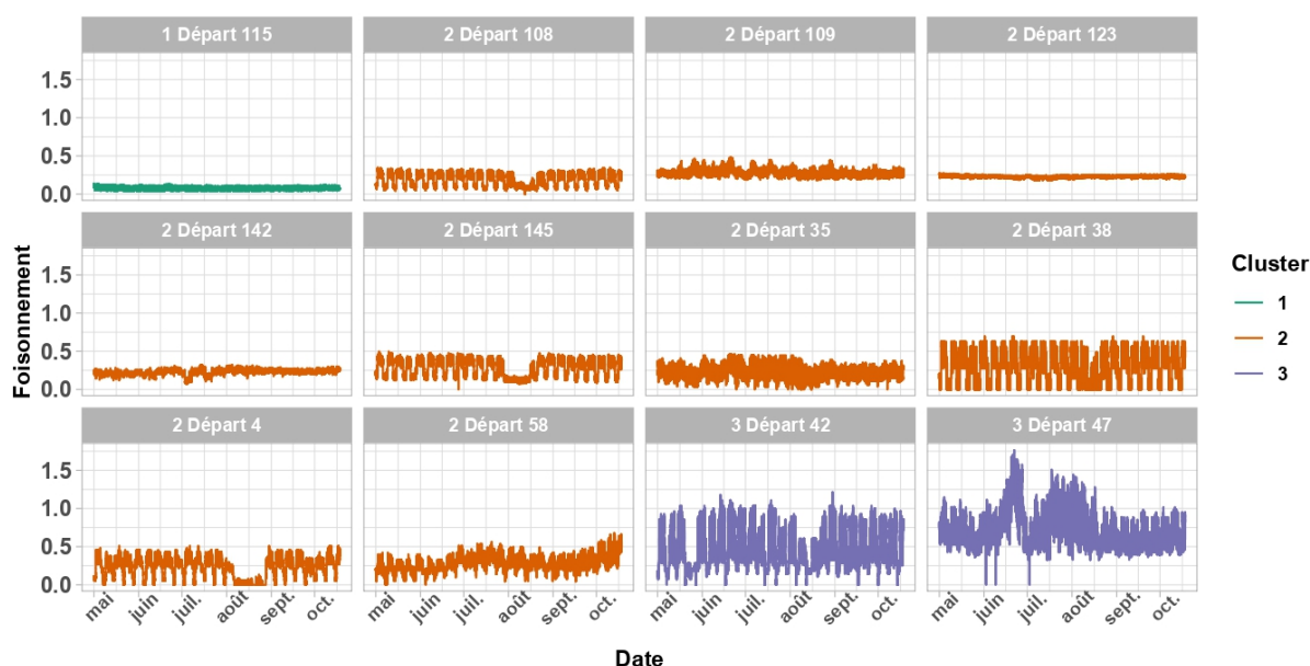
FIGURE 3.17 – Exemple de courbes de charge des départs selon le cluster. Lecture : L’axe des abscisses représente la date sur une période d’été et l’axe des ordonnées représente le foisonnement. Les blocs illustrent les courbes des départs en fonction des clusters obtenus par CAH sur la période d’été. Le cluster 1 est représenté par le départ médoïde.
