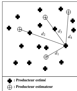
FIGURE 4.10 – Pondération par l'inverse de la distance dans le cas de quatre voisins
