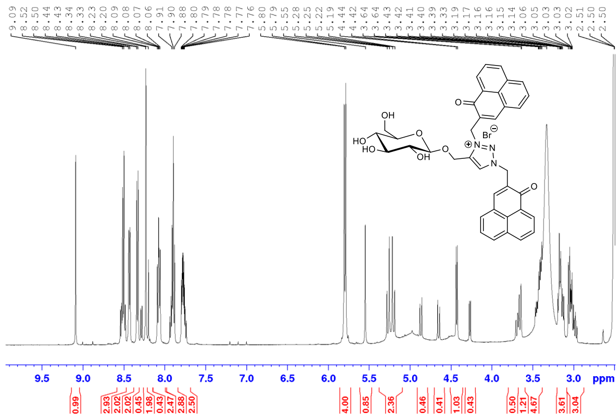
Figure A295. Spectre RMN 1 H de la PNGlc-F (contaminée par PNGlc-B) dans DMSO-d 6
