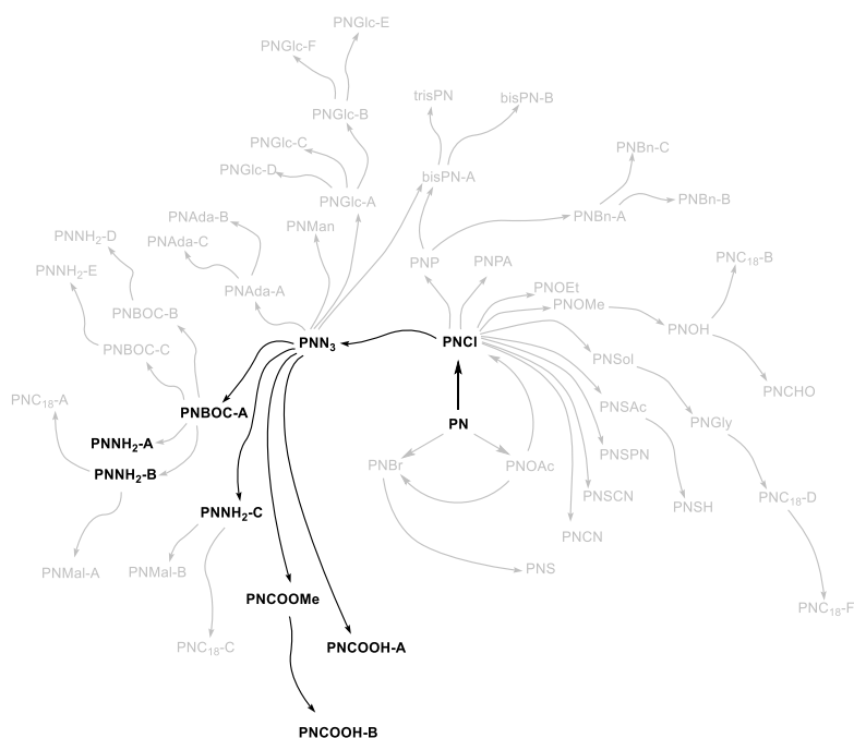
Figure 72. Résumé des voies de synthèse des composés décrits dans le chapitre II.4.2
