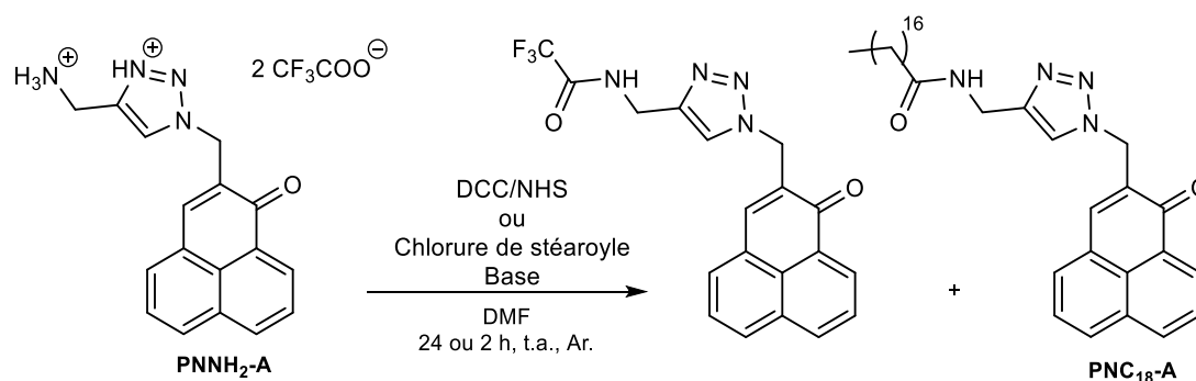
Figure 108. Synthèse de la PNC 18 -A et de son sous-produit lors du couplage peptidique avec la PNNH 2 -A
