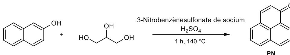
Figure 34. Synthèse de la PN (méthode A)
