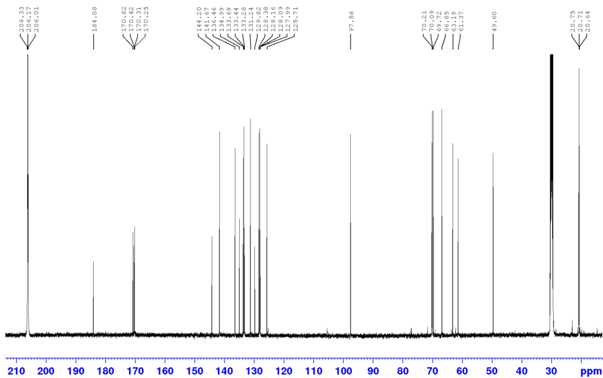
Figure A299. Spectre RMN ^{13}\text{C} de la PNMan- \alpha dans acétone- \text{d}_6
