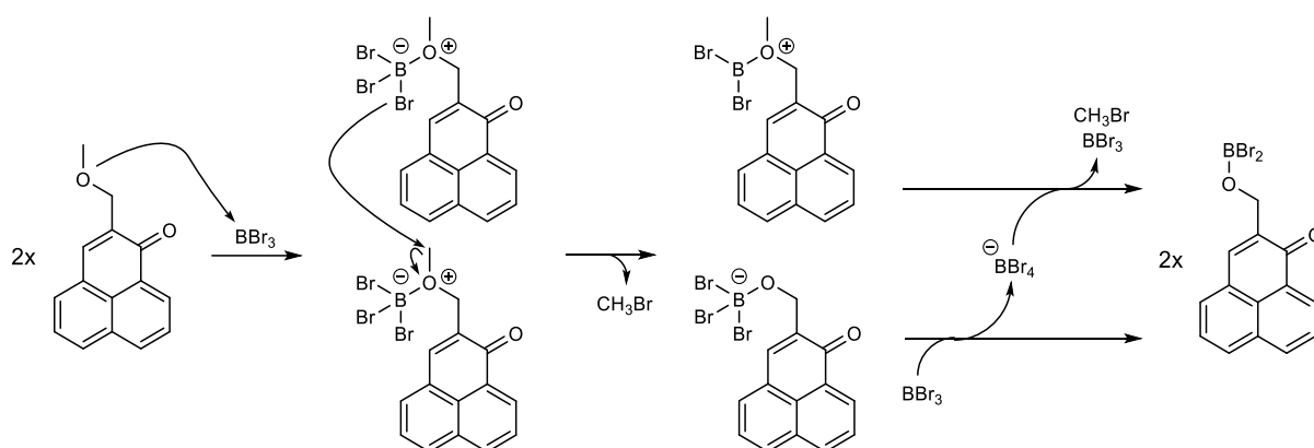
Figure 60. Mécanisme réactionnel de la déméthylation de la PNOMe par \text{BBr}_3
