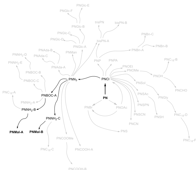
Figure 87. Résumé des voies de synthèse des composés décrits dans le chapitre III.2
