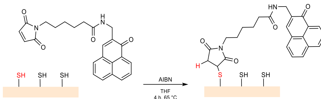
Figure 92. Réaction d'addition thiol-ène entre la PNMal et le bois/papier
