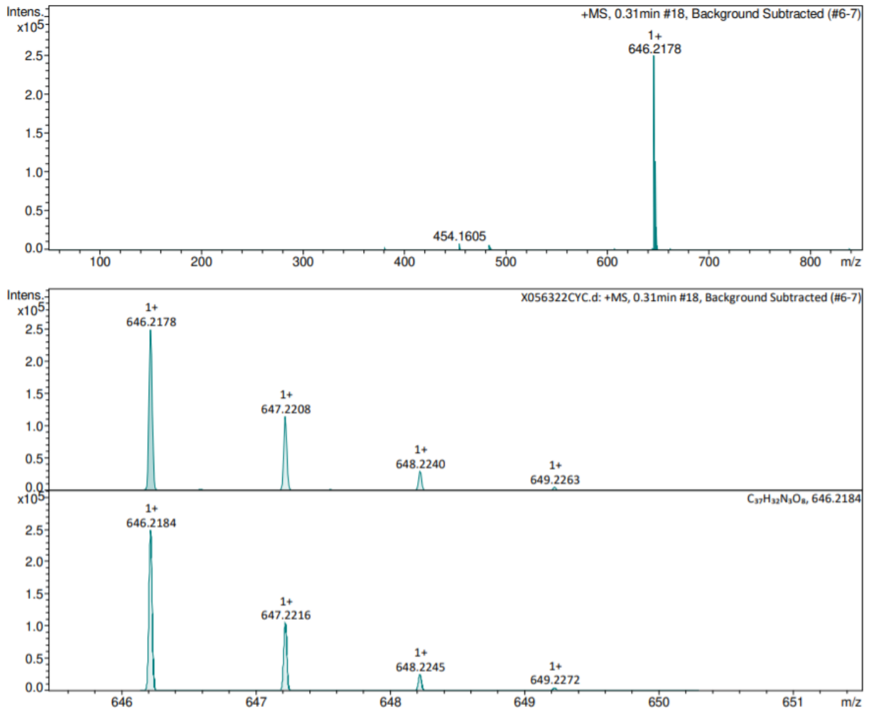
Figure A297. Spectre HRMS (ESI + ) de la PNGlc-F
