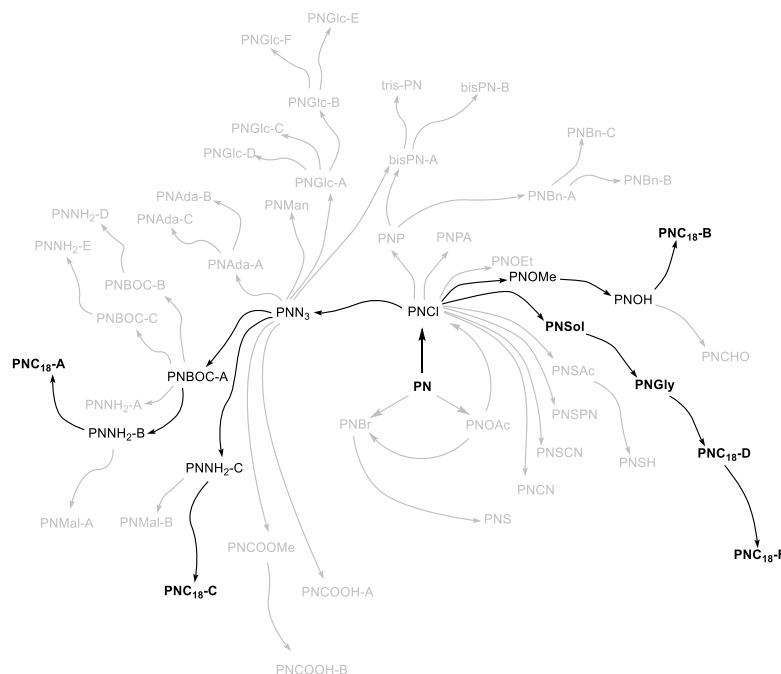
Figure 107. Résumé des voies de synthèse des composés décrits dans le chapitre IV
