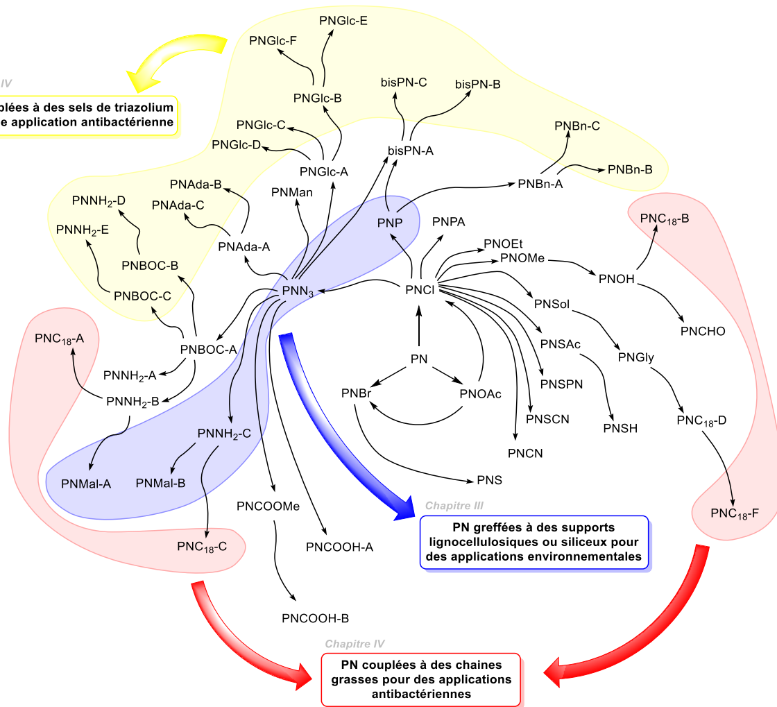
Figure 33. Synthèses décrites et objectifs de la thèse
