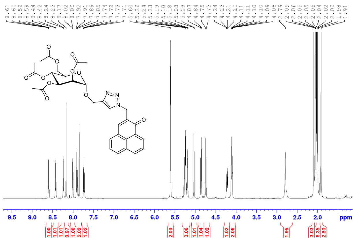
Figure A298. Spectre RMN ^1\text{H} de la PNMan- \alpha dans acétone- \text{d}_6
