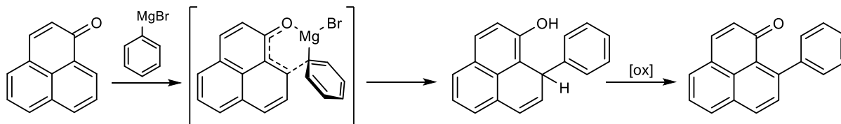
Figure 21. Réaction de Grignard sur la PN
