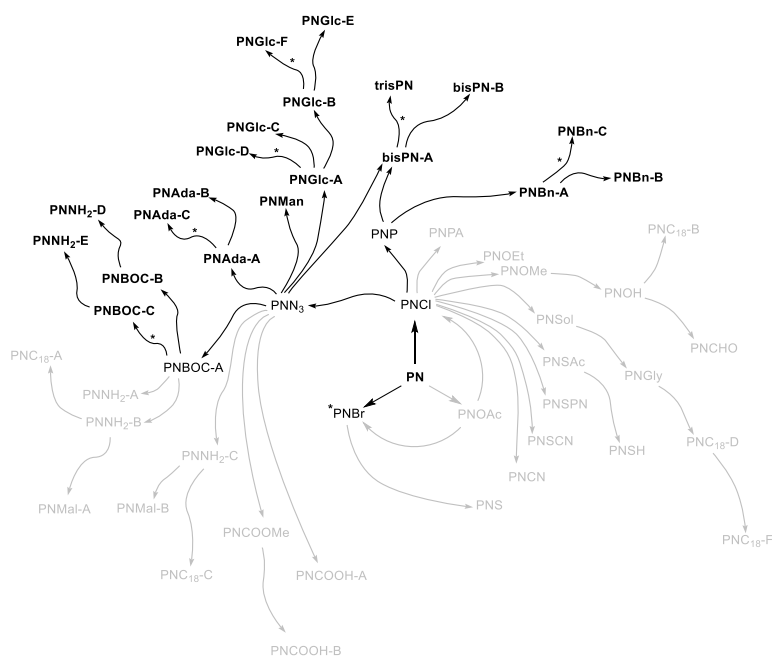
Figure 129. Résumé des voies de synthèses des composés décrits dans le chapitre V
