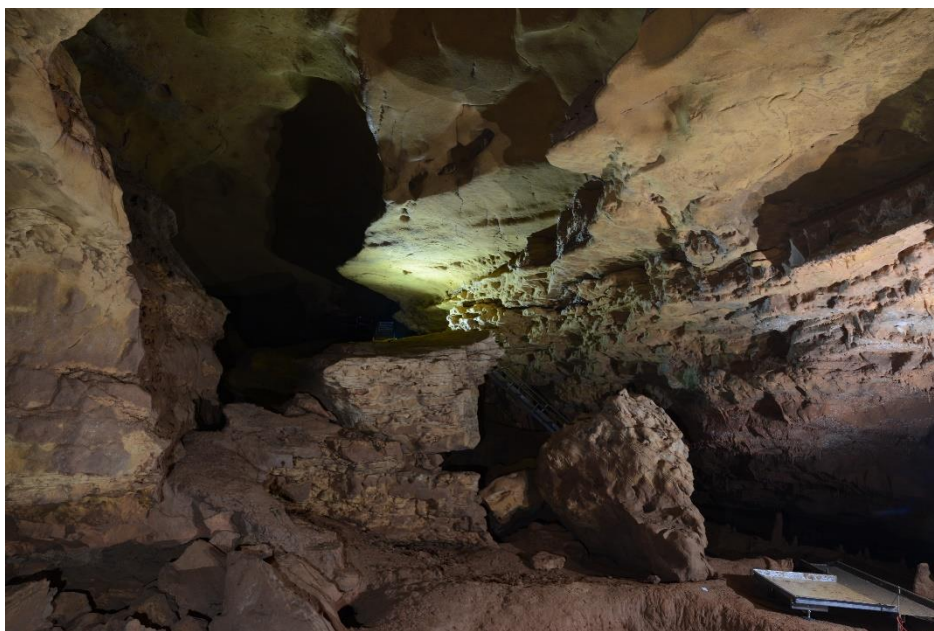
Figure 122 : Panneau de la Découverte observé depuis l’entrée amont de la Salle éponyme et éclairé depuis l’aval par une lampe frontale moderne (cl. . V. Feruglio, C. Bourdier /MC).
