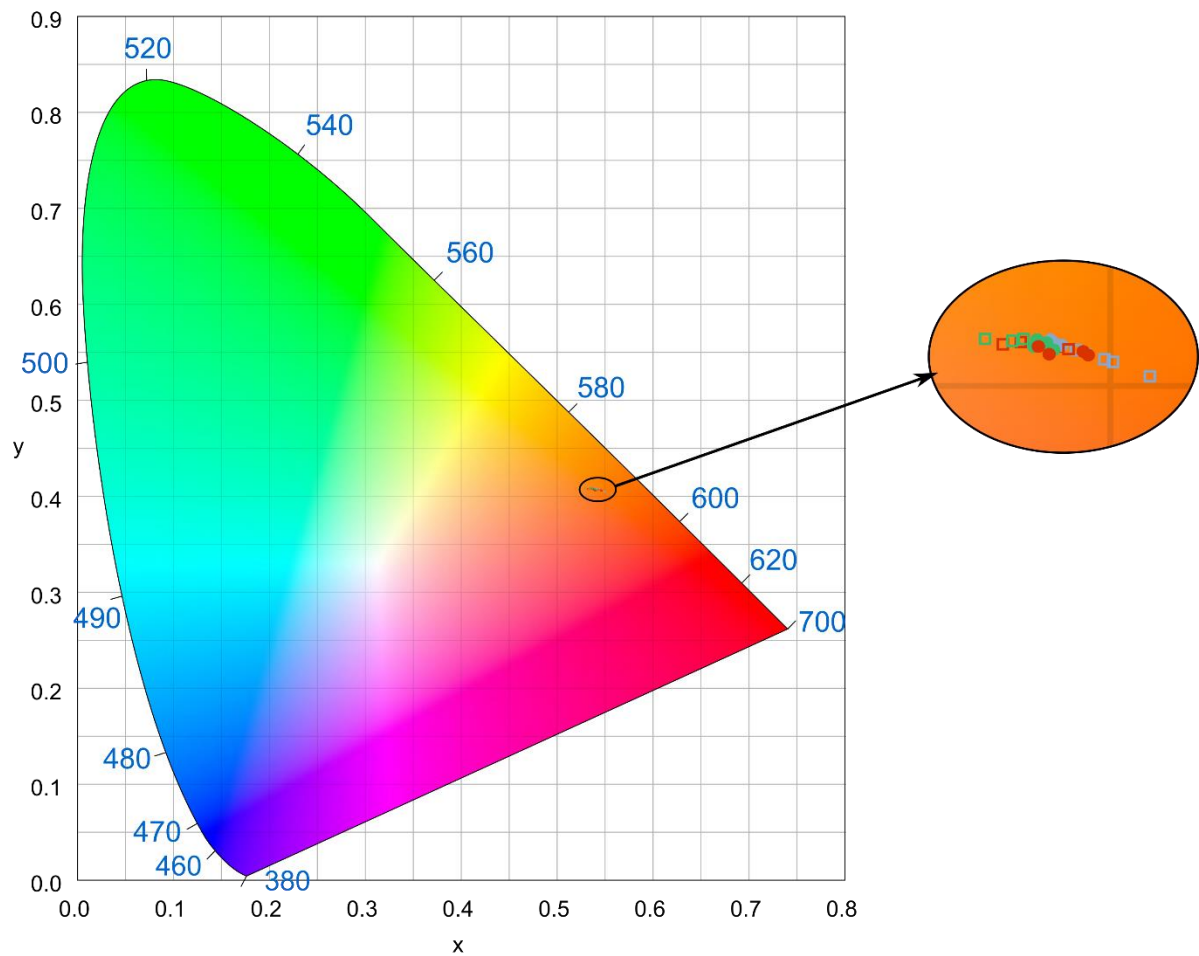
Figure 82 : Localisation des spectres des lampes à graisse sur le diagramme de chromaticité CIE xy.
