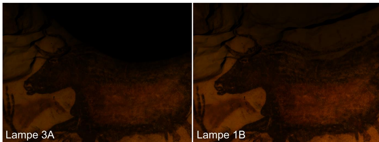
Figure 179 : Simulation numérique à partir de la méthode de calcul du modèle d'illumination élémentaire réalisée avec le logiciel Phanie et le modèle numérique du Diverticule Axial Perazio Engineering, modifié par l'équipe MicroPaGO : simulation d'éclairage avec une lampe à graisse de type 3A (à gauche) ou de type 1B (à droite) sur le Grand Taureau Noir, accompagné d'une Vache Rouge et de quatre Protomés d'Aurochs Jaunes. Distance entre la caméra et la paroi d'environ 1,20 m. Saturation de 30 000.
