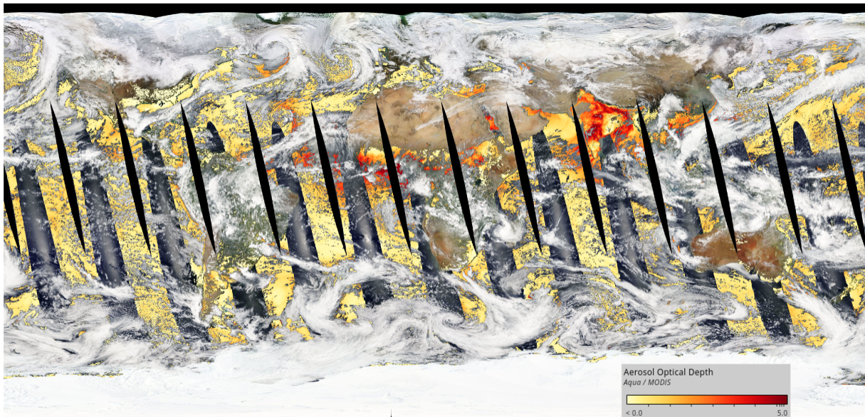
FIGURE 4.14: Réflectance mesurée par l’instrument MODIS/Aqua avec l’épaisseur optique d’aérosols pour la journée du 1 er janvier 2008. Figure obtenue à partir de l’outil de visualisation de données satellites en ligne de la NASA WorldView ( https://worldview.earthdata.nasa.gov/ , dernier accès le 30 juin 2021).
