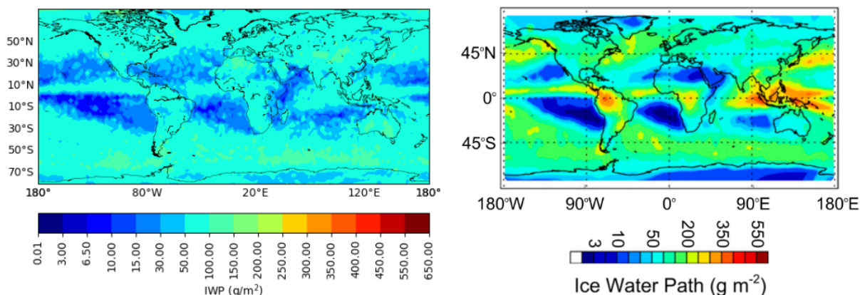
FIGURE 4.20: IWP moyens restitués par notre algorithme (à gauche) et par DARDAR (à droite, figure de Hong and Liu (2015)).
