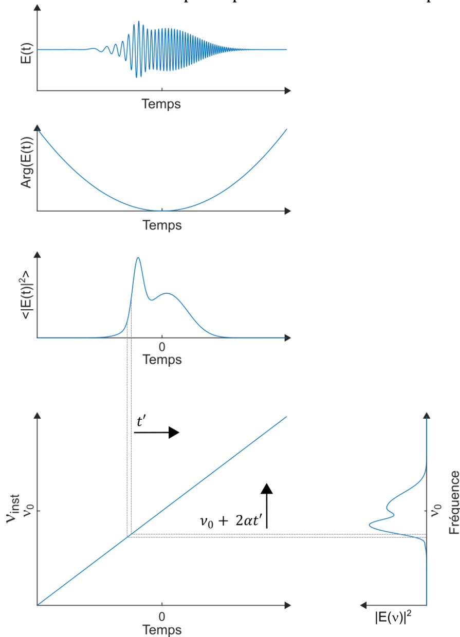
Figure 4.11 - Une impulsion du champ électrique de forme quelconque est modulée en phase quadratiquement au cours du temps, la fréquence instantanée du champ évolue donc linéairement dans le temps. La puissance optique aux alentours d'un instant t' se retrouve autour de \nu_0 + 2\alpha t' dans le spectre, et une image de l'impulsion se forme dans le domaine fréquentiel.
