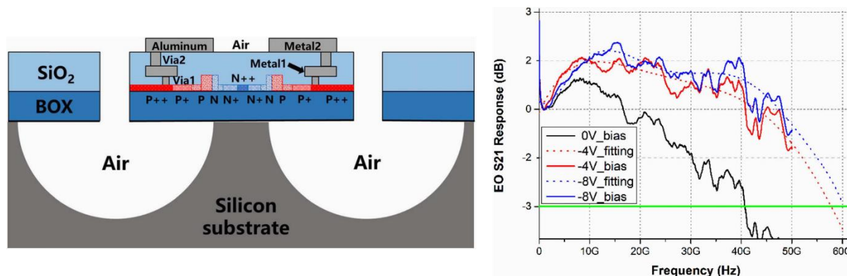
Figure 3.10 - Vue en coupe schématique d'un SPP-MZM dont le substrat de silicium a été gravé. La fonction de transfert mesurée montre une bande passante supérieure à 50 GHz pour une tension de polarisation de -4 V. Figure issue de [111].
