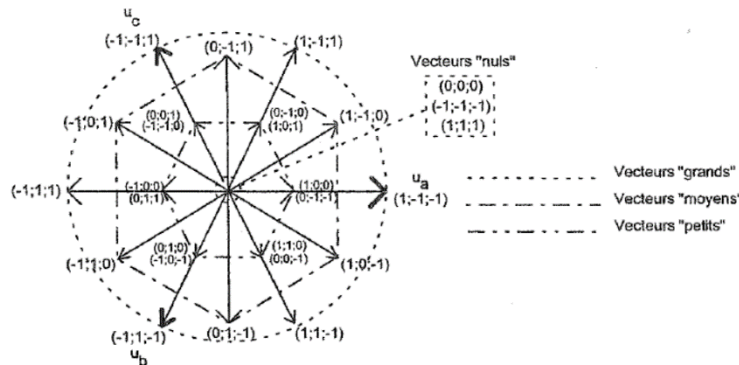
Figure 3. 16: Représentation vectorielle du redresseur trois niveaux.
