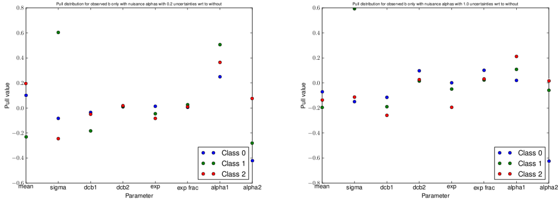
FIGURE 7.26 – Valeur du pull défini comme la différence entre la valeur Combine obtenue dans l’hypothèse de bruit de fond seul et la valeur centrale obtenue après ajustement de la fonction dCB+exp sur les simulations DY divisée par l’incertitude systématique associée pour les paramètres de la fonction dCB+exp. Les incertitudes systématiques considérées pour \alpha_{R/L} sont 0,2 à gauche et 1,0 à droite pour 2018.
