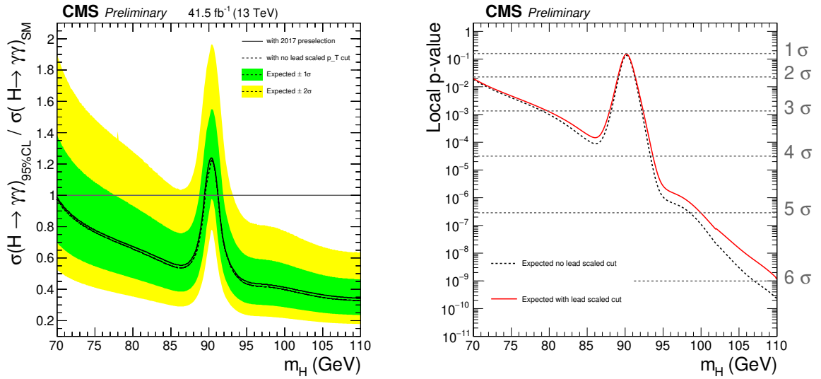
FIGURE 7.9 – Limites d'exclusion attendues sur le produit section efficace fois rapport de branchement en deux photons normalisé pour un boson de Higgs additionnel (gauche) et p-value locale attendue (droite) en fonction de la masse d'un tel boson jusqu'à 110 GeV pour 2017 sans coupure sur p_T^{(1)}/m_{\gamma\gamma} .
