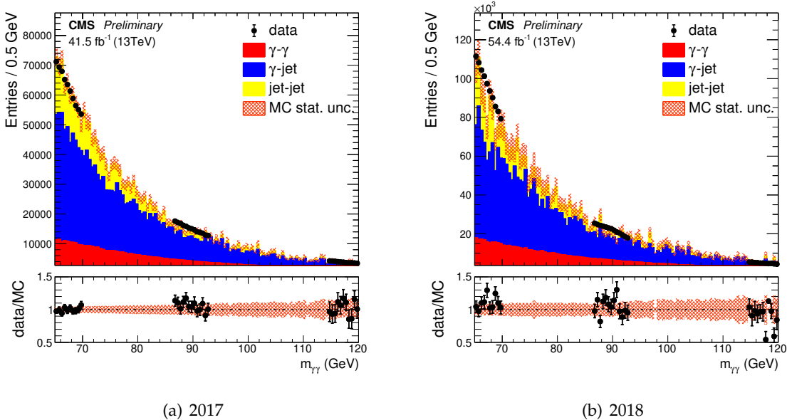
FIGURE D.1 – Distributions de masse invariante diphoton pour a) 2017 et b) 2018. Les évènements dans des fenêtres de masse entre 70 \text{ GeV} < m_{\gamma\gamma} < 87 \text{ GeV} et 93 \text{ GeV} < m_{\gamma\gamma} < 115 \text{ GeV} sont cachés. Les simulations sont normalisées au nombre d'évènements dans les données.
