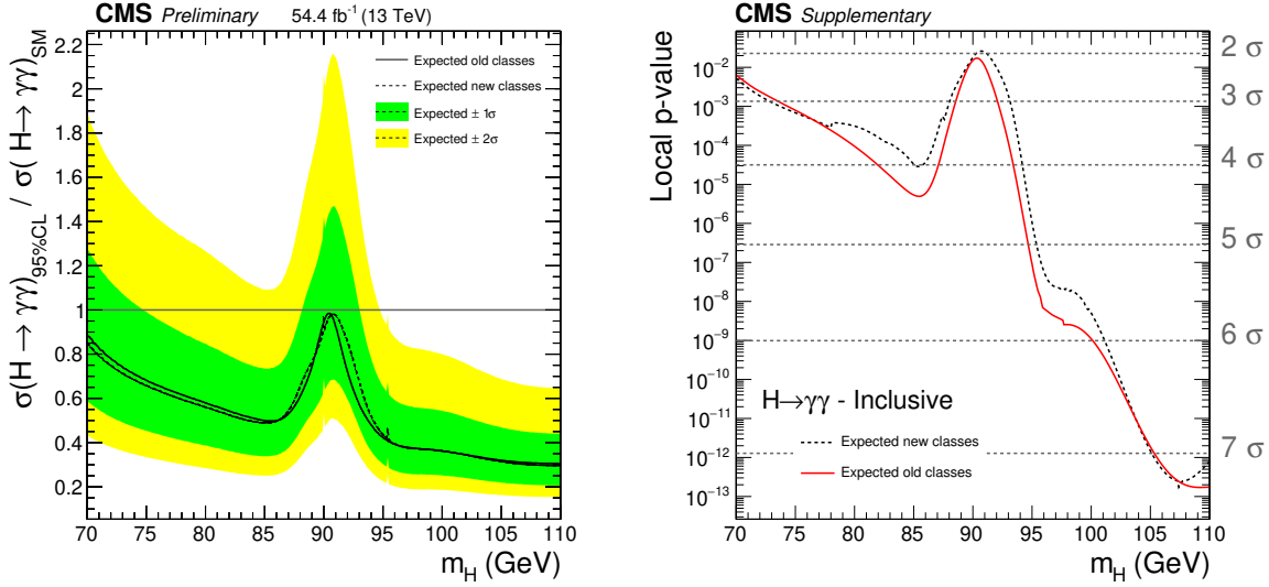
FIGURE 7.17 – Limites d'exclusion attendues sur le produit section efficace fois rapport de branchement en deux photons normalisé pour un boson de Higgs additionnel (gauche) et p-value locale attendue (droite) en fonction de la masse d'un tel boson pour la nouvelle classification 2018.
