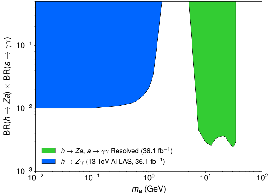
FIGURE 8.2 – Limites d'exclusion à 95 % sur BR(h \rightarrow Za) \times BR(a \rightarrow \gamma\gamma) dans notre analyse diphotons résolus (en vert) et dans le cas h \rightarrow Z\gamma où les deux photons ne sont pas discernables (en bleu) au LHC à 13 TeV pour une luminosité de 36.1 \text{ fb}^{-1} .
