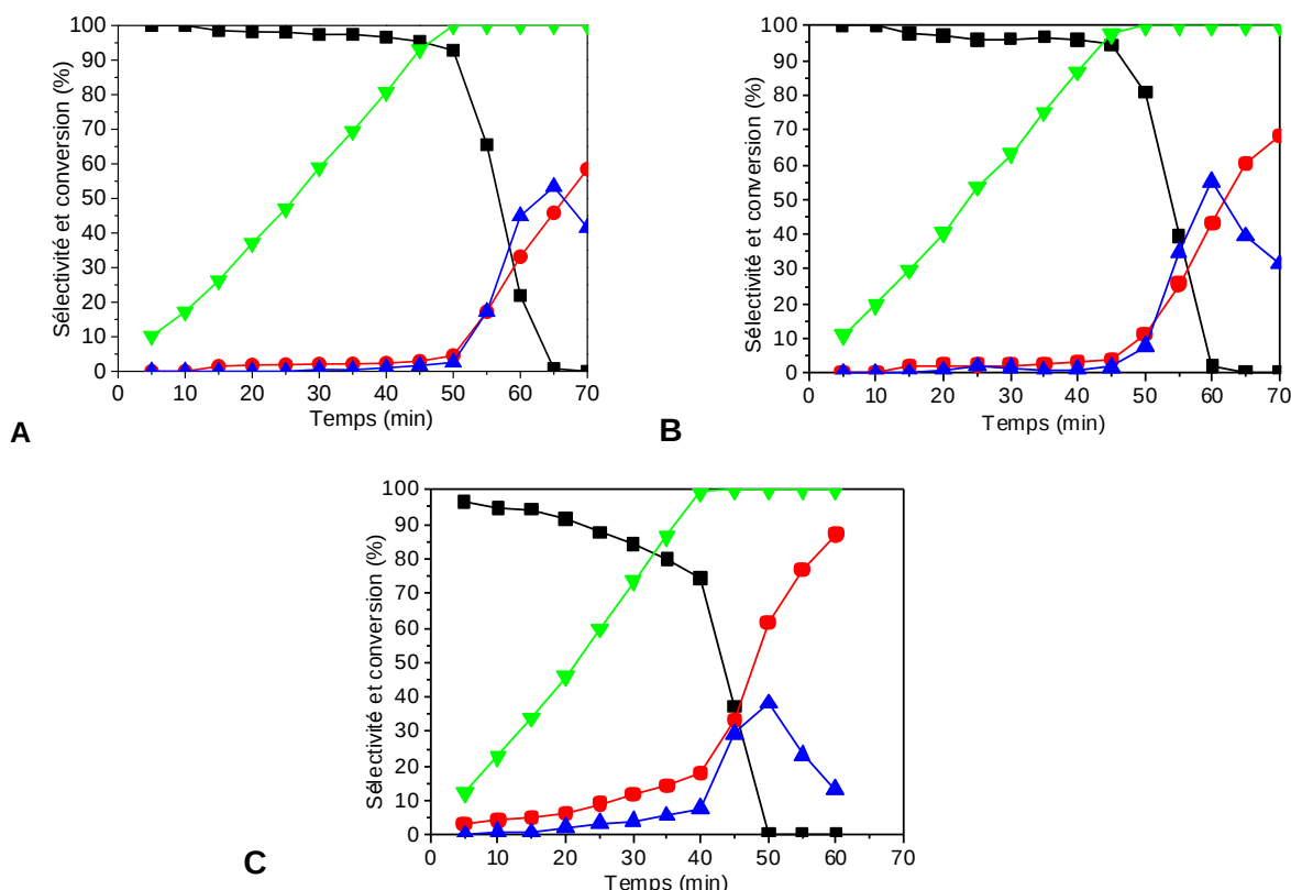
Figure 7. Semi-hydrogénation du 1-heptyne : (A) Catalysée par 1 , (B) Catalysée par 2 , et (C) Catalysée par 4 . En vert la conversion du 1-heptyne, en noir la sélectivité en 1-heptène, en rouge la sélectivité en heptane et en bleu la sélectivité en 2- et 3-heptène.
