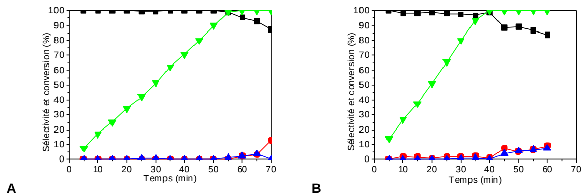
Figure 9. Semi-hydrogénation du 3-hexyne catalysée par \text{Pd}_{\text{NH}_3}(1\%)/\text{C} ( 1 ) sous flux de \text{H}_2 de (A) 2,5 mL/min et (B) 13,0 mL/min. En vert la conversion du 3-hexyne, en noir la sélectivité en 3-hexène, en rouge la sélectivité en hexane et en bleu la sélectivité en 1- et 2-hexène.
