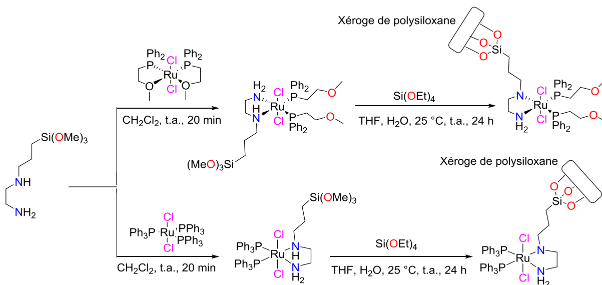
Schéma 16. Synthèse et immobilisation de catalyseurs de type \text{trans-}[\text{RuCl}_2(\text{P})_2(\text{N})_2] sur xérogel de polysiloxane.
