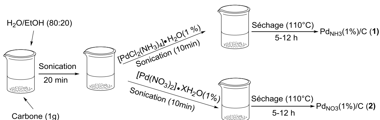
Figure 1. Préparation de \text{Pd}_{\text{NO}_3}(1\%)/\text{C} (1) et \text{Pd}_{\text{NH}_3}(1\%)/\text{C} (2) par sonication.
