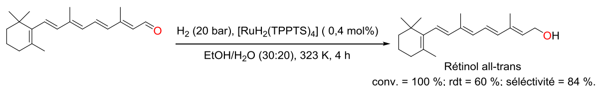
Schéma 12. Réduction du rétirol par hydrogénation catalytique avec [\text{RuH}_2(\text{TPPTS})_4] .
