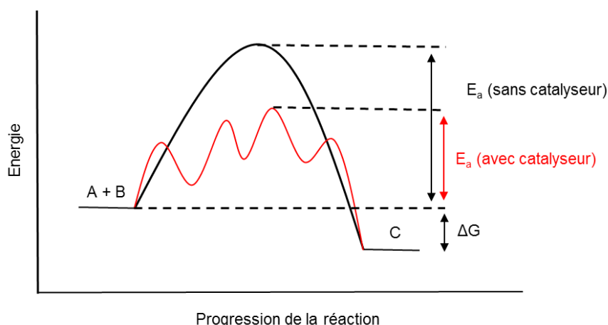
Figure 1. Chemin énergétique de la réaction de A + B conduisant à C avec (rouge) et sans (noir) catalyseur. L'énergie d'activation globale ( E_a ) est abaissée par l'action du catalyseur sans changer l'énergie globale \Delta G ou le produit de la réaction. 2
