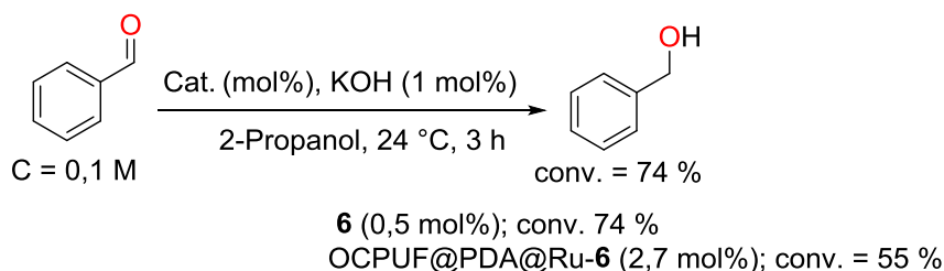
Schéma 21. Hydrogénation par transfert du benzaldéhyde catalysée par 6 et OCPUF@PDA@Ru-6.
