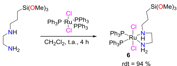
Schéma 17. Synthèse du complexe 6 .
