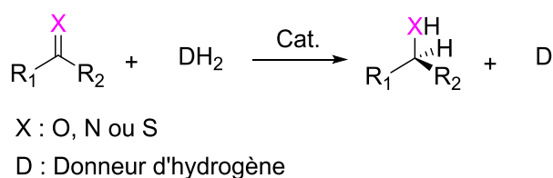
Schéma 20. Hydrogénation par transfert.
