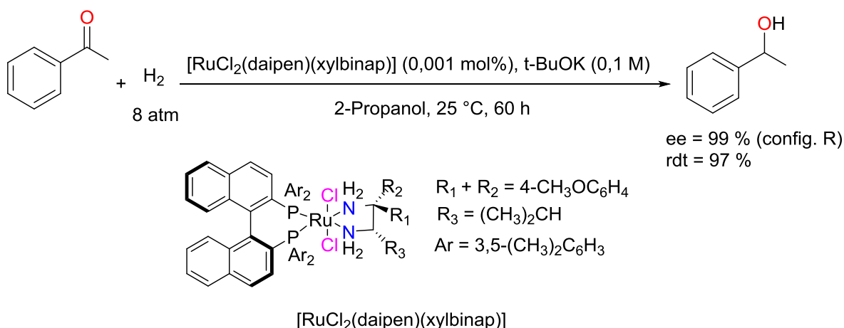
Schéma 15. Hydrogénation asymétrique de l'acétophénone par [\text{RuCl}_2(\text{daipen})(\text{xylbinap})] . 75
