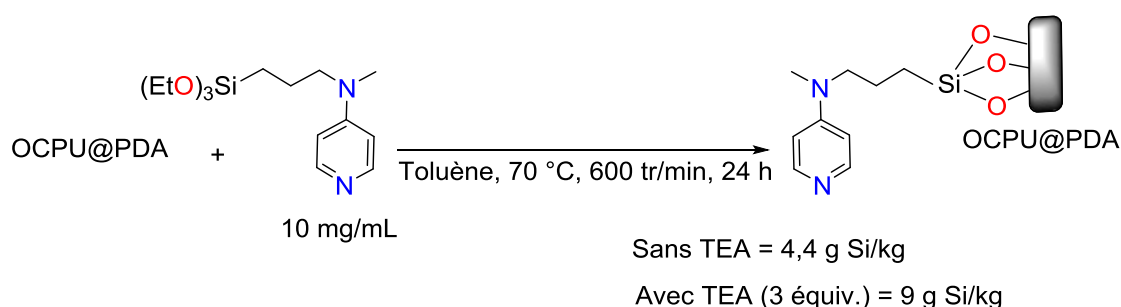
Schéma 20. La fonctionnalisation d'OCPUF@PDA par DMAP-TES avec et sans TEA.
