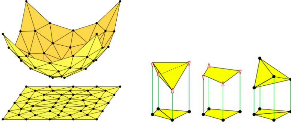
FIGURE 14. Une triangulation du carré donnée par une fonction convexe, et un flip.
