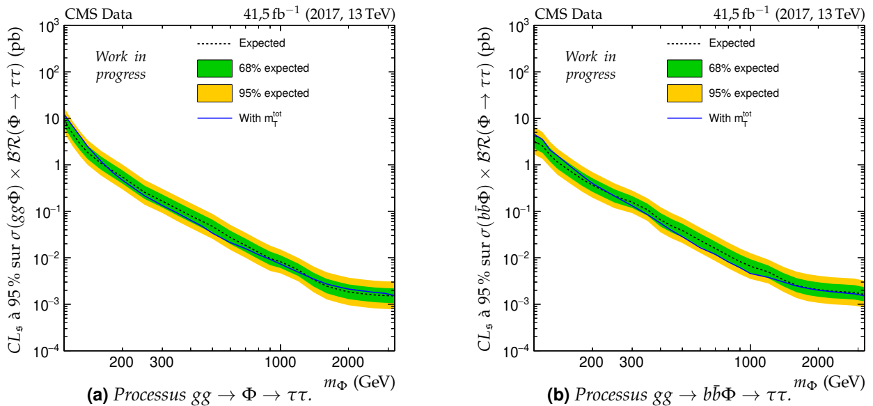
Figure 5.41 – Limites d'exclusion attendues avec m_{ML} en tant que variable discriminante (Expected) obtenues avec l'année 2017. Les limites obtenues avec m_T^{\text{tot}} sont également données (With m_T^{\text{tot}} ).
