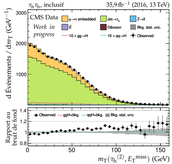
(b) Masse transverse du lepton 2 (τ h (2) ).
