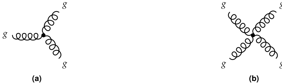
Figure 1.9 – Diagrammes de Feynman correspondant à l'interaction entre trois et quatre gluons.
