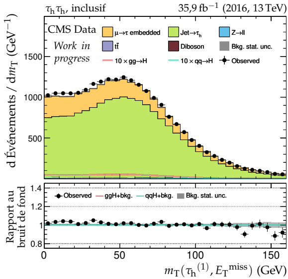
(a) Masse transverse du lepton 1 (τ h (1) ).
