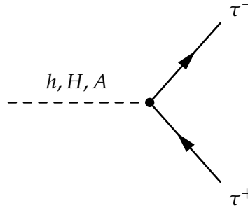
Figure 1.27 – Diagramme de Feynman d'une désintégration h, H, A \rightarrow \tau^+ \tau^- .
