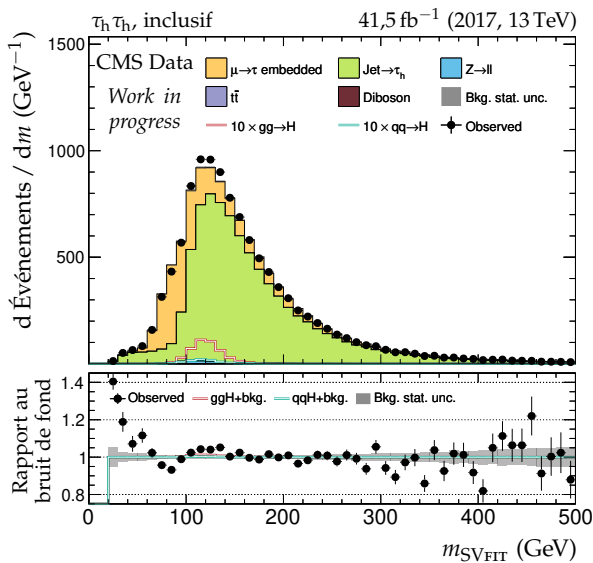
(e) Masse du système di- \tau d'après SVFIT.
