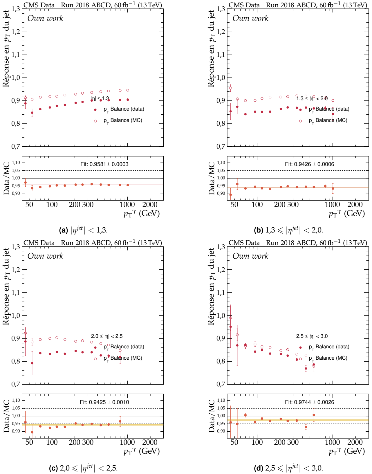
Figure 3.20 – Distributions des réponses équilibrées moyennes en fonction de p_T^\gamma pour différents intervalles de \eta^{jet} en 2018 avant extrapolation. Le rapport données réelles sur simulées est présenté dans chaque cas ainsi qu'un ajustement à une constante donnant l'ordre de grandeur de la correction résiduelle à appliquer.
