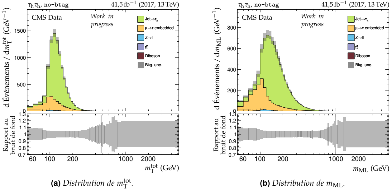
Figure 5.43 – Distributions de m_T^{\text{tot}} et m_{ML} en 2017 dans la catégorie no-btag du canal \tau_h\tau_h .
