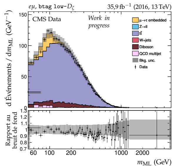
(f) Catégorie btag\ low-D_{\zeta_i} , m_{ML} .
