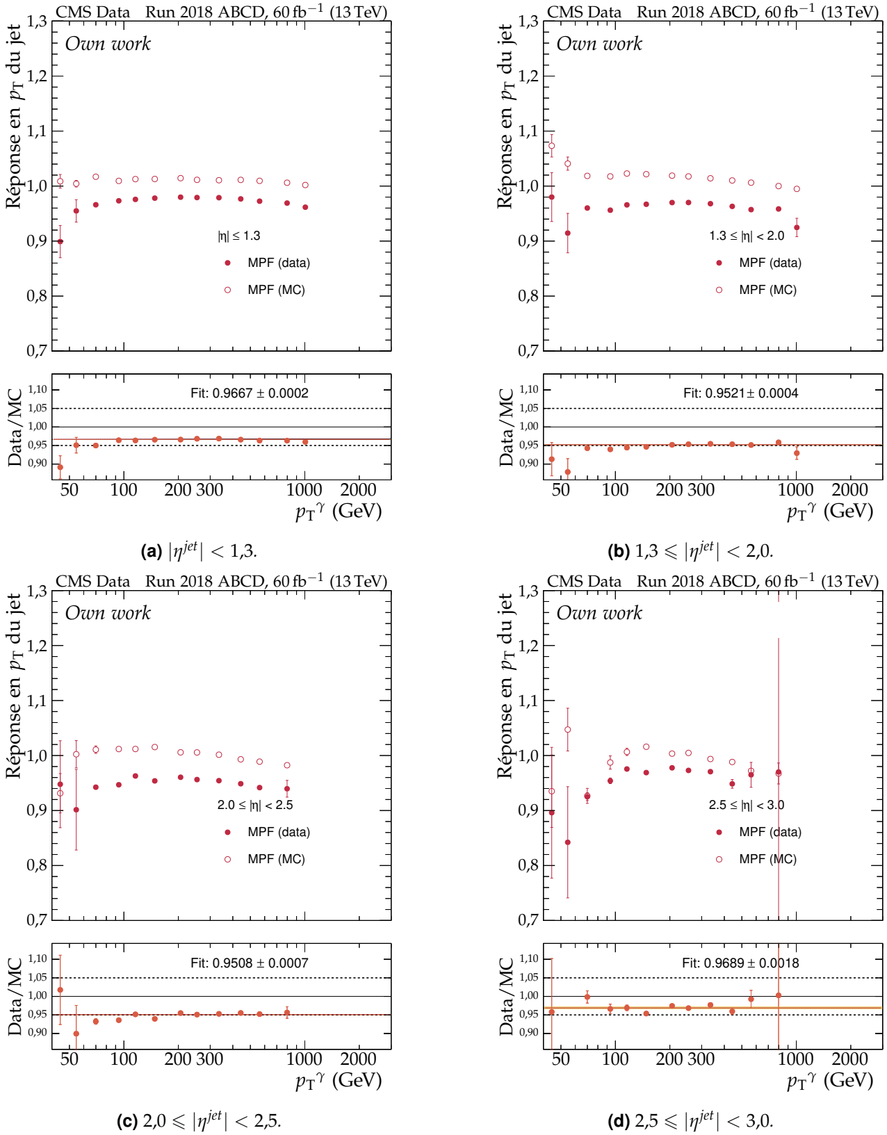
Figure 3.21 – Distributions des réponses MPF moyennes en fonction de p_T^\gamma pour différents intervalles de \eta^{jet} en 2018 avant extrapolation. Le rapport données réelles sur simulées est présenté dans chaque cas ainsi qu'un ajustement à une constante donnant l'ordre de grandeur de la correction résiduelle à appliquer.
