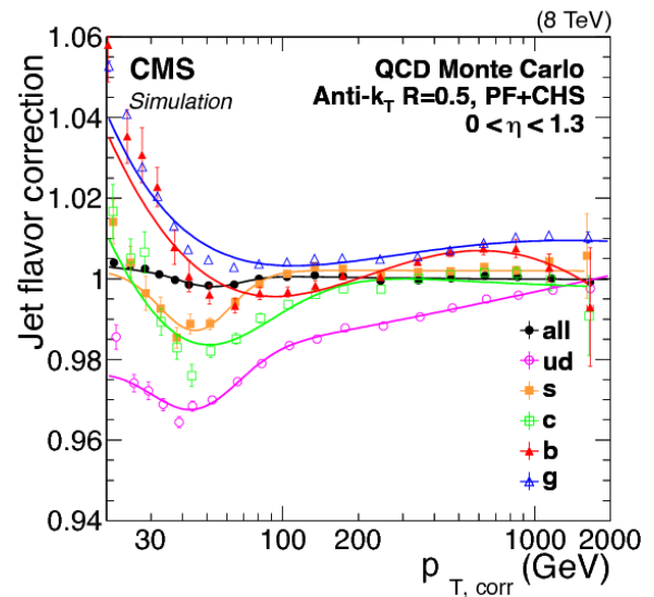
Figure 3.7 – Correction résiduelle de saveur en fonction de l'impulsion du jet à laquelle ont été appliquées les corrections décrites dans les sections précédentes, p_{T, \text{corr}} , pour des jets de pseudo-rapidité |\eta| < 1,3 [156].
