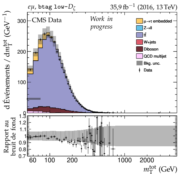
(e) Catégorie btag\ low-D_{\zeta_i} , m_T^{tot} .
