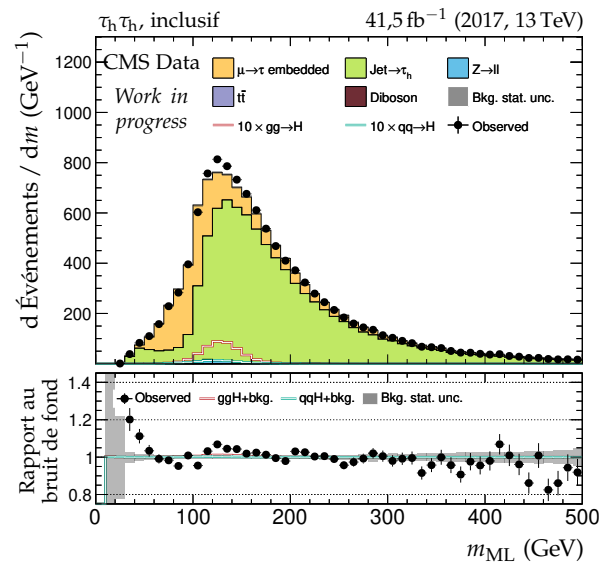
(f) Masse du système di- \tau d'après le ML.
