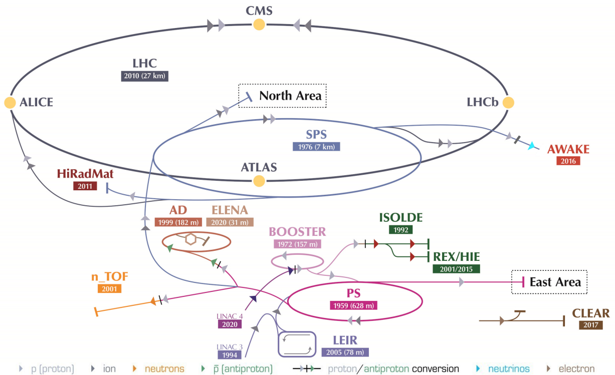
Figure 2.2 – Complexe des accélérateurs du CERN [93]. De nombreuses expériences y sont installées : AD, Décélérateur d’Antiprotons; AWAKE, Advanced WAKEfield Experiment; BOOSTER, Booster du Synchrotron à Protons; CLEAR, CERN Linear Electron Accelerator for Research; ELENA, Extra Low Energy Antiproton; HiRadMat, High-Radiation to Materials; ISOLDE, Isotope mass Separator On-Line; LEIR, Anneau d’Ions de Basse Énergie; LHC, Grand Collisionneur de Hadrons; LINAC 3, Accélérateur Linéaire 3; LINAC 4, Accélérateur Linéaire 4, remplace le LINAC 2; n_TOF, Neutrons Time Of Flight; PS, Synchrotron à Protons; REX/HIE, Radioactive EXperiment/High Intensity and Energy; SPS, Supersynchrotron à Protons; ALICE, A Large Ion Collider Experiment; ATLAS, A Toroidal LHC ApparatuS; CMS, Compact Muon Solenoid; LHCb, Large Hadron Collider beauty.
