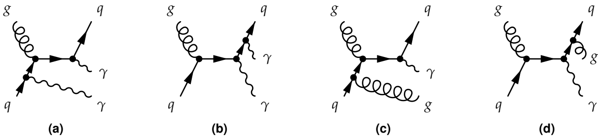
Figure 3.13 – Exemples de diagrammes de Feynman de processus correspondant à des événements avec deux photons (3.13a, 3.13b) ou deux jets (3.13c, 3.13d) dans l'état final, dus à l'ISR (3.13a, 3.13c) ou au FSR (3.13b, 3.13d).
