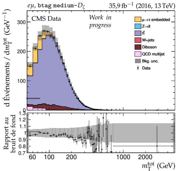
(c) Catégorie btag\ medium-D_{\zeta_i} , m_T^{tot} .
