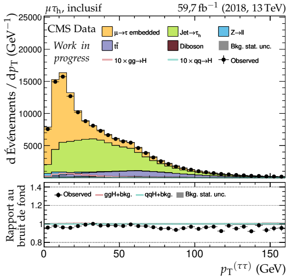
(c) Impulsion transverse du dilepton.
