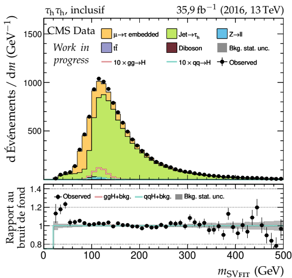
(e) Masse du système di-τ d'après SVFIT.
