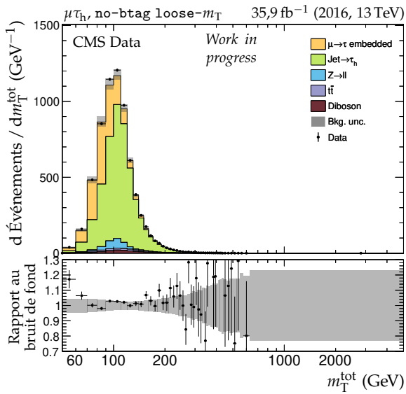
(c) Catégorie no-btag loose- m_{\text{T}} , m_{\text{T}}^{\text{tot}} .
