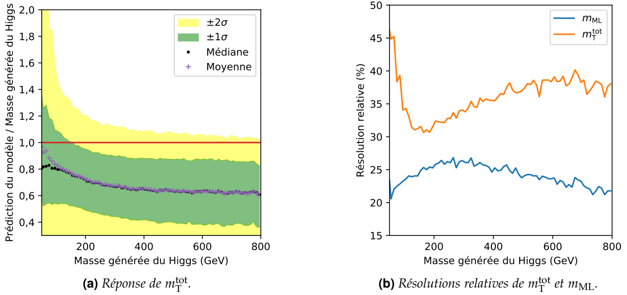
Figure 5.40 – Réponse de m_T^{\text{tot}} et comparaison de sa résolution relative à celle de m_{ML} .
