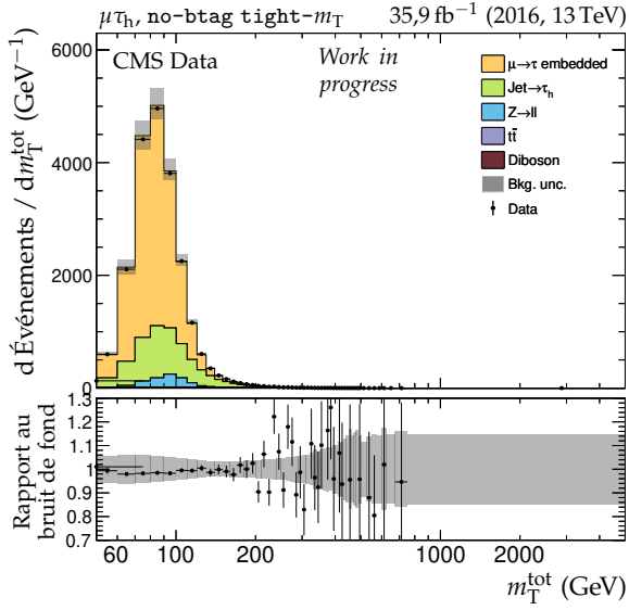
(a) Catégorie no-btag tight- m_{\text{T}} , m_{\text{T}}^{\text{tot}} .
