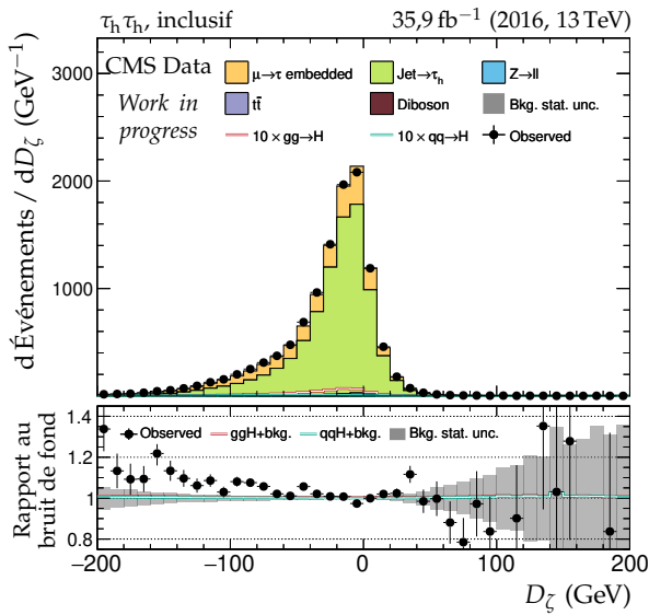
(c) Valeur de D ζ .
