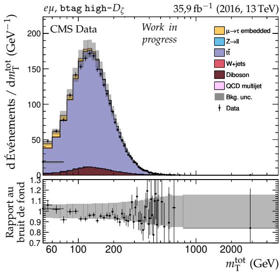
(a) Catégorie btag\ high-D_{\zeta_i} , m_T^{tot} .
