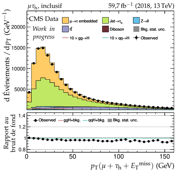
(e) Impulsion transverse du système di- \tau .
