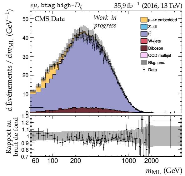
(b) Catégorie btag\ high-D_{\zeta_i} , m_{ML} .
