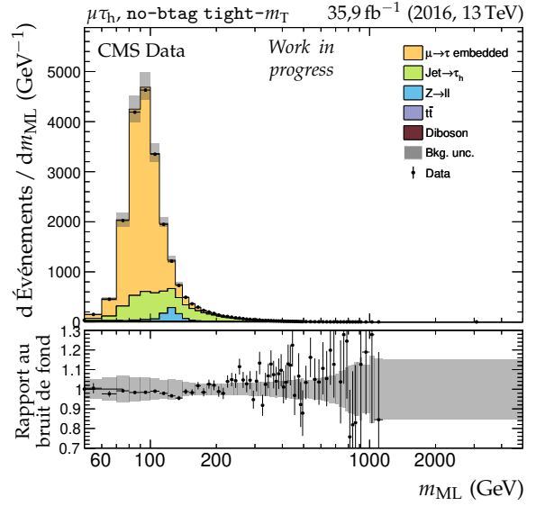
(b) Catégorie no-btag tight- m_{\text{T}} , m_{\text{ML}} .
