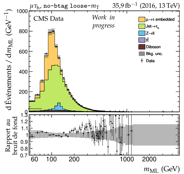
(d) Catégorie no-btag loose- m_{\text{T}} , m_{\text{ML}} .
