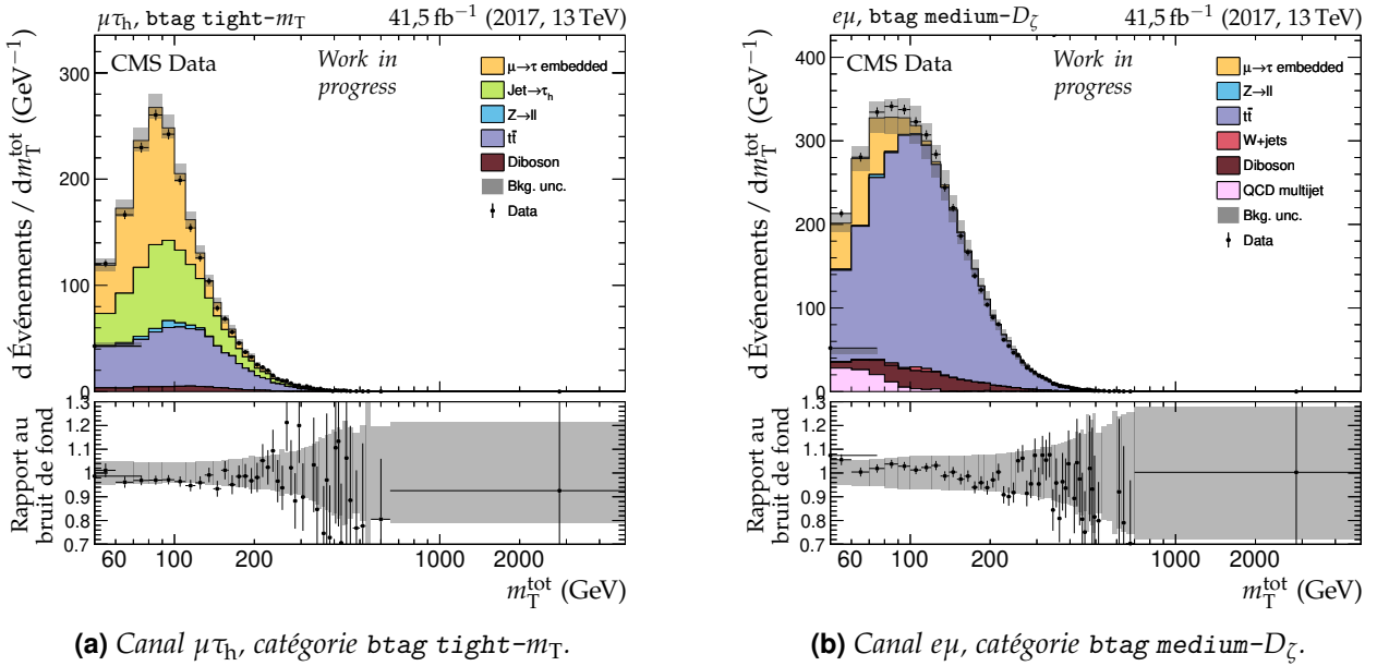
Figure 4.16 – Distributions de m_T^{\text{tot}} en 2017 pour deux catégories et canaux. Les données observées (points noirs) sont comparées à la modélisation des bruits de fond (histogrammes remplis en couleur et empilés). Les bandes grises correspondent à l'incertitude totale (statistique et systématique) sur le bruit de fond avant ajustement des paramètres de nuisance par COMBINE. Le rapport au bruit de fond est donné dans la partie inférieure des graphiques.
