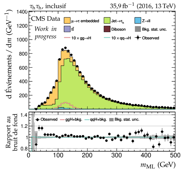
(f) Masse du système di-τ d'après le ML.
