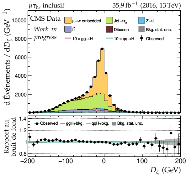
(c) Valeur de D_{\zeta_i} .
