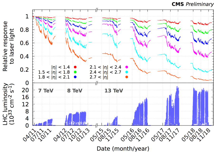
Figure 2.16 – Évolution temporelle de la réponse du ECAL [135] (haut) et luminosité instantanée du LHC (bas).
