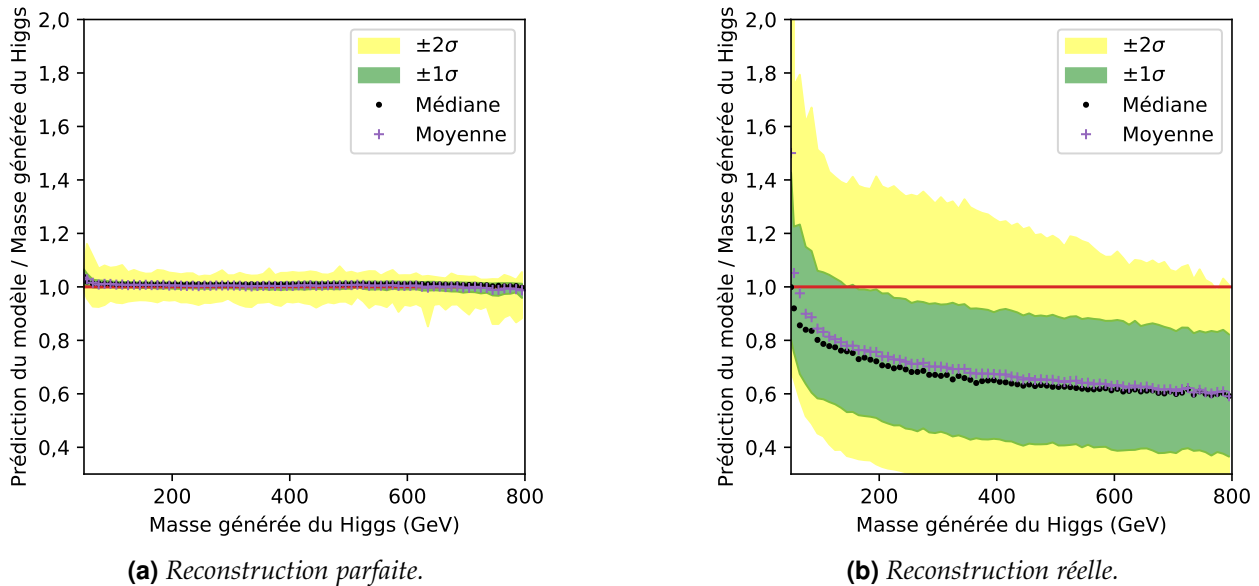
Figure 5.25 – Réponses du modèle B^{\text{gen}} dans le cas d'une reconstruction des particules parfaite et réelle.
