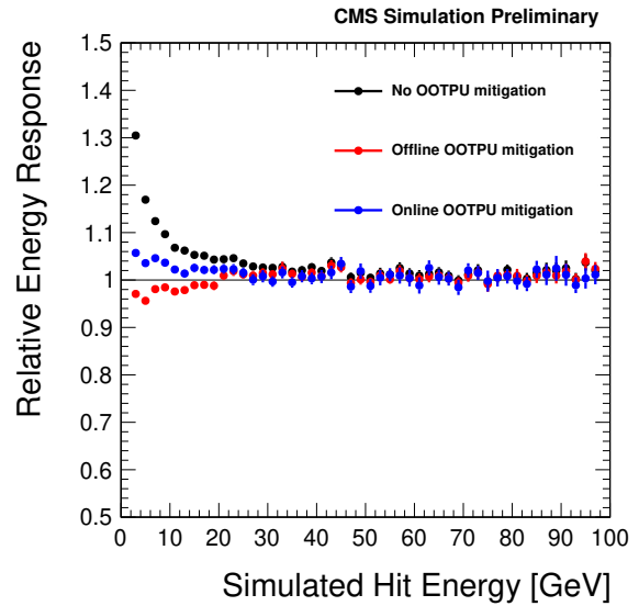
Figure 2.19 – Réponse relative du calorimètre hadronique de CMS [138] en fonction de l'énergie simulée du dépôt, estimée par simulation. En noir, sans correction de l'empilement asynchrone (OOTPU). En bleu, avec des corrections en ligne, c'est-à-dire un ajustement des amplitudes et temps d'arrivée des signaux en prenant en compte jusqu'à trois signaux avant et après le signal d'intérêt. En rouge, avec l'ensemble des corrections.
