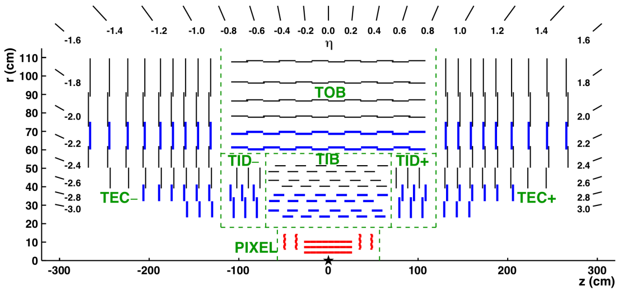
Figure 2.12 – Schéma détaillé du trajectographe du détecteur CMS dans le plan (Orz) [131, 132]. Le trajectographe est symétrique par rapport à l'axe (Oz) , axe du faisceau. Le centre du trajectographe, correspondant approximativement au lieu des collisions, est indiqué par une étoile. Les différentes sous-parties du trajectographe sont délimitées par les pointillés verts. Les modules à piste donnant des signaux en deux dimensions sont indiqués en lignes noires fines et ceux donnant des signaux en trois dimensions en lignes bleues épaisses. Ces derniers sont en fait constitués de deux modules à piste dos à dos dont l'un est tourné de 90^\circ . Les modules à pixels, en rouge, permettent également d'obtenir des signaux à trois dimensions. Les légers décalages des modules leur permettent d'éviter tout angle mort dans la zone d'acceptation du détecteur.
