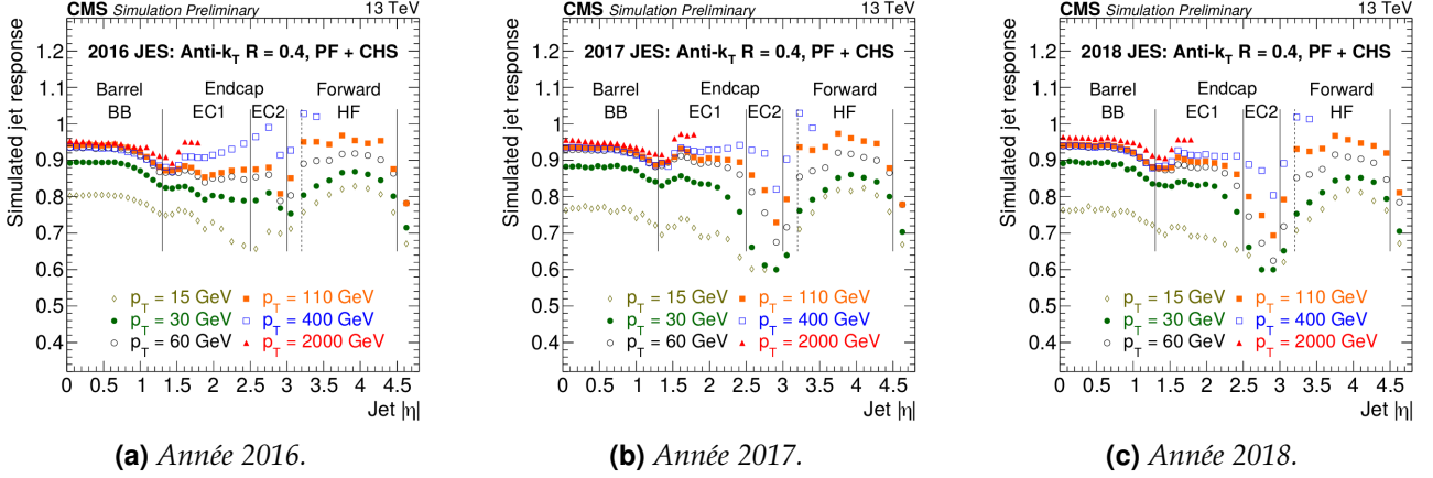
Figure 3.4 – Réponse des jets reconstruits en fonction de p_T et \eta lors du Run II [164]. La chute de la réponse des jets dans la région |\eta| \simeq 3 est due à la transition entre le bouchon et la partie vers l'avant du détecteur. Pour |\eta| > 4,5 , les limites d'acceptation du détecteur expliquent la chute de la réponse des jets. La dégradation au cours du temps du détecteur dans la région « EC2 » s'observe par la baisse de la réponse des jets dans cette région de 2016 à 2017.
