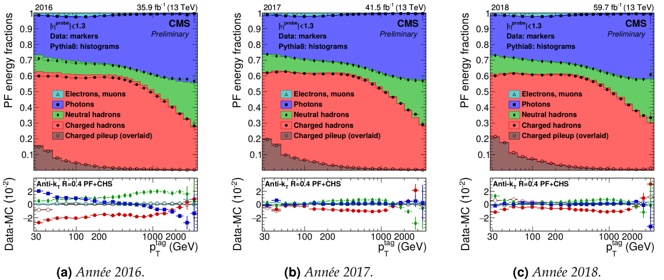
Figure 2.25 – Composition des jets reconstruits à l'aide de l'algorithme anti- k_T lors du Run II [164] en fonction de l'impulsion transverse du jet dans les données réelles (Data, histogrammes avec des points) et simulées (MC, histogrammes en couleurs). La partie Charged pileup (overlaid) en brun correspond à la fraction du jet retirée par la procédure CHS décrite dans le chapitre 3.
