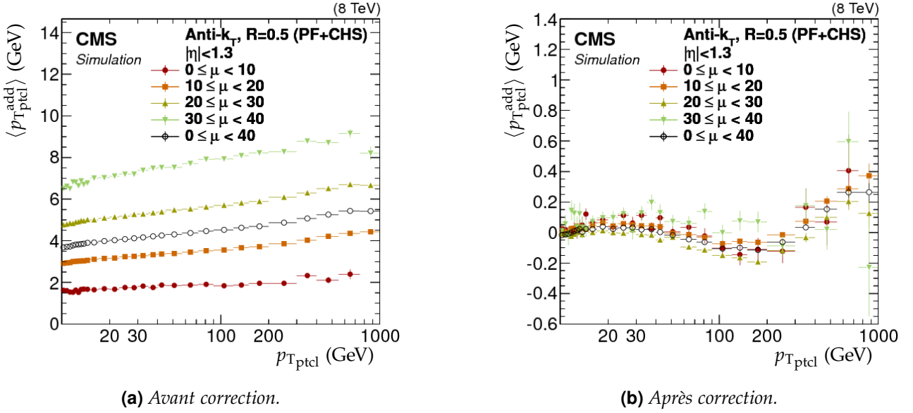
Figure 3.3 – Contribution additionnelle de l'empilement au niveau particule telle que définie dans l'équation (3.3) pour |\eta| < 1,3 en fonction de l'impulsion du jet au niveau particule pour différentes valeurs du nombre d'interaction d'empilement ( \mu ) [156].
