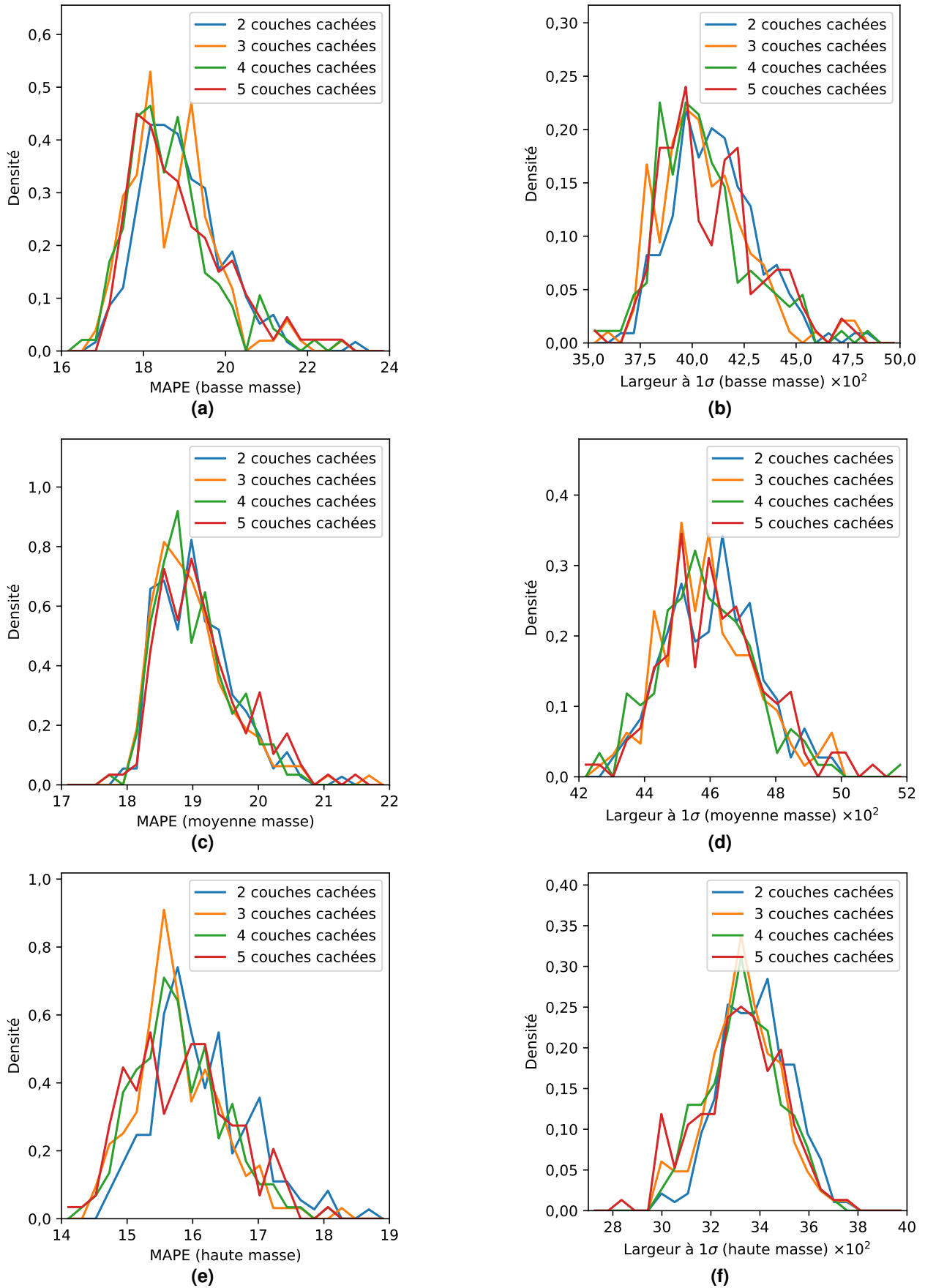
Figure 5.17 – Évaluations des DNNs regroupés selon N_{cc} par L_{MAPE} et \Delta_{1\sigma} .
