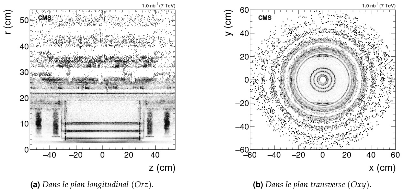
Figure 2.24 – Carte des points d'interaction entre particules des événements et matière composant le détecteur [132, 147] à partir de données prises en 2011 à \sqrt{s} = 7 TeV.
