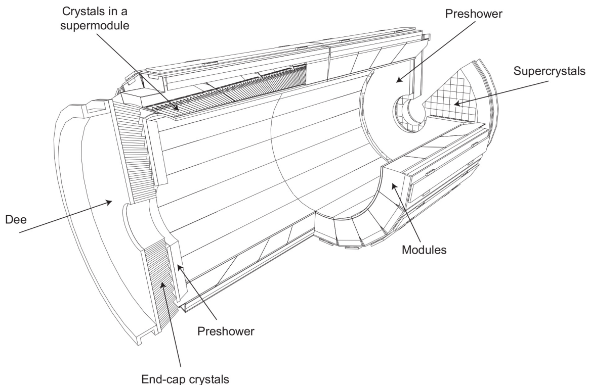
Figure 2.15 – Schéma du calorimètre électronique de CMS [114, 134] montrant le positionnement des cristaux, modules et supermodules dans le tonneau, des supercristaux et du détecteur de gerbes dans les bouchons.
