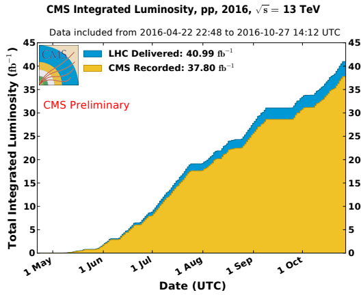
(a) Luminosité totale délivrée par le LHC et enregistrée par le détecteur CMS en fonction du temps en 2016.
