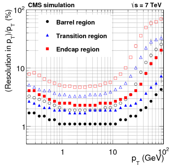
(b) Résolution pour des particules chargées.
