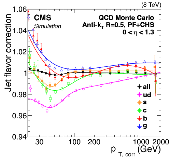
Figure 3.7 – Correction résiduelle de saveur en fonction de l'impulsion du jet à laquelle ont été appliquées les corrections décrites dans les sections précédentes, p_{T,corr} , pour des jets de pseudo-rapidité |\eta| < 1,3 [156].
