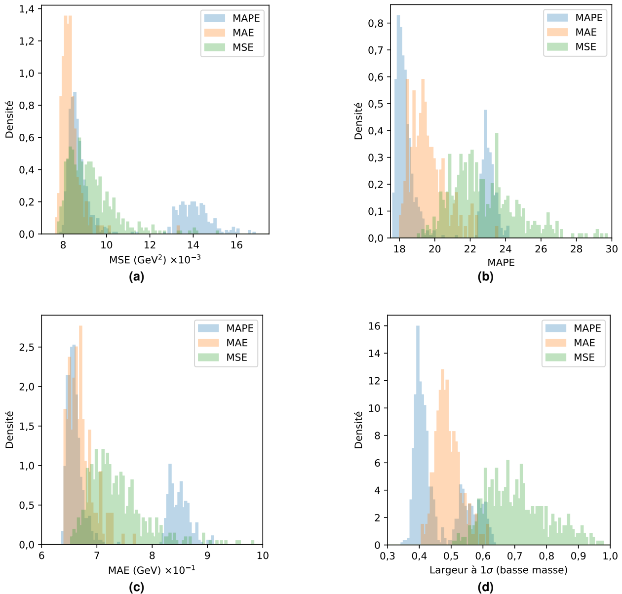
Figure 5.15 – Évaluations des DNNs regroupés selon la fonction de coût par L_{MSE} , L_{MAPE} , L_{MAE} et \Delta_{1\sigma} .
