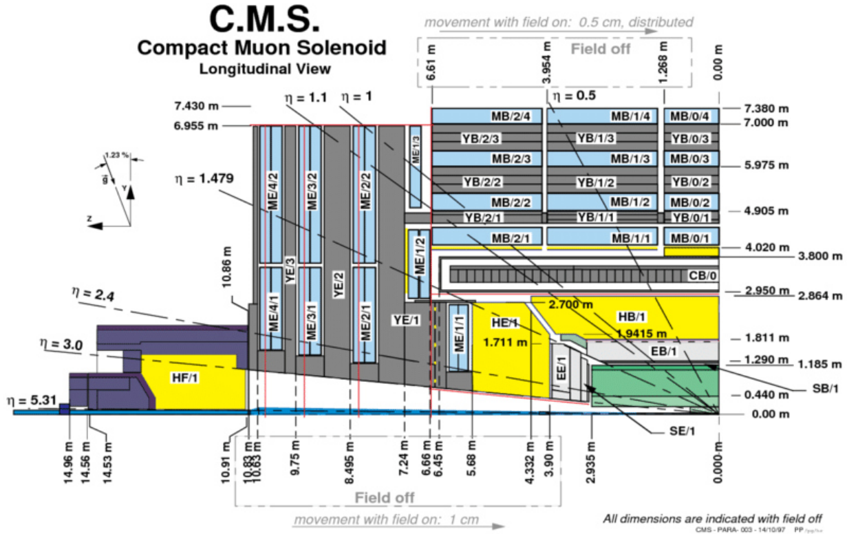
Figure 2.10 – Vue longitudinale d'un quadrant du détecteur CMS [126]. Les directions correspondant à quelques valeurs de pseudo-rapacité sont illustrées et des mesures de distances par rapport au centre du détecteur, lieu des collisions, sont indiquées. Le sol de la cavité présente une inclinaison de 1,23 % par rapport à la direction de la gravité locale \vec{g} , ce que montre le schéma à gauche.
