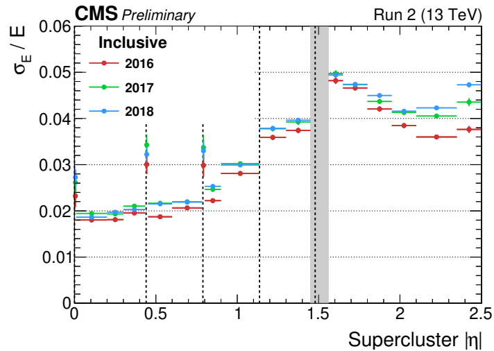
Figure 2.17 – Résolution relative de l'énergie des électrons dans le ECAL lors du Run II en fonction de \eta [136]. La résolution est obtenue à partir d'événements Z \rightarrow e^+e^- .
