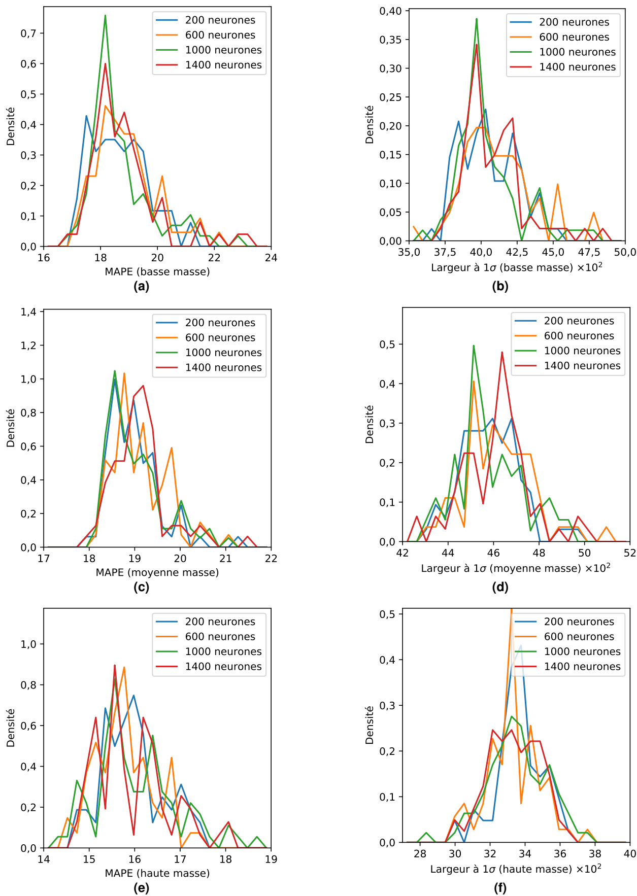
Figure 5.18 – Évaluations des DNNs regroupés selon N_{it} par L_{MAPE} et \Delta_{1\sigma} .
