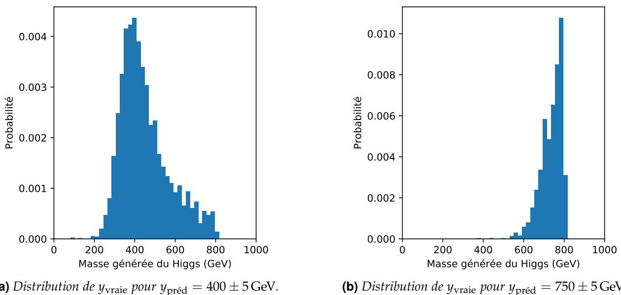
Figure 5.36 – Distributions de y_{\text{vraie}} à y_{\text{préd}} fixée.
