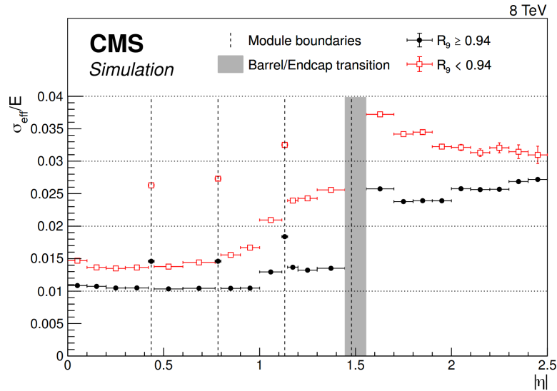
Figure 3.10 – Résolution relative en énergie des photons en fonction de \eta pour des événements simulés h \rightarrow \gamma\gamma [195]. La variable R_9 est définie au chapitre 2.
