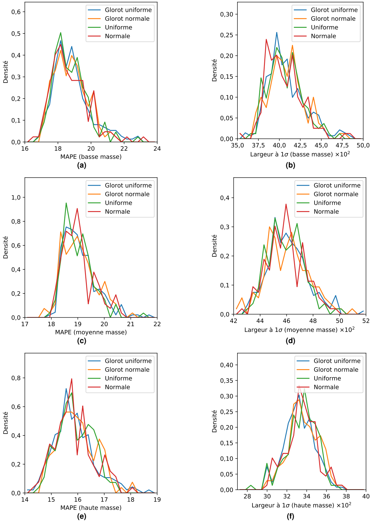
Figure 5.19 – Évaluations des DNNs regroupés selon le mode d'initialisation des poids par L_{MAPE} et \Delta_{1\sigma} .
