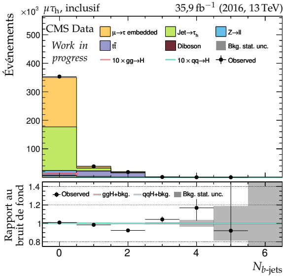
(a) Nombre de b -jets.
