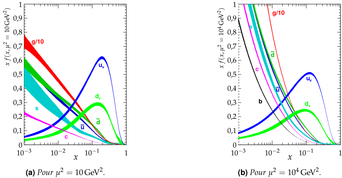
Figure 2.4 – Fonctions de distribution partoniques (PDF, Parton Distribution Functions) à différentes échelles d'énergie \mu obtenues au NNLO NNPDF3.0 [107] avec \alpha_s(m_Z^2) = 0,118 [9]. Les bandes tracées correspondent aux PDF f , avec incertitude, multipliées par la fraction d'impulsion x , où f peut être les quarks u et d de valence ( u_v, d_v ) ou les gluons ( g ), quarks et antiquarks de la mer ( \bar{u}, \bar{d}, s \simeq \bar{s}, c = \bar{c}, b = \bar{b} ).
