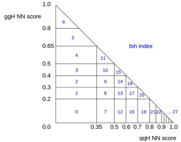
Figure 4.18 – Réduction à une dimension de la catégorie xxh [227].
