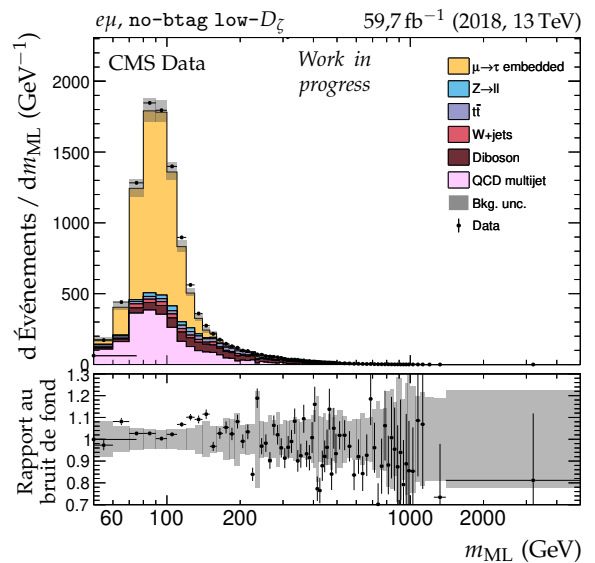
(f) Catégorie no-btag low- D_{\zeta_i} , m_{\text{ML}} .
