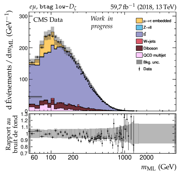
(f) Catégorie bttag low- D_{\zeta} , m_{\text{ML}} .
