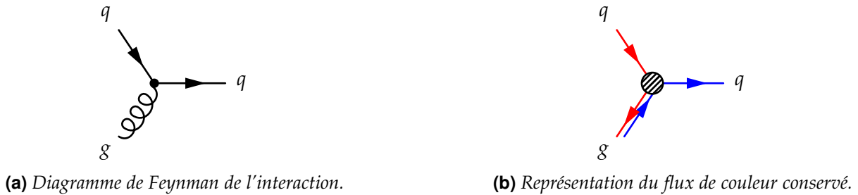
Figure 1.8 – Interaction entre un quark rouge et un gluon bleu-antirouge, donnant un quark bleu.
