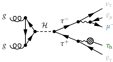
Figure 5.3 – Diagramme de Feynman des événements d'entraînement des modèles dans le cas du canal \mu\tau_h .
