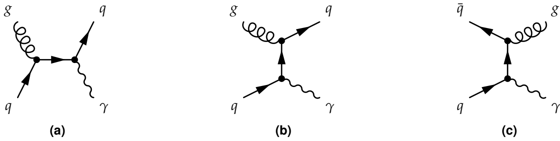
Figure 3.11 – Exemples de diagrammes de Feynman de processus physiques donnant un photon et un jet dans l'état final.
