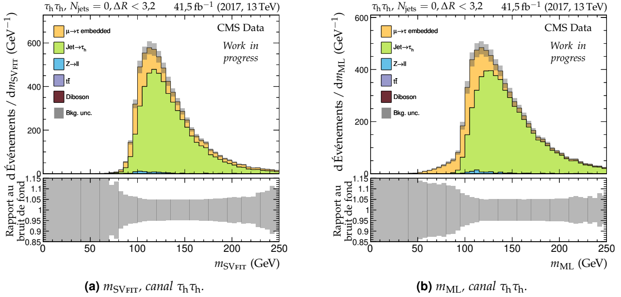
Figure 5.47 – Distributions de m_{\text{SVFIT}} et m_{\text{ML}} en 2017 dans le canal \tau_h \tau_h avec les événements sans jets et tels que la distance \Delta R entre les deux éléments du dilepton dans le plan (\eta, \phi) soit inférieure à 3,2.
