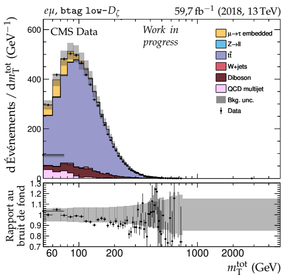
(e) Catégorie bttag low- D_{\zeta} , m_T^{\text{tot}} .
