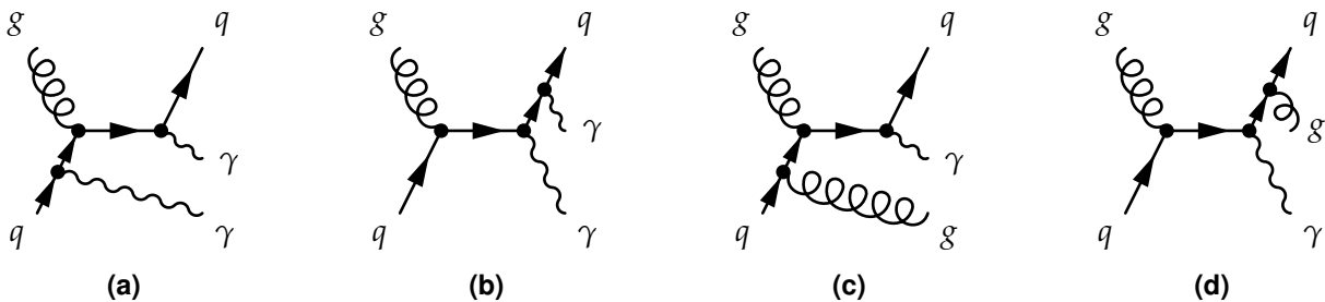
Figure 3.13 – Exemples de diagrammes de Feynman de processus correspondant à des événements avec deux photons (3.13a, 3.13b) ou deux jets (3.13c, 3.13d) dans l'état final, dus à l'ISR (3.13a, 3.13c) ou au FSR (3.13b, 3.13d).
