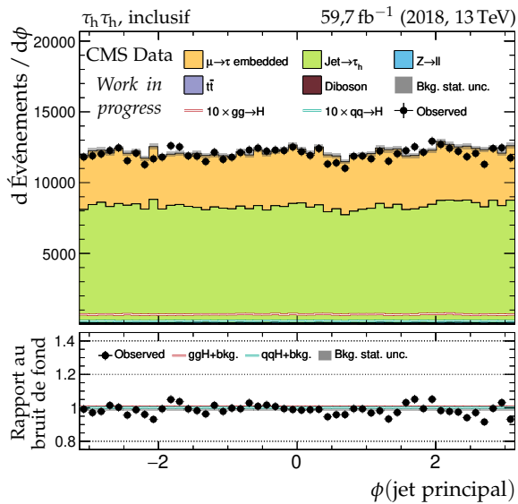
(e) Angle azimutal du jet principal.
