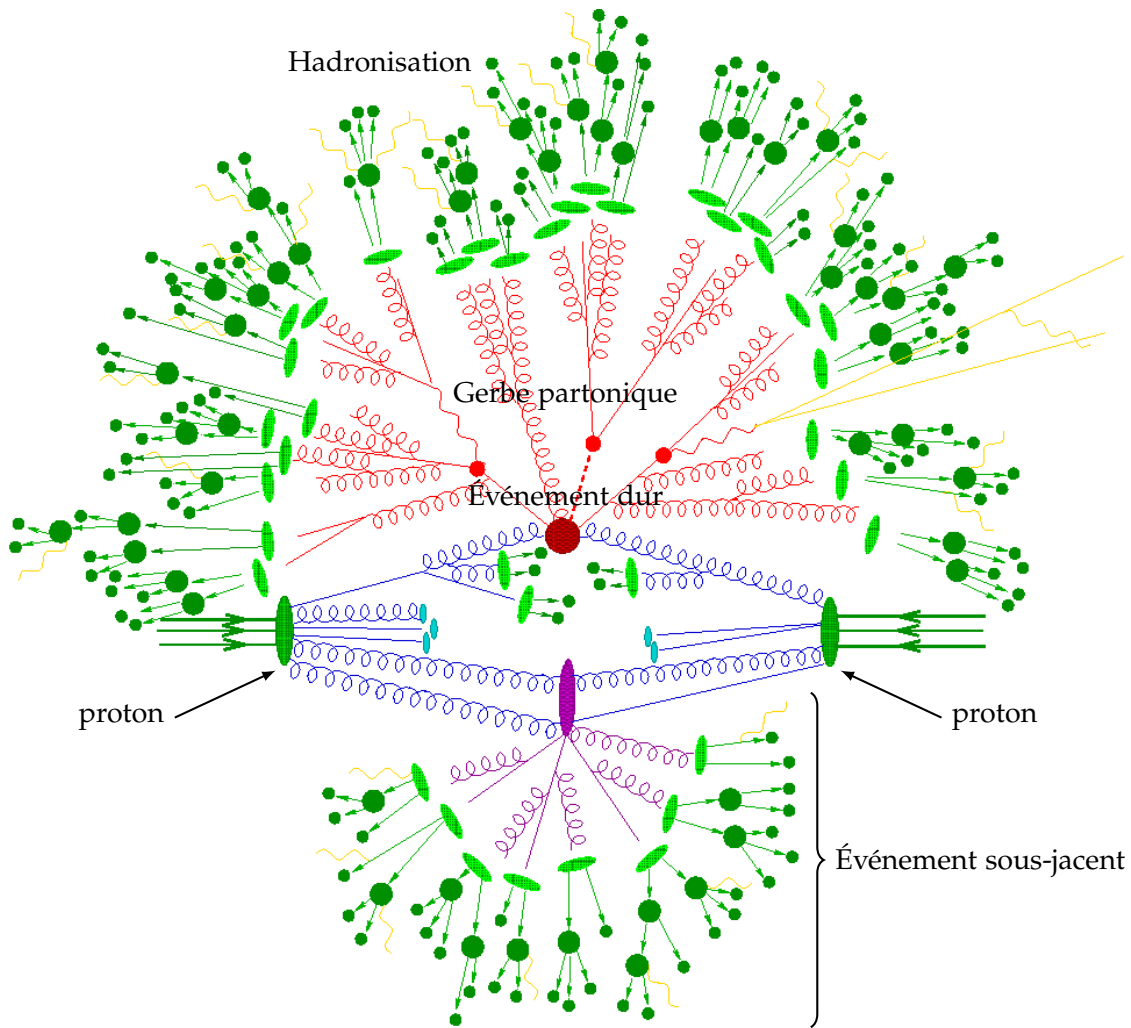
Figure 2.28 – Représentation d'une collision de protons [183]. Les interactions initiales entre les constituants des deux protons sont représentées en bleu. Celle de plus haute énergie est l'événement dur. Les particules en étant issues sont représentées en rouge. Le reste des interactions entre les constituants des protons est l'événement sous-jacent, dont sont issues les particules en violet. Les gerbes partoniques formées dans les événements dur et sous-jacent subissent la hadronisation dont sont issues les particules en vert observées dans le détecteur. Des radiations de photons, en jaune, peuvent survenir.
