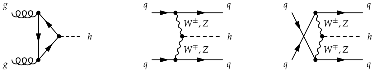
(a) Production par fusion de gluons (ggh).
