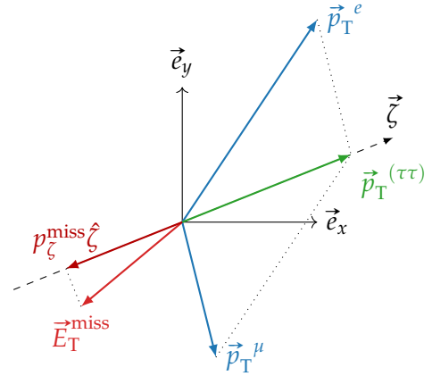
Figure 4.2 – Illustration de la définition de \hat{\zeta} [220]. Le plan de ce schéma est le plan transverse.
