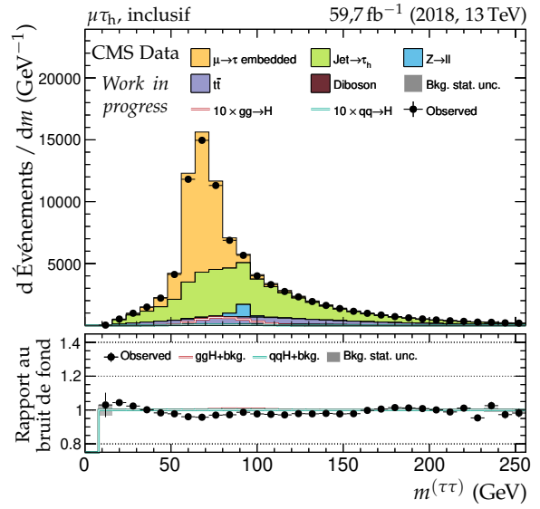
(d) Masse visible du dilepton.
