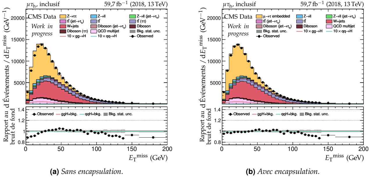
Figure 4.5 – Distributions de E_T^{\text{miss}} pour le canal \mu\tau_h en 2018. Les données observées (points noirs) sont comparées à la modélisation des bruits de fond (histogrammes remplis en couleur et empilés). Les bandes grisées correspondent à l’incertitude statistique totale sur le bruit de fond. Le rapport au bruit de fond est donné dans la partie inférieure des graphiques.
