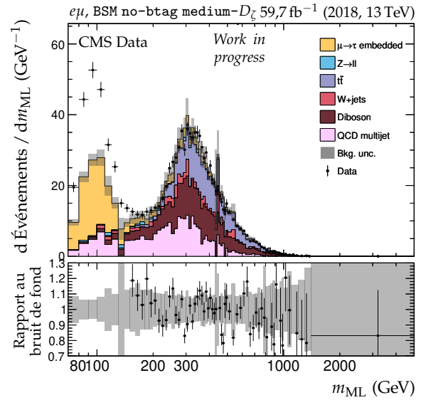
(d) Catégorie BSM no-btag medium- D_{\zeta} , m_{\text{ML}} .
