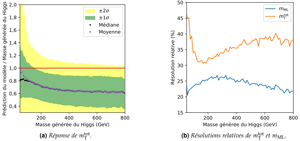
Figure 5.40 – Réponse de m_T^{tot} et comparaison de sa résolution relative à celle de m_{ML} .
