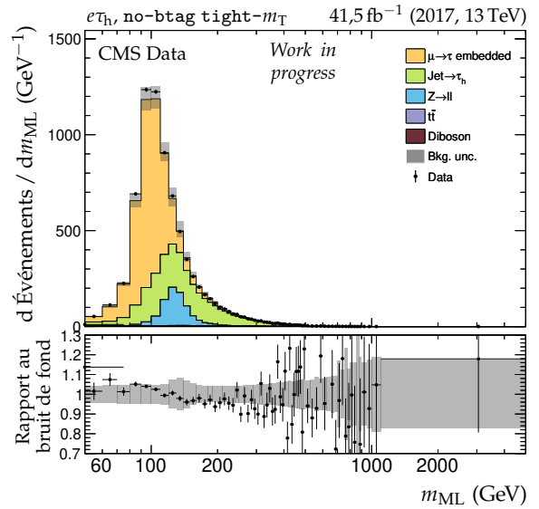
(b) Catégorie no-btag tight- m_T , m_{\text{ML}} .
