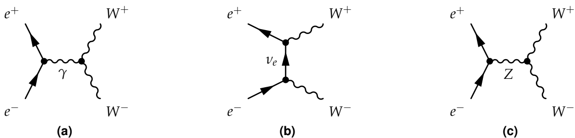
Figure 1.4 – Diagrammes de Feynman de production de paire W^+W^- à l'arbre.
