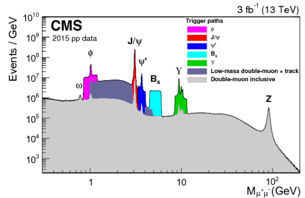
Figure 2.21 – Distribution de la masse invariante des dimuons obtenus à partir du système de déclenchement des chambres à muons [142]. Les données ont été récoltées en 2015 à l'aide d'un déclenchement global (gris) ainsi que plusieurs déclenchements spécifiques (en couleur). Les résonances de diverses particules apparaissent distinctement.
