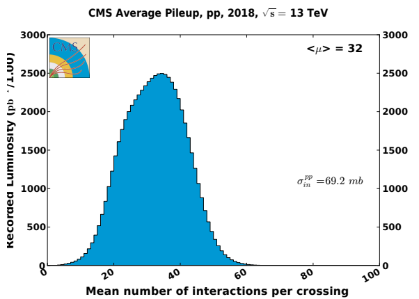
(b) Distribution du nombre moyen d'interactions par croisement de faisceaux en 2018.
