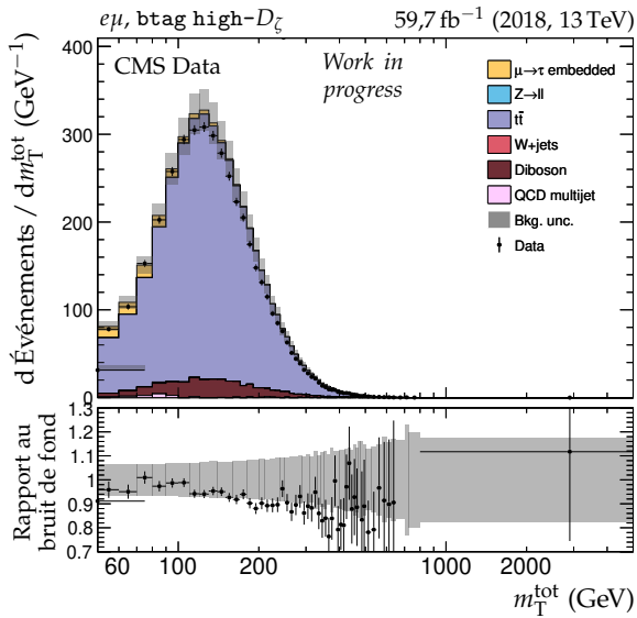
(a) Catégorie bttag high- D_{\zeta} , m_T^{\text{tot}} .
