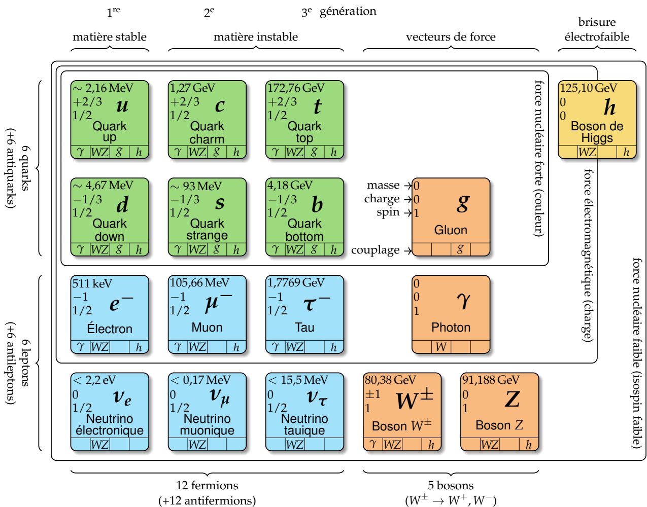
Figure 1.1 – Particules élémentaires du modèle standard. Les quarks (en vert) et les leptons (en bleu) sont des fermions. Les bosons vecteurs (en orange) sont les médiateurs des forces fondamentales. Le boson de Higgs est quant à lui un boson scalaire (en jaune).
