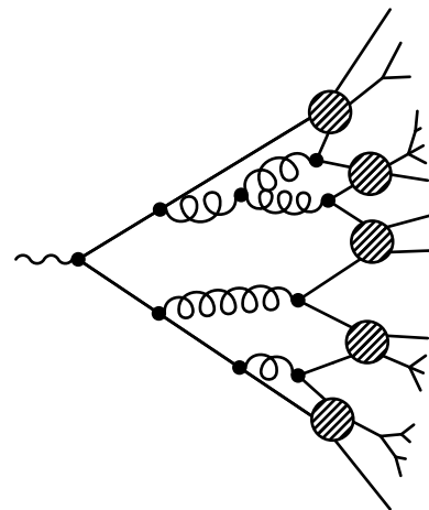
Figure 1.14 – Schématisation de l’hadronisation dans le cadre du modèle d’agglomération hadronique.
