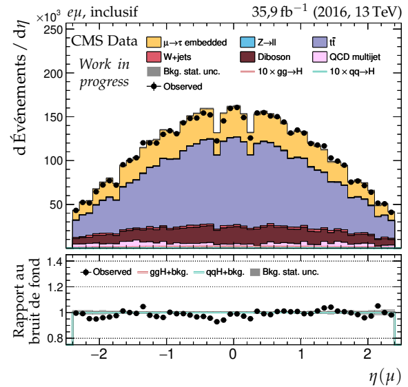
(d) Pseudo-rapidité du lepton 2 ( \mu ).
