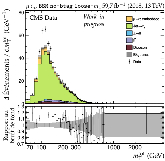
(c) Catégorie BSM no-btag loose- m_{\text{T}} , m_{\text{T}}^{\text{tot}} .
