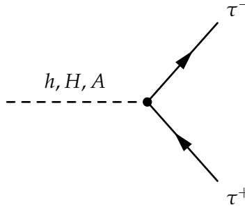
Figure 1.27 – Diagramme de Feynman d'une désintégration h, H, A \rightarrow \tau^+ \tau^- .
