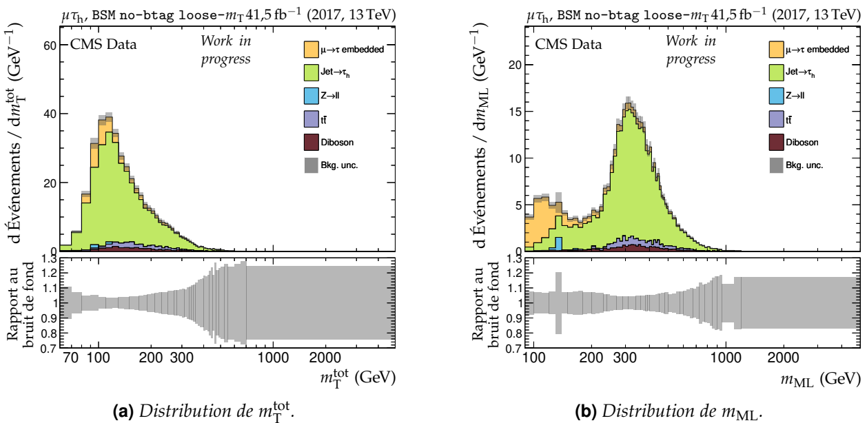
Figure 5.44 – Distributions de m_T^{\text{tot}} et m_{ML} en 2017 dans la catégorie BSM no-btag loose- m_T du canal \mu\tau_h .
