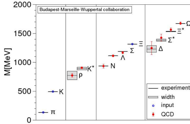
Figure 1.11 – Spectre de masse des hadrons légers [43]. Les lignes horizontales ainsi que les zones grisées sont les valeurs expérimentales et les largeurs de désintégration. Les résultats obtenus en utilisant des calculs de QCD sur réseau sont représentés par des cercles, avec les erreurs associées. Seules les masses des hadrons \pi , K et \Xi ne présentent pas de barres d'erreurs, celles-ci sont utilisées pour fixer les paramètres libres du modèle.
