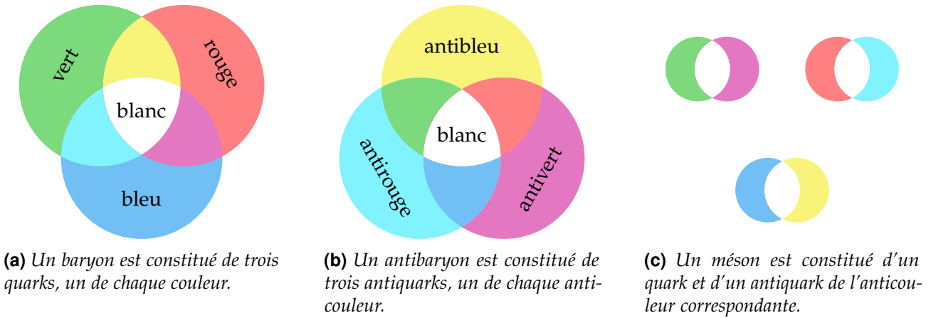
Figure 1.7 – Combinaisons des couleurs des quarks dans les hadrons. La couleur globale est toujours blanche, c'est-à-dire que la charge de couleur globale est nulle.
