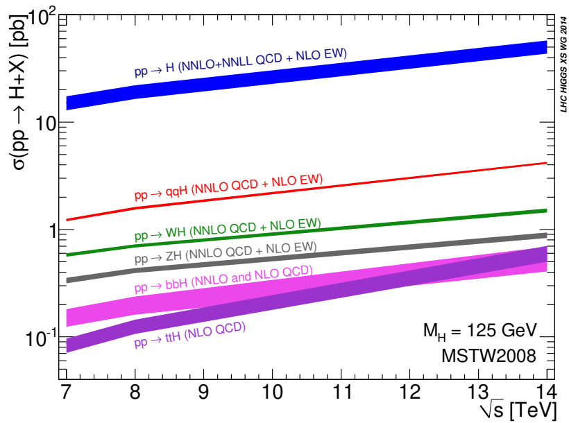
Figure 1.19 – Sections efficaces des modes de production du boson de Higgs du modèle standard [83-86].
