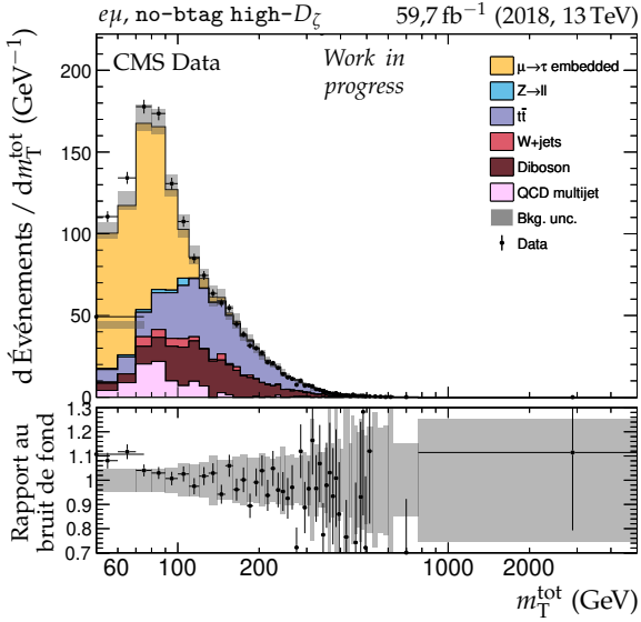
(a) Catégorie no-btag high- D_{\zeta_i} , m_T^{\text{tot}} .
