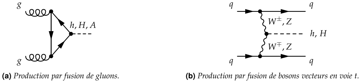
Figure 1.23 – Diagrammes de Feynman de production de boson de Higgs dans le cadre du MSSM par fusion de gluons ( ggH ) et fusion de bosons vecteurs (VBF).
