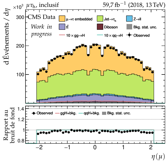
(c) Pseudo-rapidité du lepton 1 ( \mu ).
