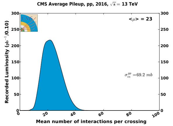
(b) Distribution du nombre moyen d'interactions par croisement de faisceaux en 2016.
