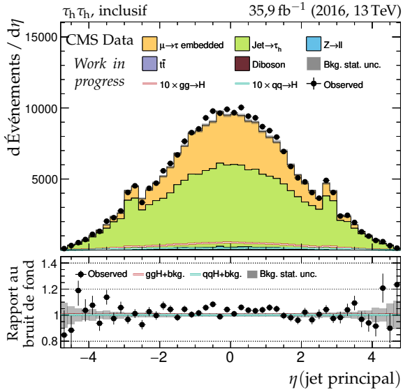
(c) Pseudo-rapacité du jet principal.
