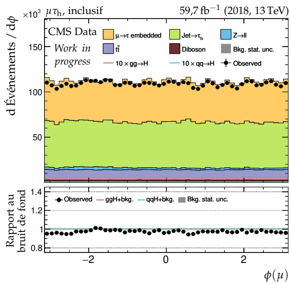
(e) Angle azimutal du lepton 1 ( \mu ).
