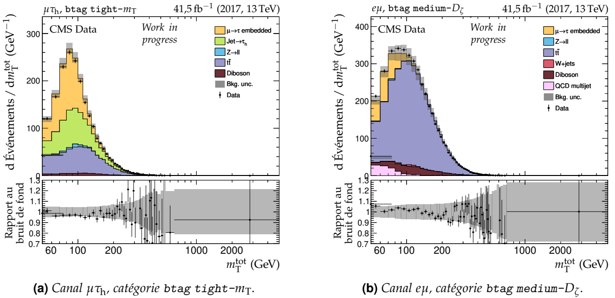
Figure 4.16 – Distributions de m_T^{\text{tot}} en 2017 pour deux catégories et canaux. Les données observées (points noirs) sont comparées à la modélisation des bruits de fond (histogrammes remplis en couleur et empilés). Les bandes grises correspondent à l'incertitude totale (statistique et systématique) sur le bruit de fond avant ajustement des paramètres de nuisance par COMBINE. Le rapport au bruit de fond est donné dans la partie inférieure des graphiques.
