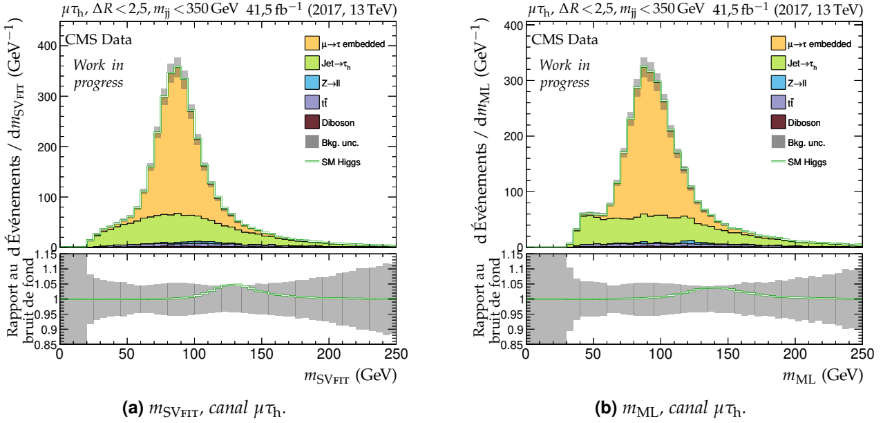
Figure 5.49 – Distributions de m_{\text{SVFIT}} et m_{\text{ML}} en 2017 dans le canal \mu\tau_h avec les événements contenant au moins deux jets avec la masse invariante des deux jets principaux m_{jj} inférieure à 350 GeV et tels que la distance \Delta R entre les deux éléments du dilepton dans le plan (\eta, \phi) soit inférieure à 2,5.
