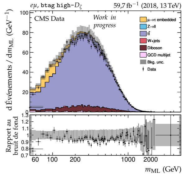
(b) Catégorie bttag high- D_{\zeta} , m_{\text{ML}} .
