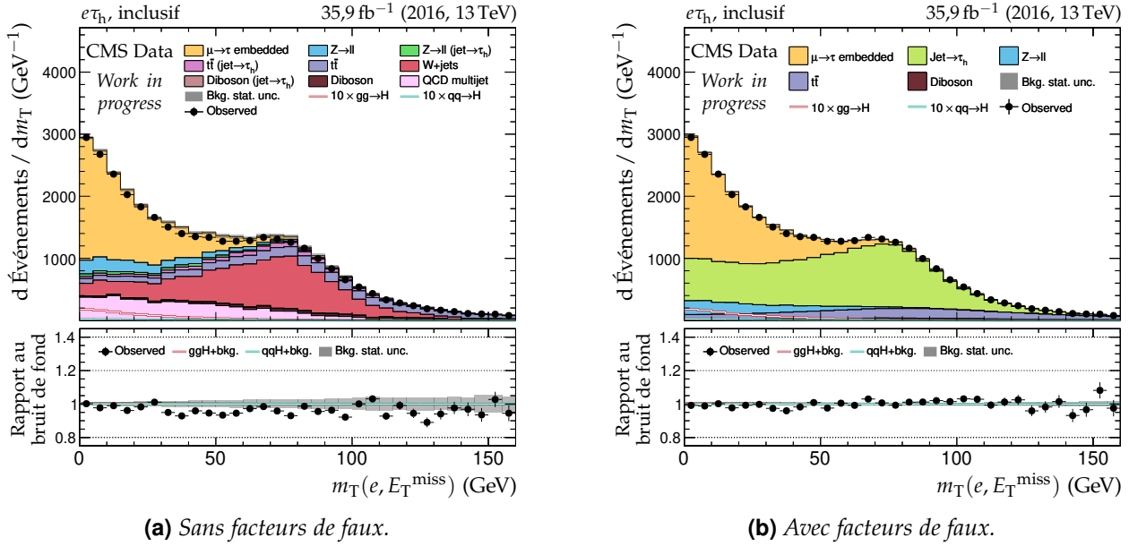
Figure 4.12 – Distributions de la masse transverse de l'électron pour le canal e\tau_h en 2016.
