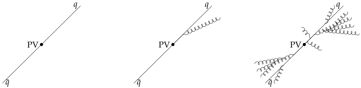
(a) Deux quarks sont initialement produits, ce qui correspond au diagramme de la figure 1.12a.
