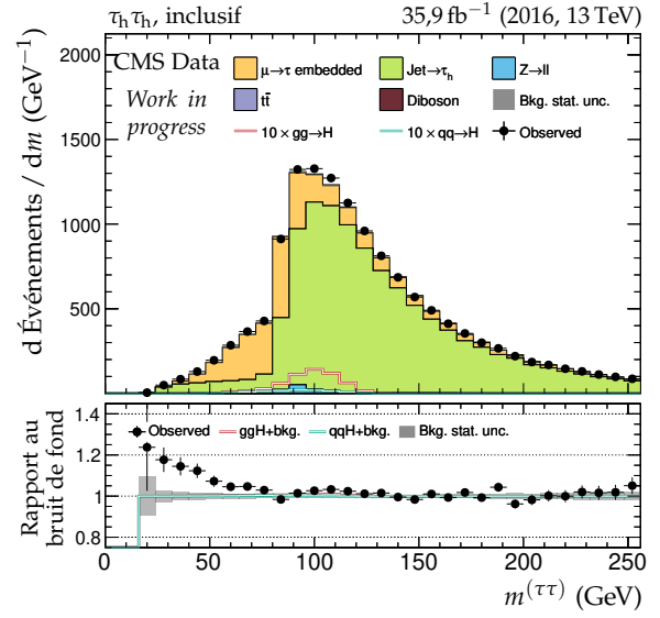
(d) Masse visible du dilepton.
