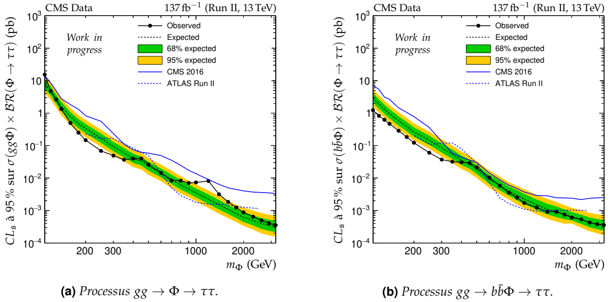
Figure 4.21 – Limites d’exclusion indépendantes du modèle physique obtenues avec l’intégralité des données du Run II récoltées par CMS. Les précédents résultats [81] obtenus avec les données de l’année 2016 sont également donnés (CMS 2016) ainsi que ceux de la collaboration ATLAS sur l’intégralité du Run II [208] (ATLAS Run II).
