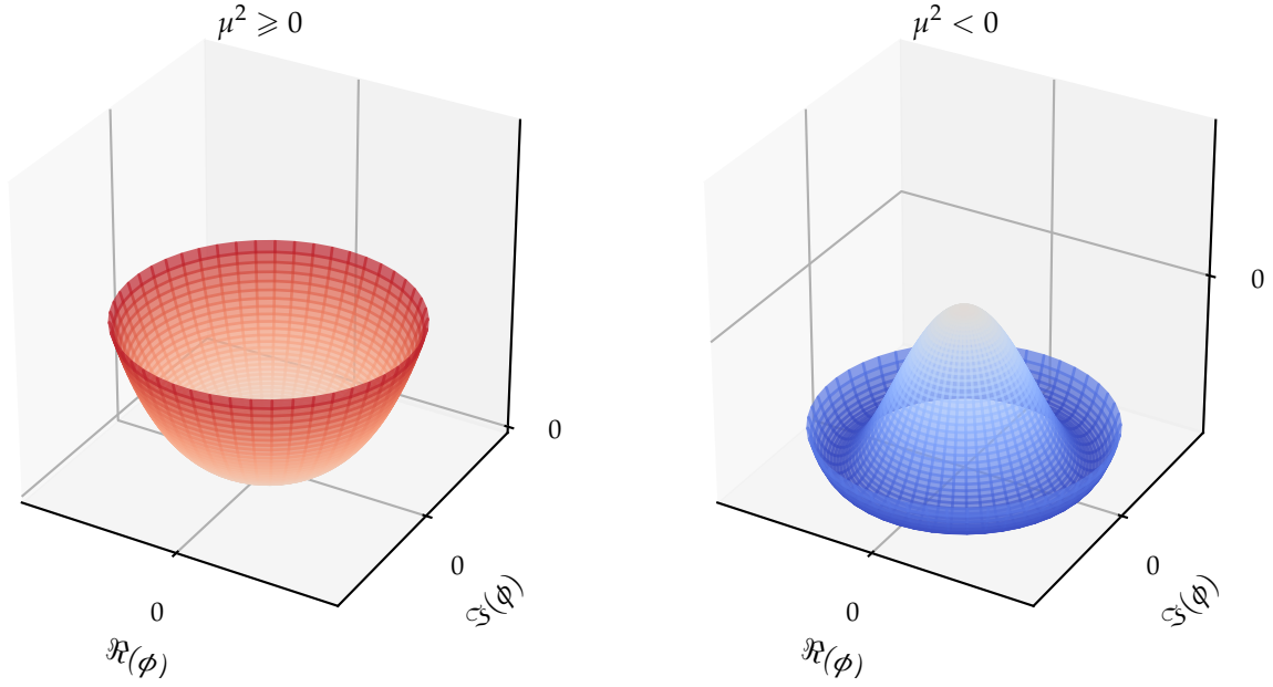
Figure 1.6 – Forme du potentiel du Higgs V selon le signe de \mu^2 .
