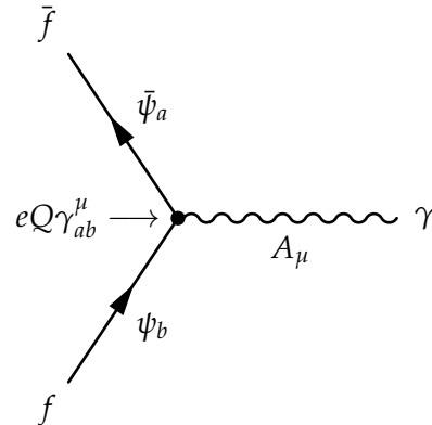
Figure C.4 – Diagramme de Feynman issu du terme du lagrangien du modèle standard de l’équation (C.1). Un fermion f et un antifermion \bar{f} sont présents dans l’état initial et sont décrits par un champ fermionique \psi et son adjoint \bar{\psi} . Le champ \psi interagit par ses composantes a et b avec le champ vectoriel A_\mu au vertex, avec un couplage donné par eQ\gamma_{ab}^\mu . Il en résulte un photon \gamma , décrit par ce champ A_\mu .
