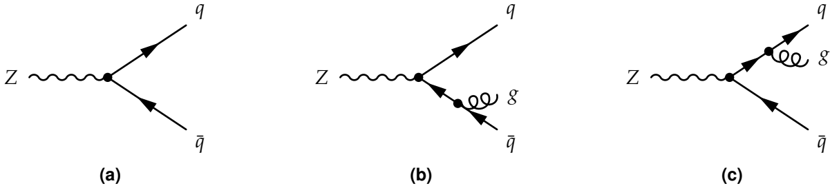
Figure 1.12 – Un boson Z se désintègre en paire quark-antiquark. Dans les cas des figures 1.12b et 1.12c, un gluon supplémentaire est émis.
