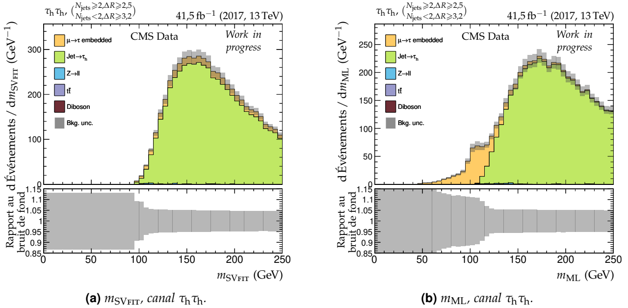
Figure 5.48 – Distributions de m_{\text{SVFIT}} et m_{\text{ML}} en 2017 dans le canal \tau_h \tau_h avec les événements contenant moins de deux jets et tels que la distance \Delta R entre les deux éléments du dilepton dans le plan (\eta, \phi) soit supérieure à 3,2 ou contenant au moins deux jets et \Delta R \geq 2,5 .
