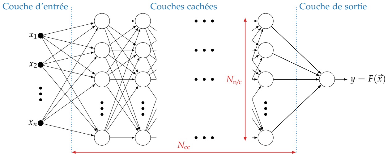
Figure 5.8 – Structure normale profonde à propagation avant complètement connectée d'un réseau de neurones. Une couche d'entrée comporte autant de neurones que de variables x_i . La couche de sortie en comporte autant que de valeurs à donner, c'est-à-dire une. Les fonctions d'activation de ces deux couches sont linéaires. Entre elles se trouvent N_{cc} couches cachées, chacune contenant N_{n/c} neurones. Diverses fonctions d'activation peuvent être utilisées dans les couches cachées.
