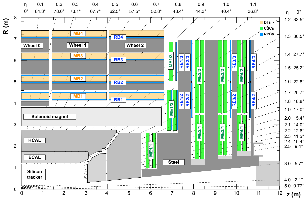
Figure 2.20 – Schéma d'un quadrant du détecteur CMS [142] montrant la localisation des chambres à muons et leur nature : tubes à dérivation (DT, en jaune), chambres à pistes cathodiques (CSC, en vert) et chambres à plaques résistives (RPC, en bleu). Certaines valeurs de \eta et les directions associées sont indiquées.
