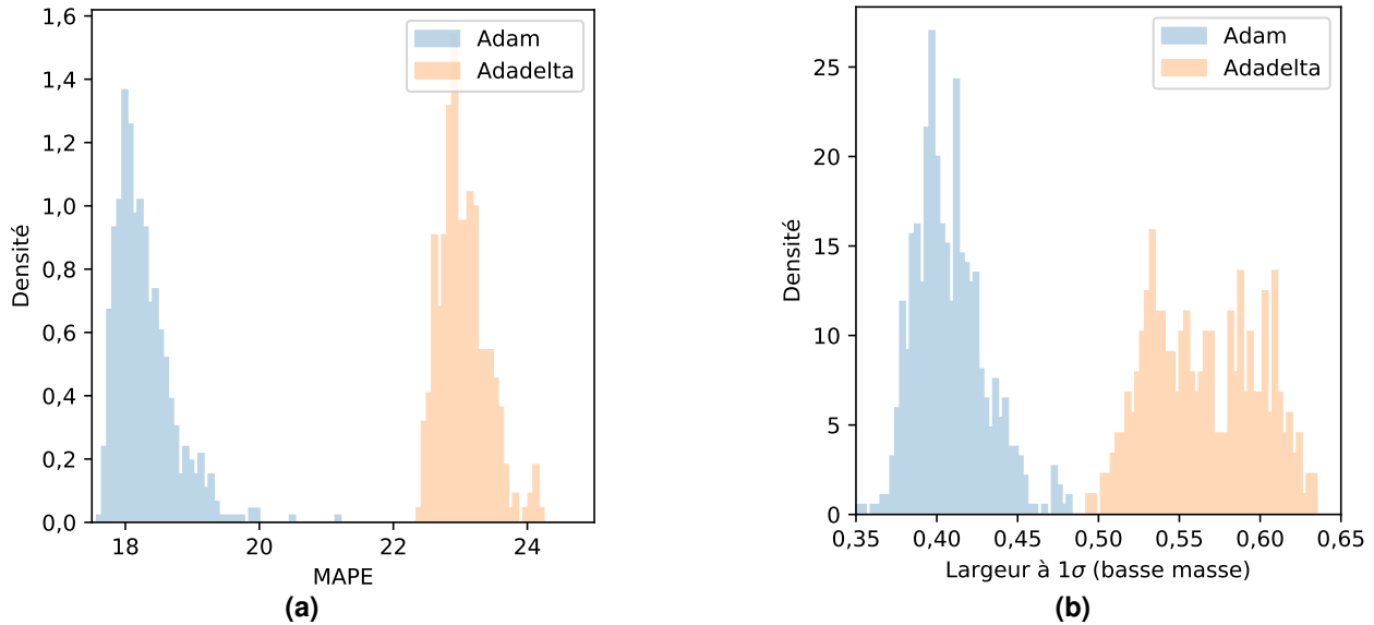
Figure 5.16 – Évaluations des DNNs regroupés selon l'algorithme d'optimisation par L_{\text{MAPE}} et \Delta_{1\sigma} .
