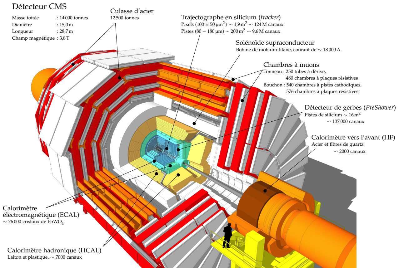
Figure 2.8 – Vue ouverte du détecteur CMS [120].
