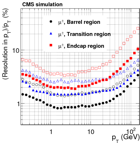
(a) Résolution pour des muons seuls et isolés.
