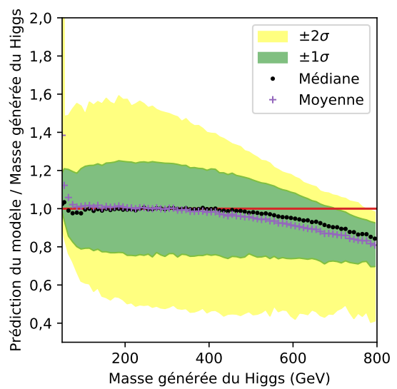
(f) Réponse du modèle G.
