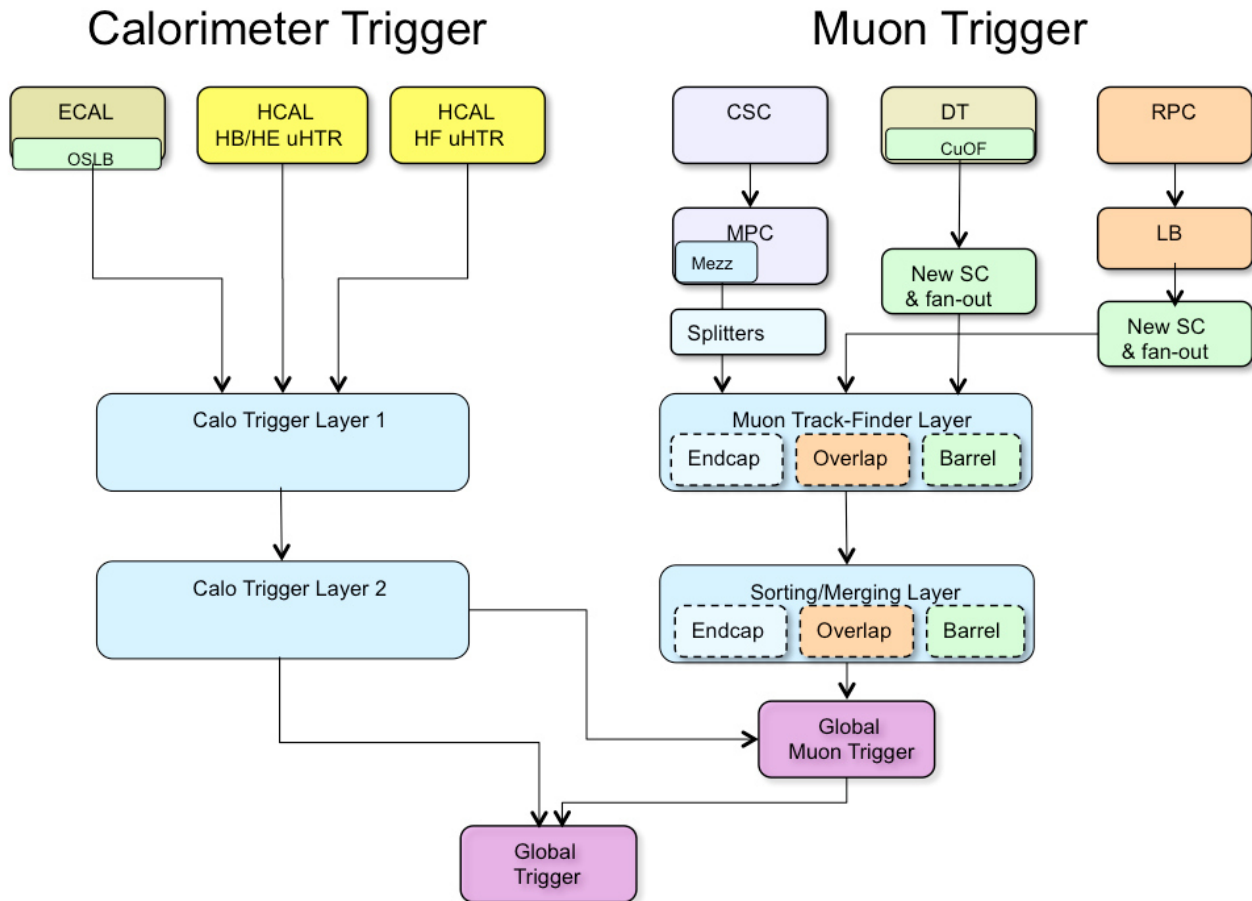
Figure 2.22 – Architecture du système de déclenchement L1 [146].
