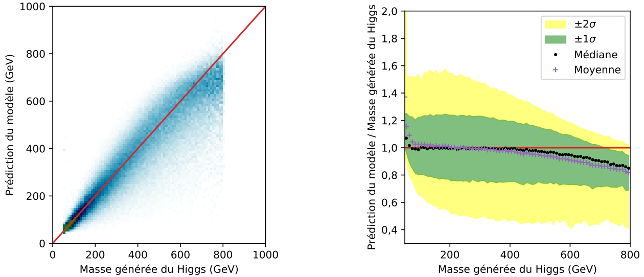
(a) Histogramme à deux dimensions de y_{\text{préd}} en fonction de y_{\text{vraie}} .
