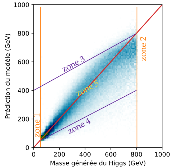
Figure 5.38 – Zones considérées pour l'entraînement.
