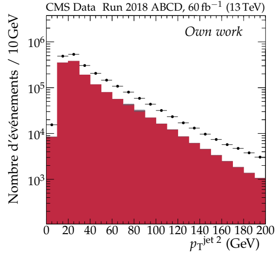
(d) Impulsion transverse du second jet.
