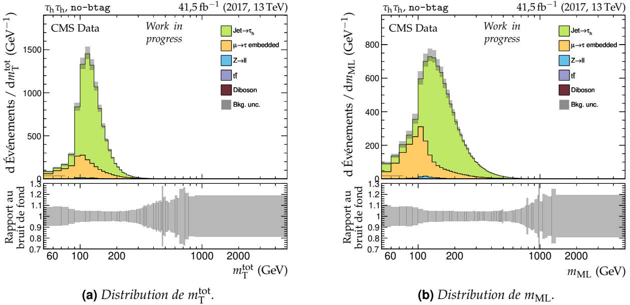
Figure 5.43 – Distributions de m_T^{\text{tot}} et m_{ML} en 2017 dans la catégorie no-btag du canal \tau_h\tau_h .
