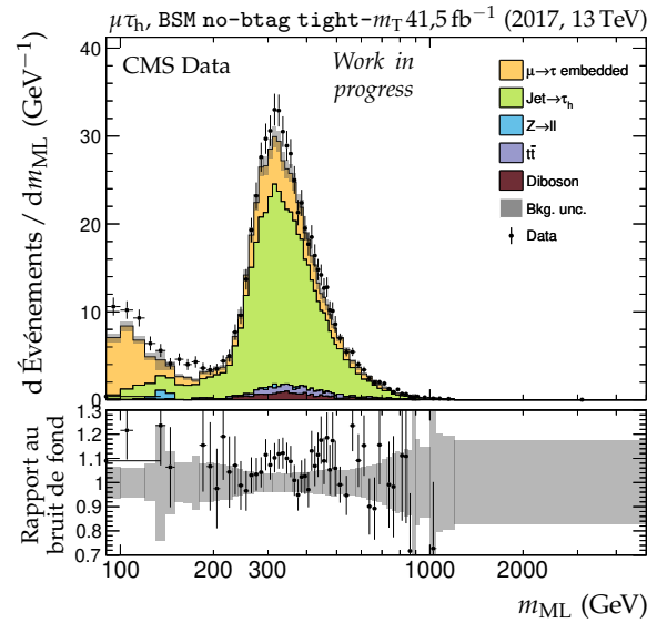
(b) Catégorie BSM no-btag tight- m_{\text{T}} , m_{\text{ML}} .
