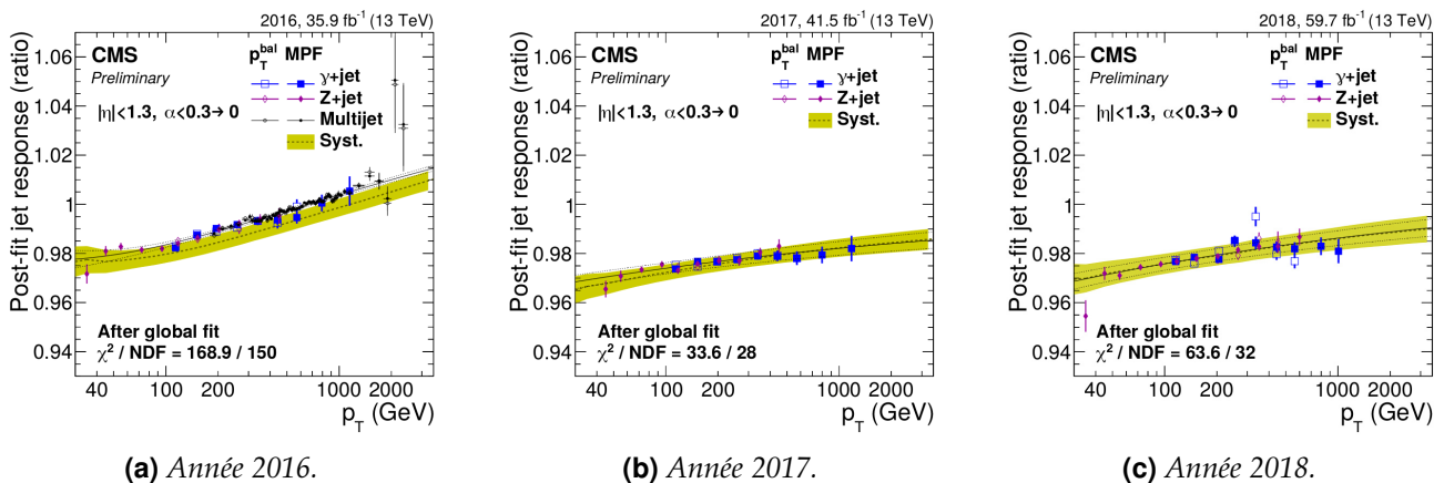
Figure 3.6 – Correction résiduelle absolue en p_T pour |\eta| < 1,3 lors du Run II obtenue par ajustement global sur les événements \gamma + \text{jets} , Z + \text{jets} et multijet [164].
