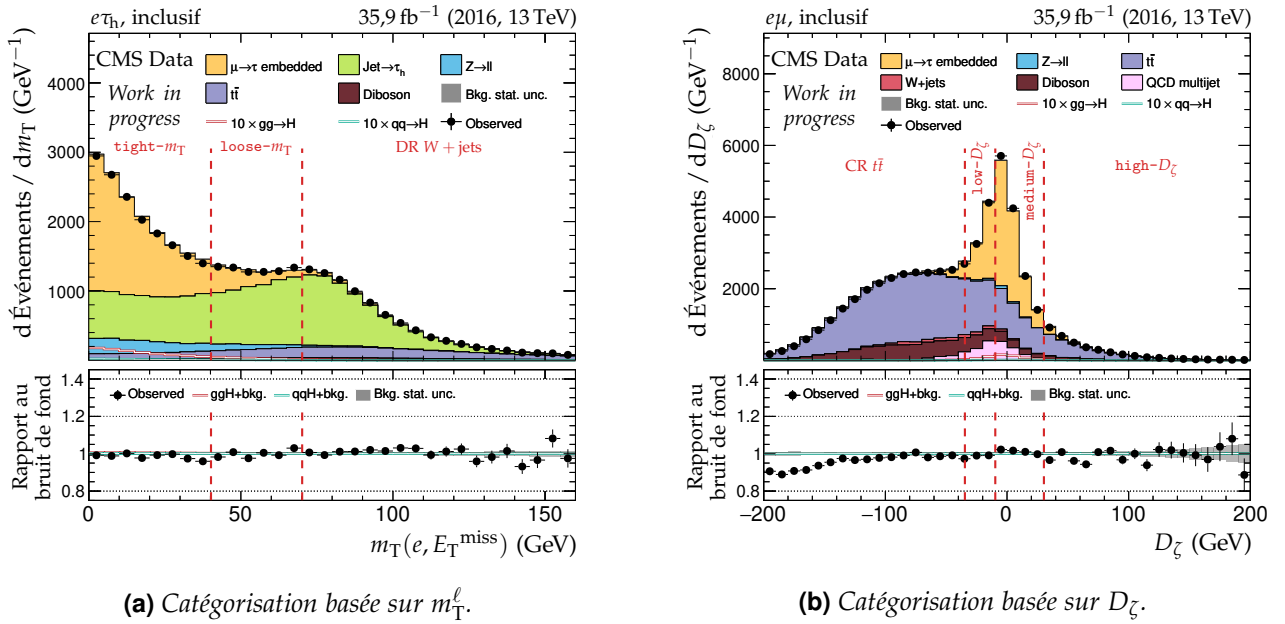
Figure 4.13 – Illustrations des catégorisations basées sur m_T^\ell et D_{Z_i} , respectivement sur les événements des canaux e\tau_h et e\mu de l'année 2016.
