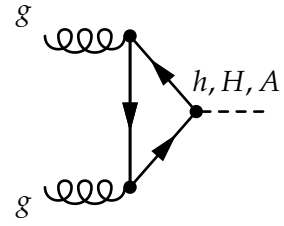
Figure 4.1 – Diagramme de Feynman de production de boson de Higgs dans le cadre du MSSM par fusion de gluons ( ggH ).
