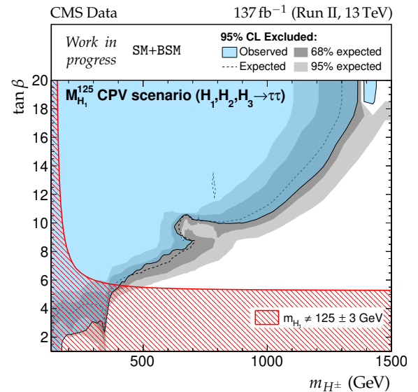
Figure 4.23 – Limites d'exclusion du scénario M_{H_1}^{125} (CPV) dans le plan (m_{H^\pm}, \tan \beta) obtenues avec l'intégralité des données du Run II récoltées par CMS.
