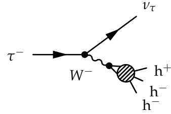
Figure 2.27 – Diagramme de Feynman de désintégration hadronique d'un \tau^- .
