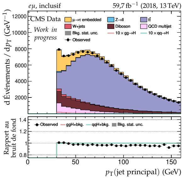
(a) Impulsion transverse du jet principal.
