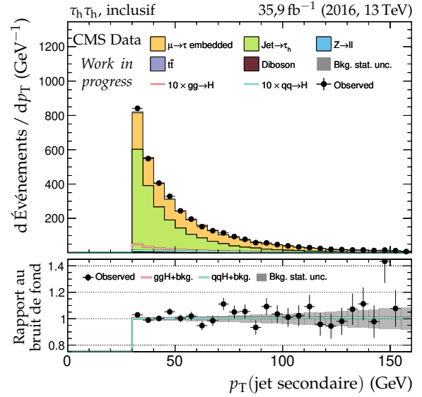
(b) Impulsion transverse du jet secondaire.
