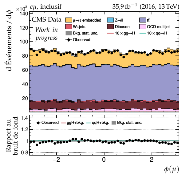
(f) Angle azimutal du lepton 2 ( \mu ).
