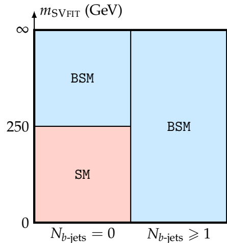
Figure 4.19 – Définition des deux régions utilisant des catégories différentes.
