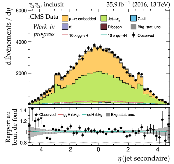
(d) Pseudo-rapacité du jet secondaire.
