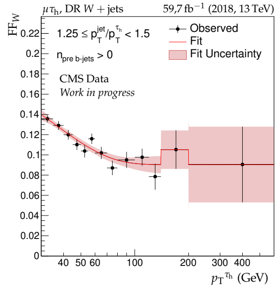
Figure 4.9 – Ajustement de FF_W dans le canal \mu\tau_h en 2018 [209].
