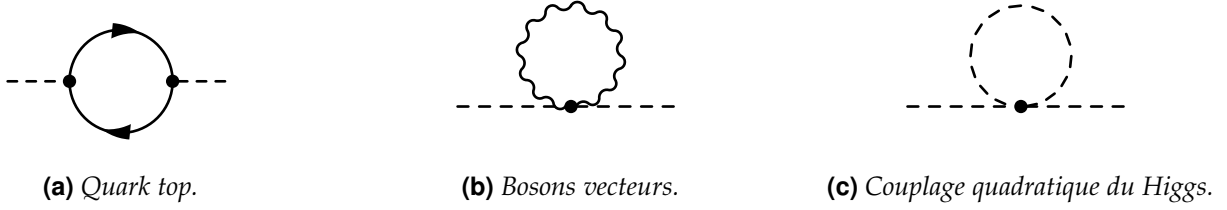
Figure 1.17 – Diagrammes de Feynman des contributions aux corrections radiatives à la masse du boson de Higgs.
