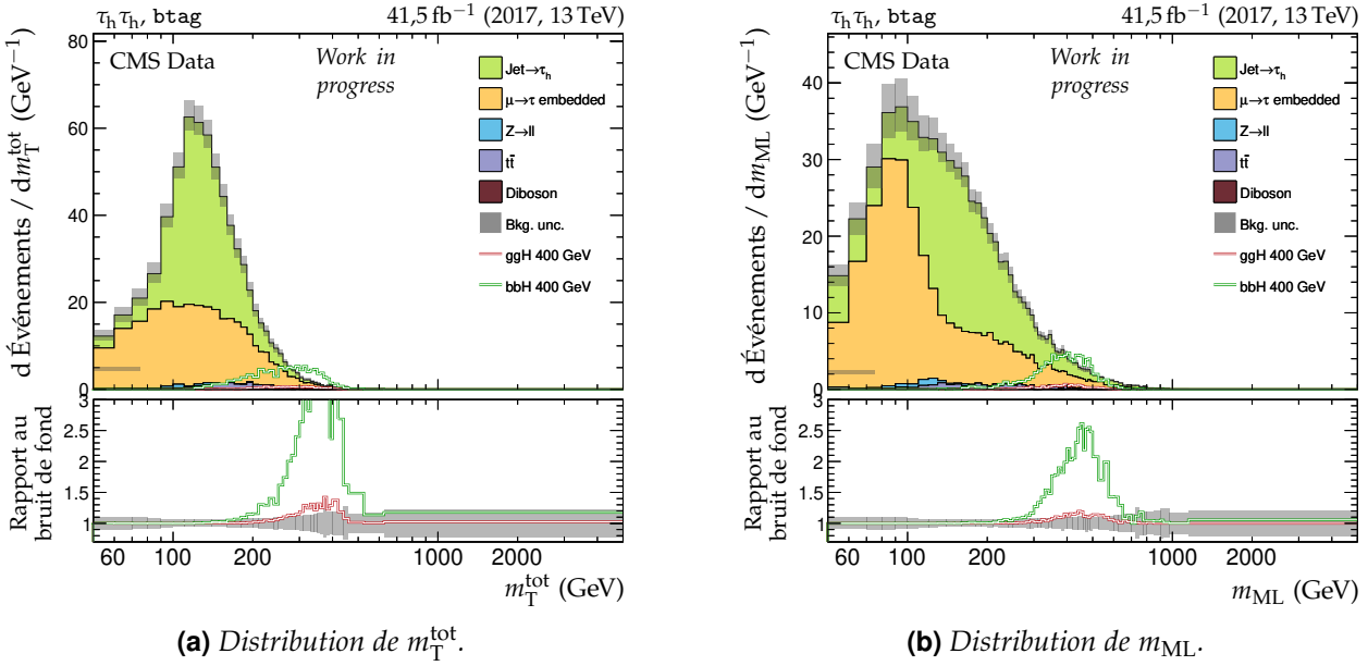
Figure 5.42 – Distributions de m_T^{tot} et m_{ML} en 2017 dans la catégorie btag du canal \tau_h\tau_h . Un signal correspondant à un boson de Higgs supplémentaire de masse 400 GeV est ajouté à titre d'illustration.
