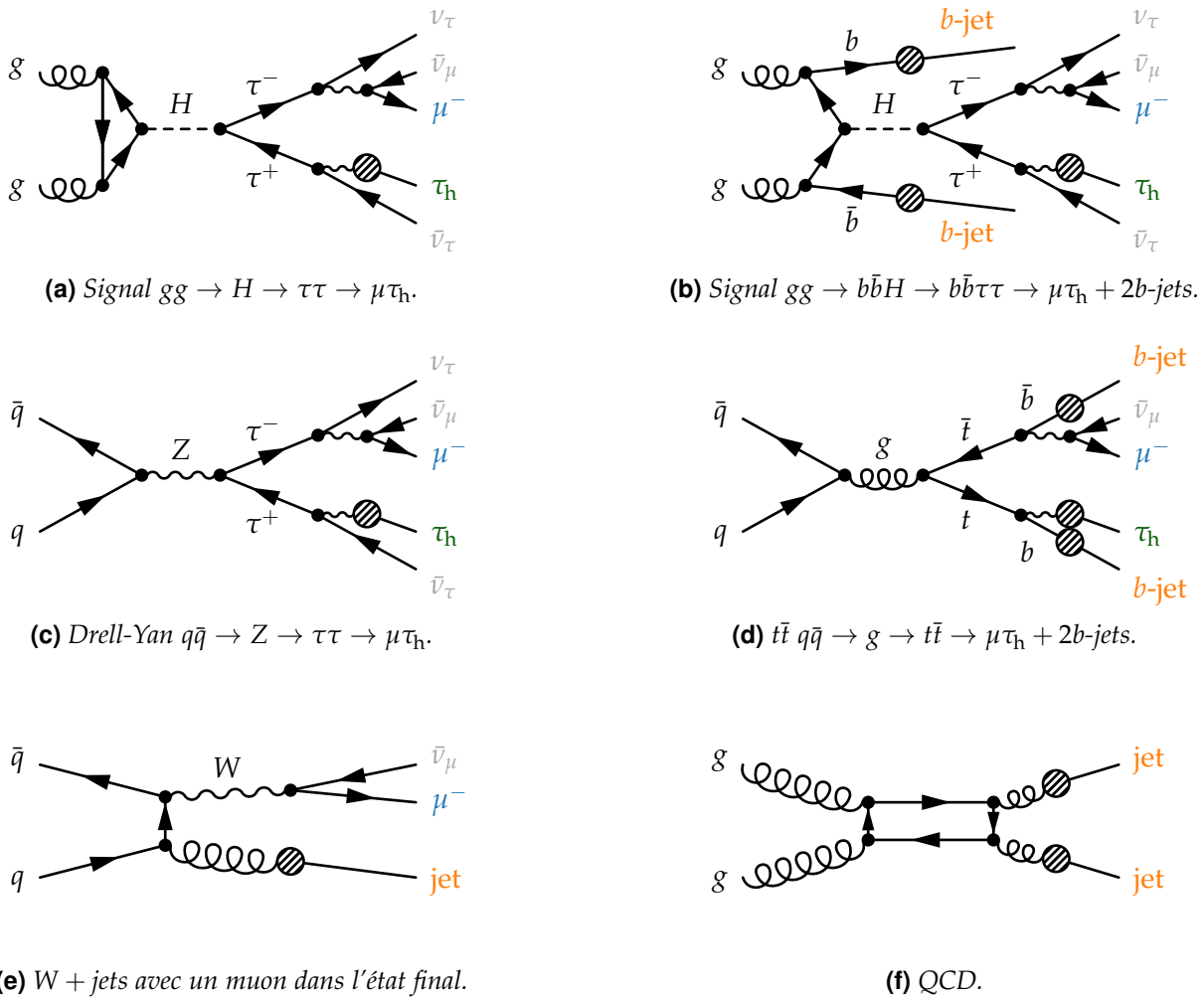
Figure 4.3 – Diagrammes de Feynman complets des signaux ggH (4.3a) et b\bar{b}H (4.3b) et bruits de fond Drell-Yan (4.3c), t\bar{t} (4.3d), W + \text{jets} (4.3e) et QCD (4.3f) de l'analyse illustrés dans le cas du canal \mu\tau_h .
