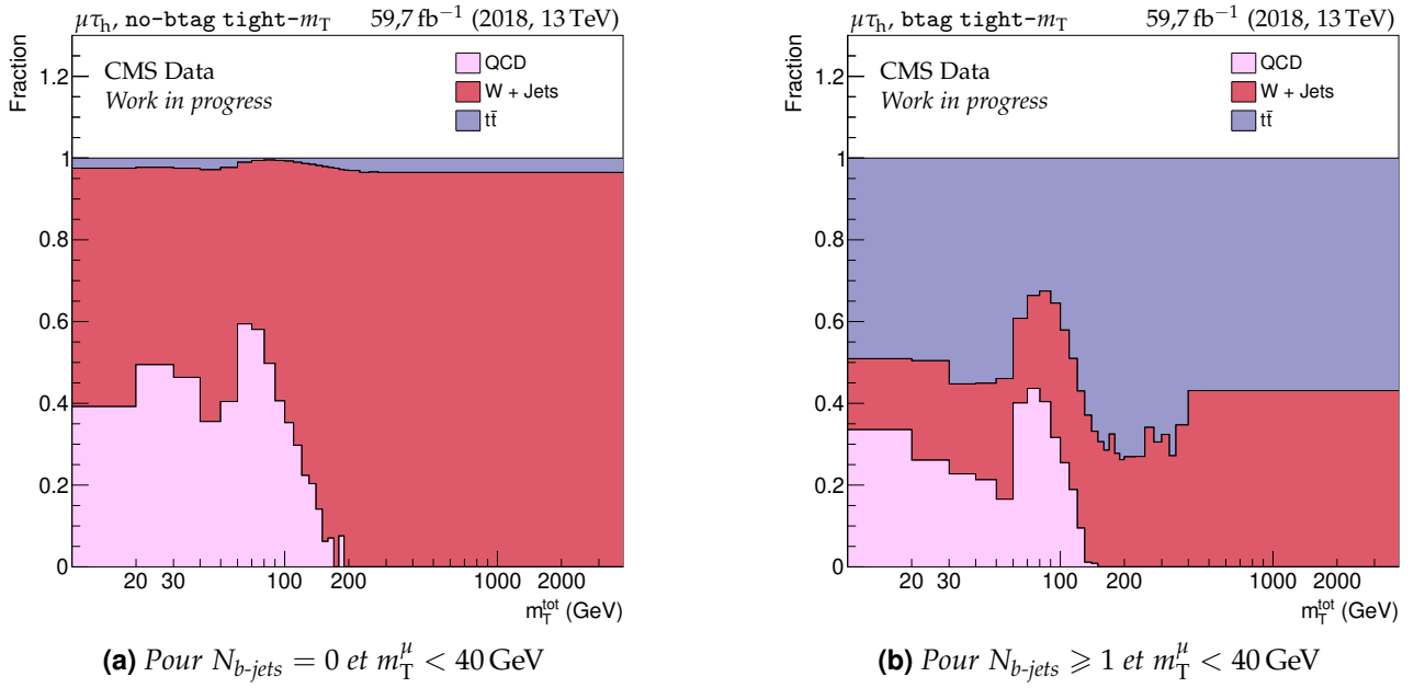
Figure 4.7 – Fractions des sources de faux \tau_h dans le canal \mu\tau_h en 2018 [209].
