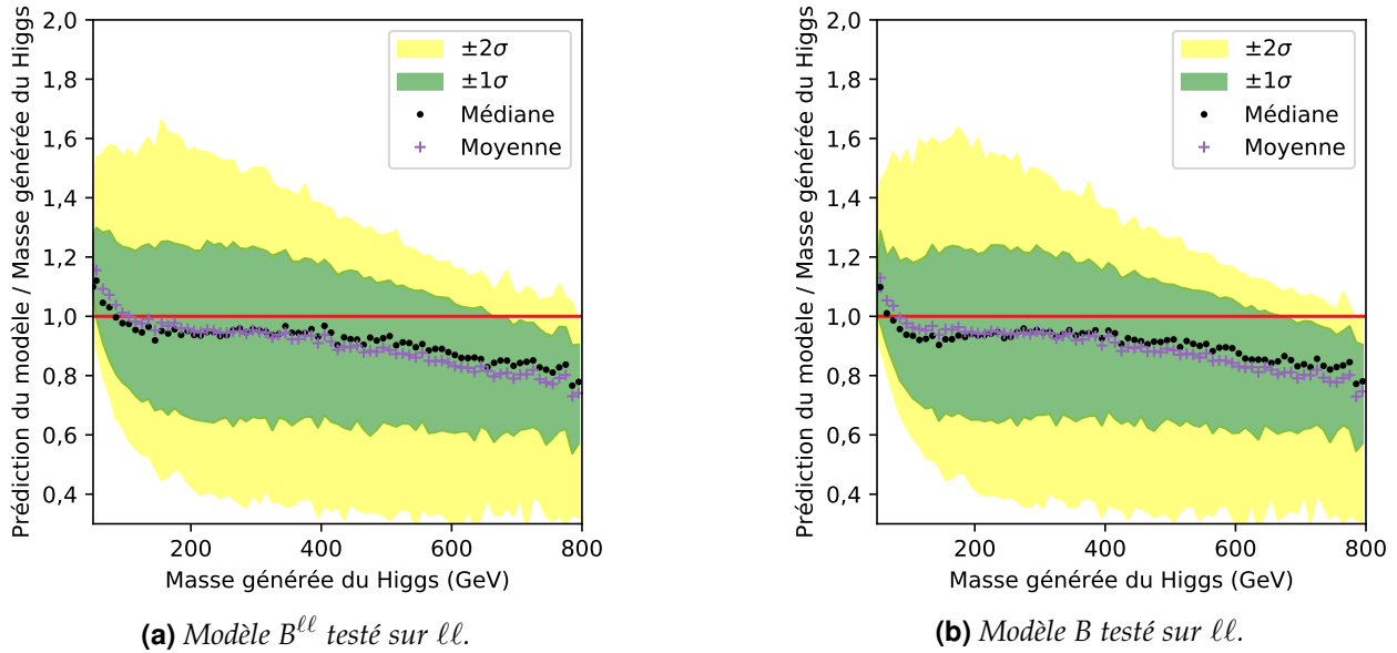
Figure 5.31 – Comparaison de B^{\ell\ell} à B .
