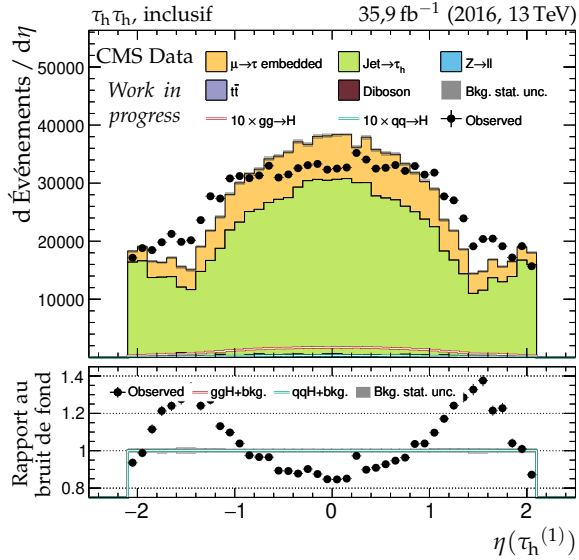
(c) Pseudo-rapidité du lepton 1 ( \tau_h^{(1)} ).
