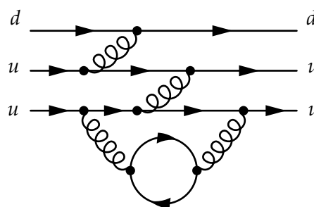
Figure 2.3 – Diagramme de Feynman de la propagation d'un proton avec apparition d'une paire q\bar{q} .
