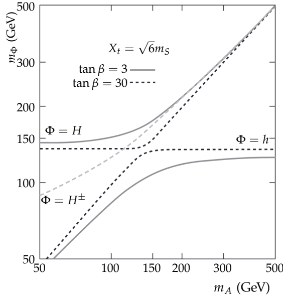
Figure 1.18 – Masses des bosons de Higgs du MSSM en fonction de m_A pour \tan \beta = 3 et 30 dans le cas de mélange maximal du stop avec m_{\tilde{t}} = 2 TeV et les autres paramètres de la SUSY fixés à 1 TeV [68].
