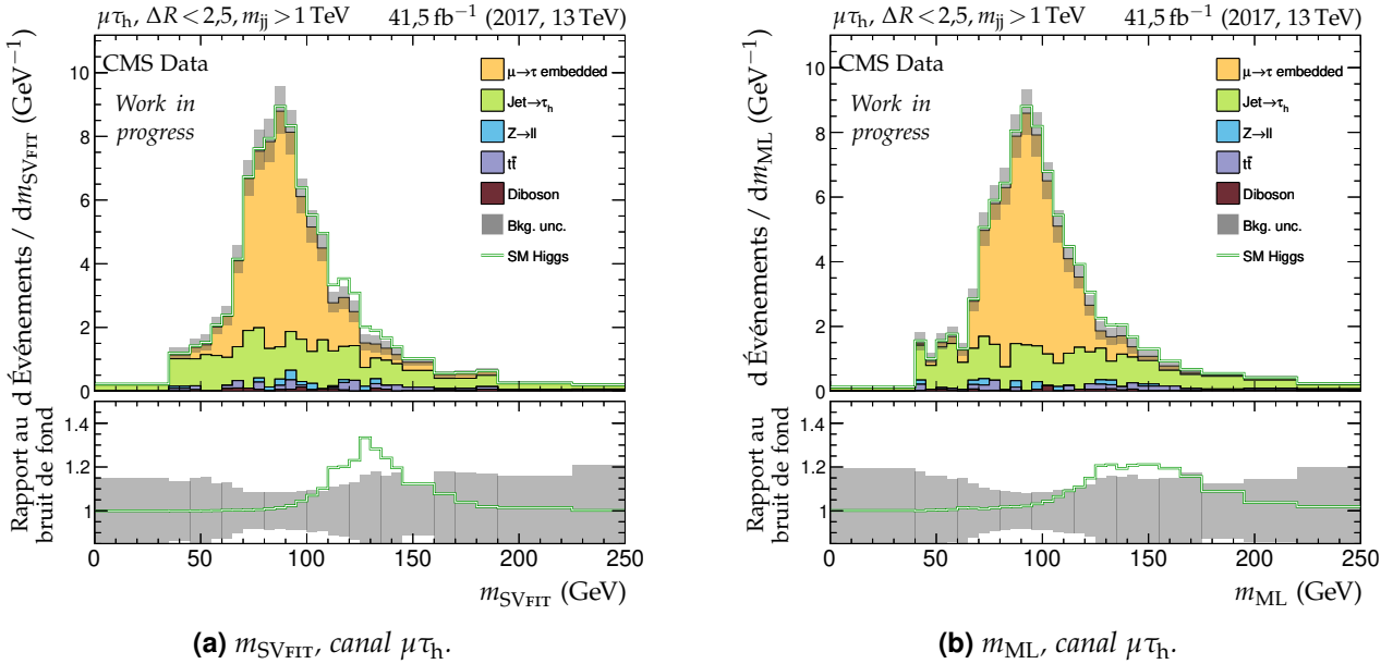
Figure 5.50 – Distributions de m_{\text{SVFIT}} et m_{\text{ML}} en 2017 dans le canal \mu\tau_h avec les événements contenant au moins deux jets avec la masse invariante des deux jets principaux m_{jj} supérieure à 1 TeV et tels que la distance \Delta R entre les deux éléments du dilepton dans le plan (\eta, \phi) soit inférieure à 2,5.
