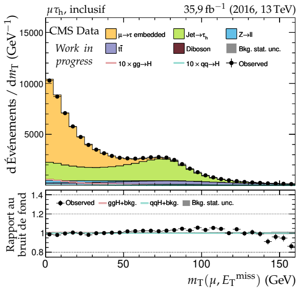
(a) Masse transverse du lepton 1 ( \mu ).
