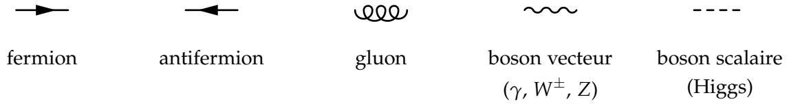
Figure C.3 – Types de particules et lignes correspondantes dans les diagrammes de Feynman.
