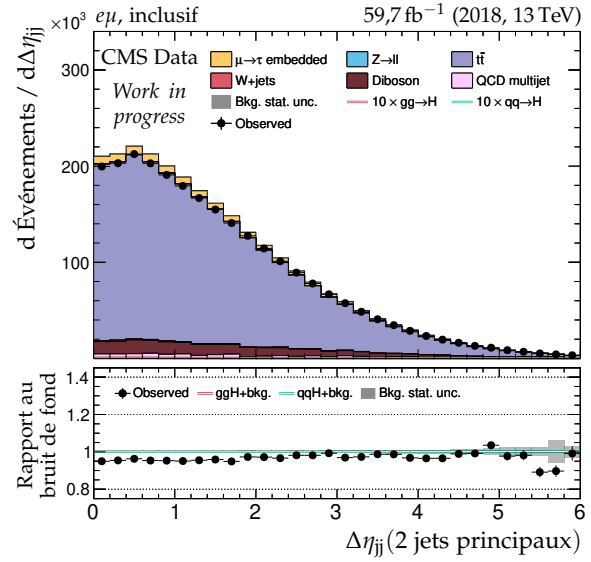
(d) Distance en \eta entre les deux jets.
