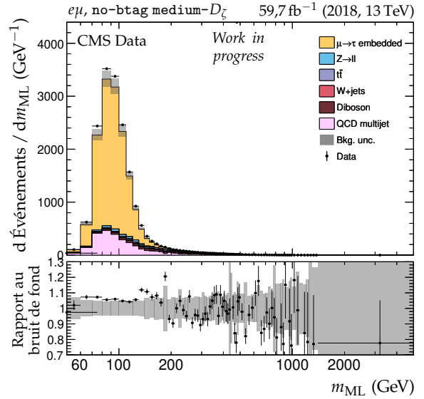
(d) Catégorie no-btag medium- D_{\zeta_i} , m_{\text{ML}} .
