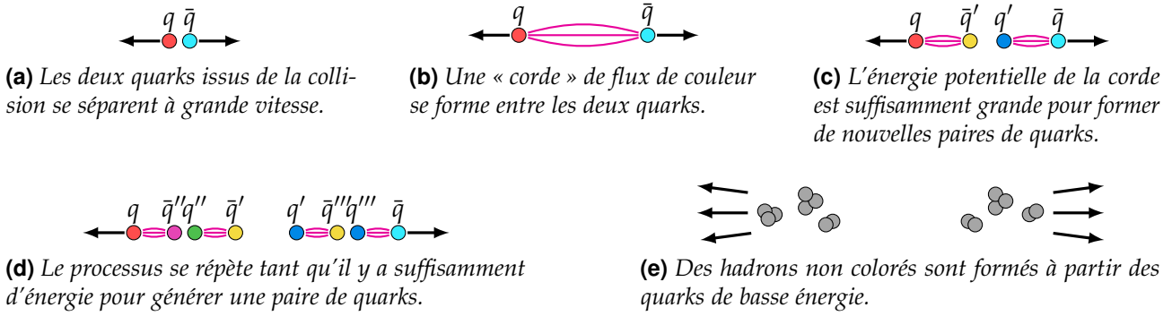
Figure 1.15 – Processus de formation de deux jets dans le cadre du modèle des cordes de Lund.
