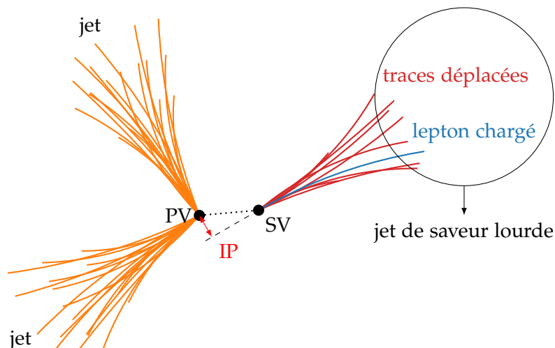
Figure 1.16 – Trois jets, dont un de saveur lourde. Les particules composant ce jet proviennent d'un vertex secondaire (SV), différent du vertex primaire (PV) où a lieu la collision entre les protons et la formation du hadron lourd à l'origine du SV. Le paramètre d'impact (IP) est également indiqué. Réalisé à l'aide de CMSTransverseTikZ [51].
