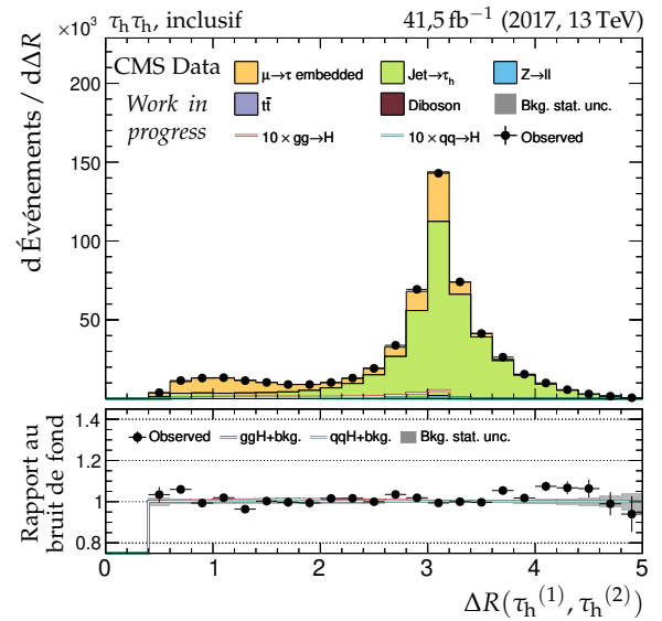
(f) Distance \Delta R entre les leptons ( \tau_h^{(1)} , \tau_h^{(2)} ).
