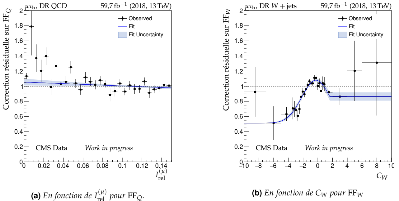
Figure 4.11 – Corrections résiduelles des facteurs de faux dans le canal \mu\tau_h en 2018 [209].
