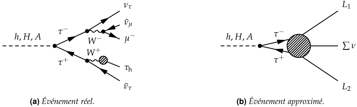
Figure 4.15 – Diagrammes de Feynman d'un événement H \rightarrow \tau\tau \rightarrow \mu\tau_h , avec trois neutrinos dans l'état final.
