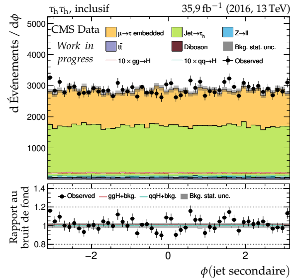
(f) Angle azimutal du jet secondaire.
