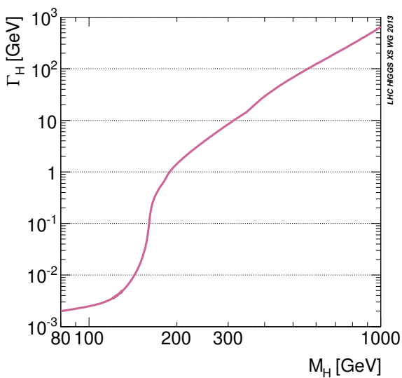
(a) Largeur du boson de Higgs du modèle standard [85].
