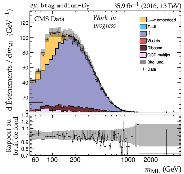
(d) Catégorie btag medium- D_{\zeta} , m_{\text{ML}} .
