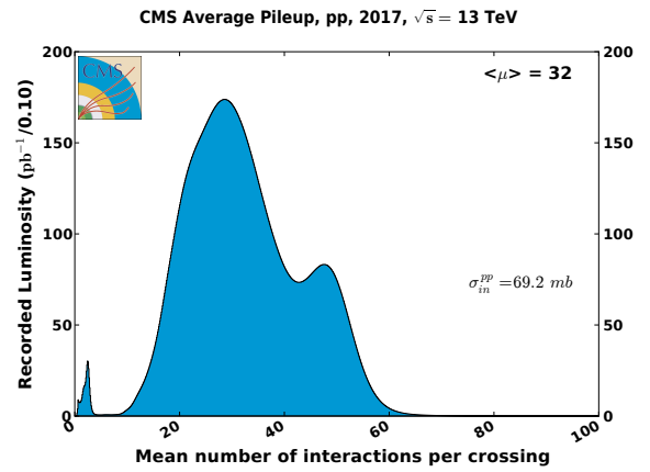
(b) Distribution du nombre moyen d'interactions par croisement de faisceaux en 2017.
