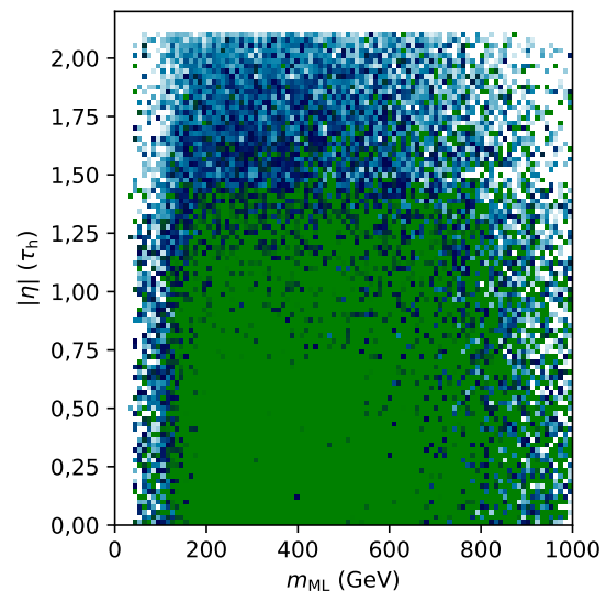
Figure G.1 – Distribution de |\eta|(\tau_h) en fonction de m_{ML} .
