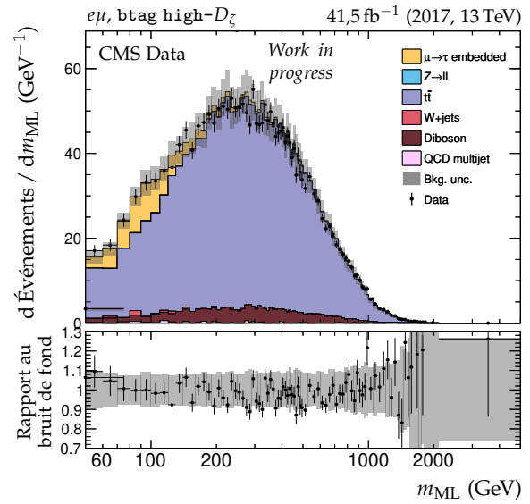
(b) Catégorie btag high- D_{\zeta} , m_{\text{ML}} .
