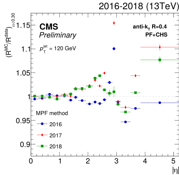
Figure 3.5 – Correction résiduelle relative en \eta lors du Run II [164].
