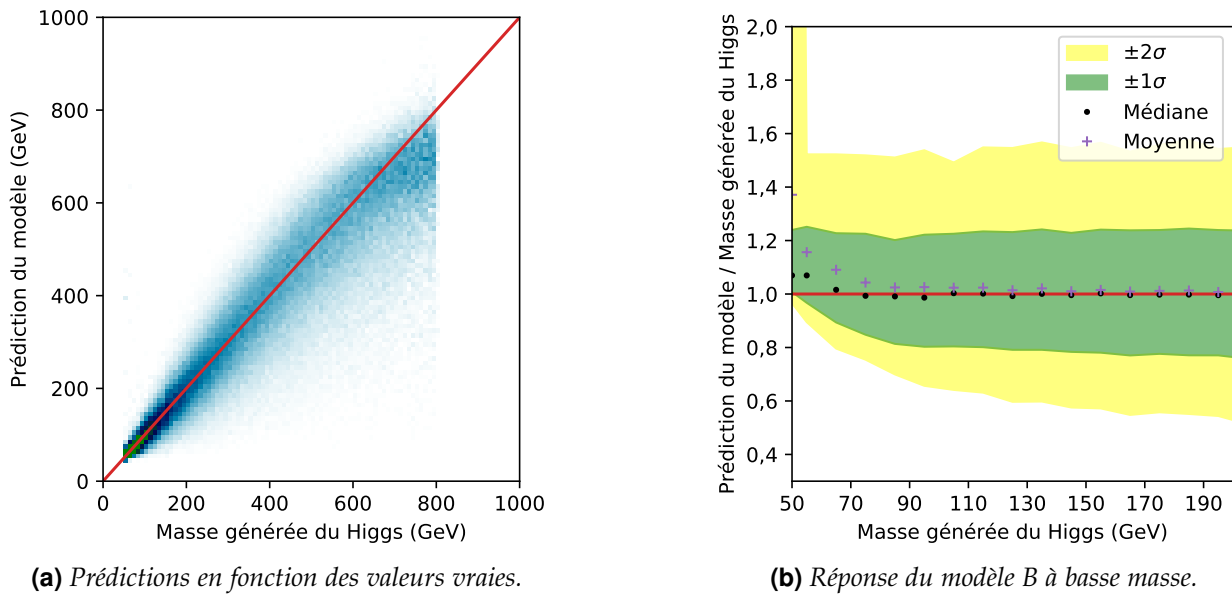
Figure 5.35 – Performances du modèle B.
