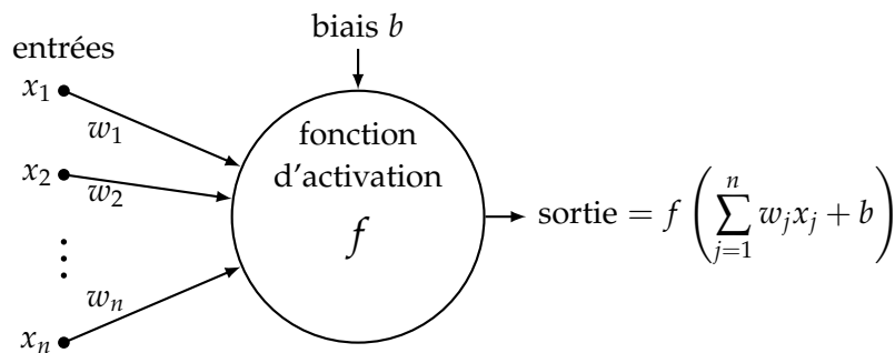
Figure 5.6 – Structure d'un neurone. Une fonction f dite d'« activation » est appliquée à la somme des entrées x_j pondérées par les poids w_j et du biais b afin d'obtenir la valeur de sortie.
