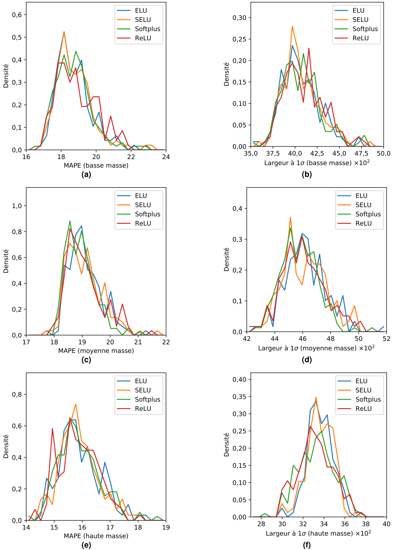
Figure 5.20 – Évaluations des DNNs regroupés selon la fonction d'activation par L_{\text{MAPE}} et \Delta_{1\sigma} .
