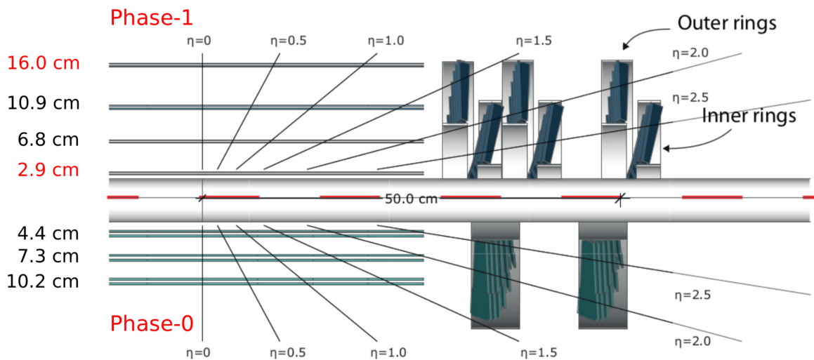
Figure 2.13 – Comparaison des trajectographes à pixels utilisés en 2016 (Phase-0, en bas) et à partir de 2017 (Phase-1, en haut) [130, 133].
