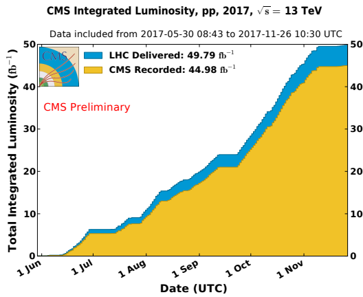
(a) Luminosité totale délivrée par le LHC et enregistrée par le détecteur CMS en fonction du temps en 2017.
