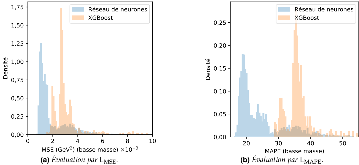
Figure 5.14 – Évaluations des XGBs et des DNNs par L_{MSE} et L_{MAPE} à basse masse.
