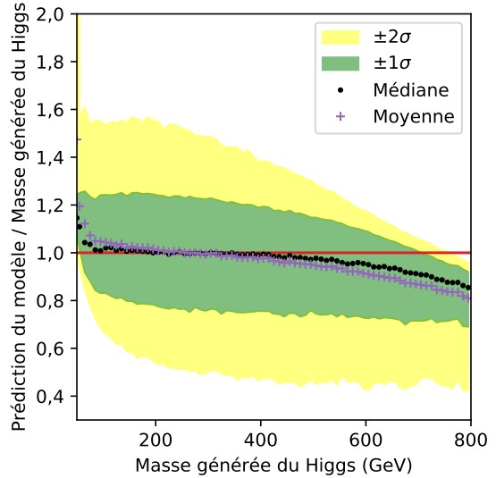
Figure 5.21 – Réponse du modèle A.
