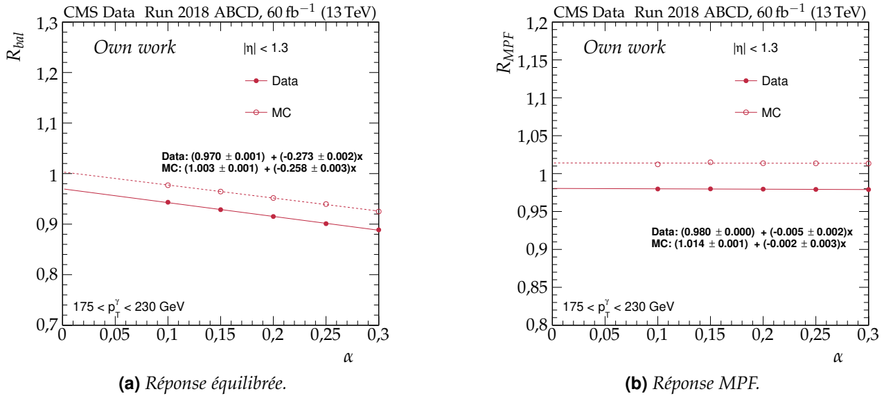
Figure 3.19 – Extrapolation vers \alpha = 0 de la réponse des jets pour |\eta| < 1,3 et 175 < p_T^\gamma < 230 GeV en 2018.
