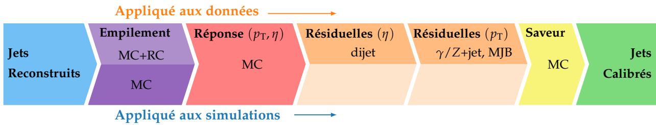
Figure 3.1 – Étapes successives de la JEC pour les données réelles (« données ») et simulées (« simulations ») [156]. Les corrections des étapes marquées « MC » sont obtenues par l'étude de simulations, celles marquées « RC » par une méthode de cône aléatoire (Random Cone) sur les données réelles. Les types d'événements utilisés dans les corrections résiduelles sont également indiqués.
