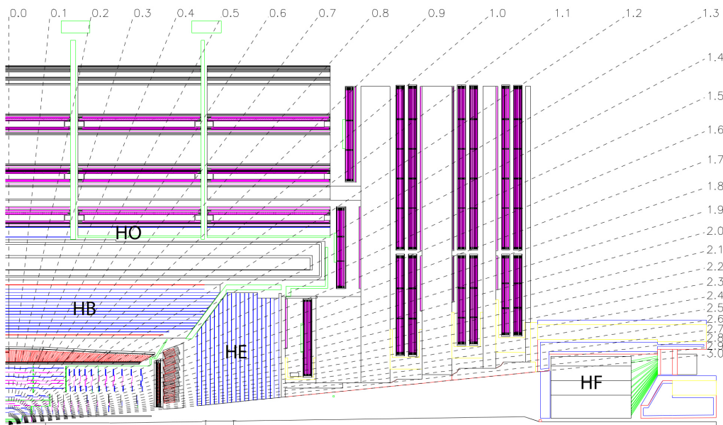
Figure 2.18 – Schéma d'un quadrant du détecteur CMS [114] montrant la localisation des calorimètres hadroniques du tonneau (HB), externe (HO), du bouchon (HE) et vers l'avant (HF). Certaines valeurs de \eta et les directions associées sont indiquées.
