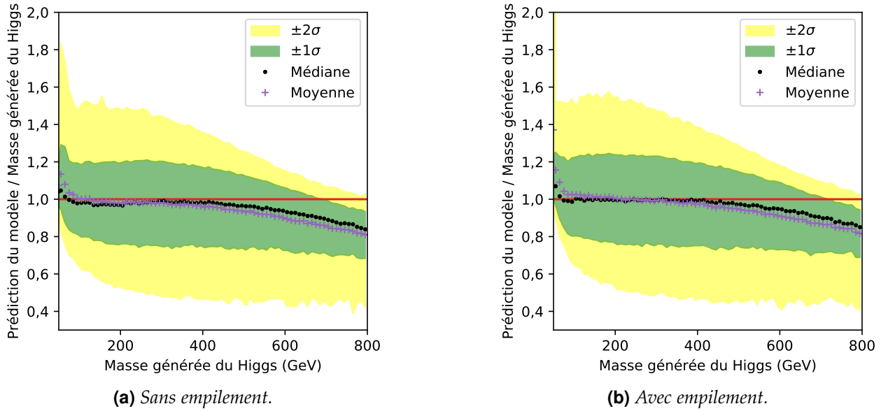
Figure 5.24 – Réponses du modèle B sur les événements sans et avec empilement.
