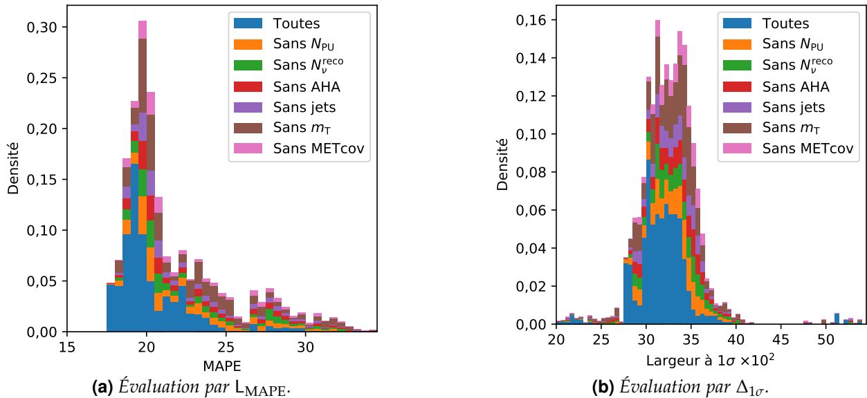
Figure 5.10 – Évaluations des XGBs regroupés selon les variables d'entrée.
