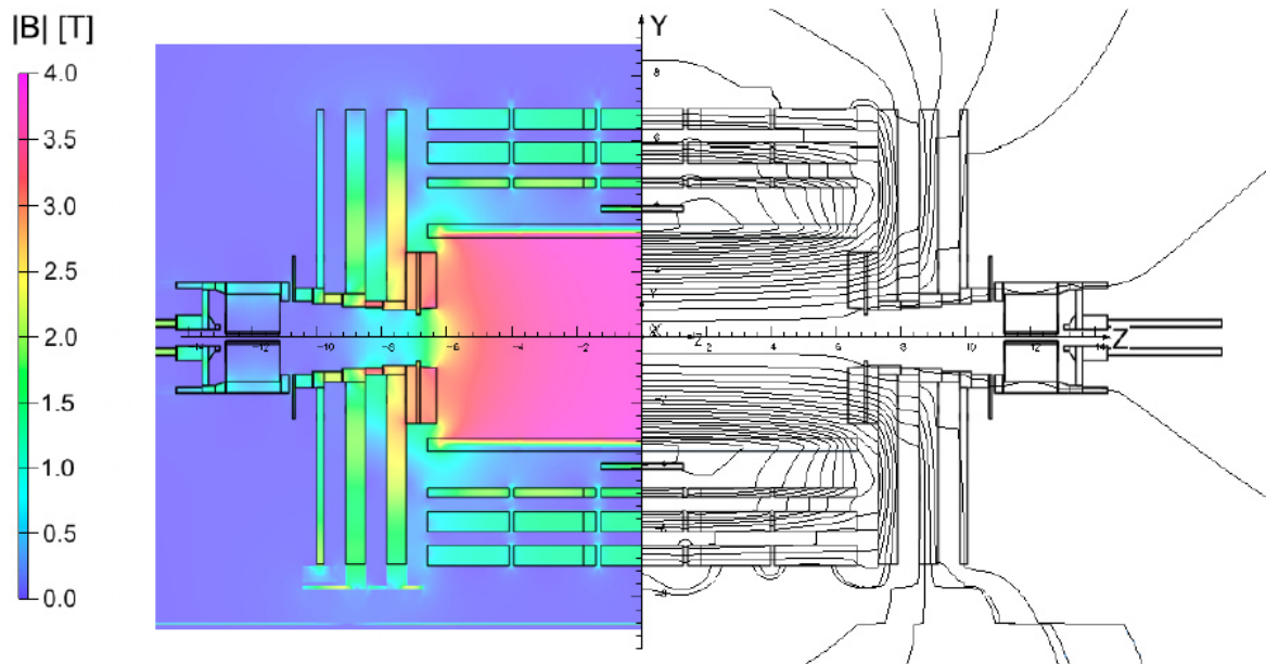
Figure 2.11 – Valeurs de la norme du champ magnétique (à gauche) et lignes de champ (à droite) prédites dans la section longitudinale du détecteur CMS avec une valeur du champ au centre de 3,8 T [129]. Chaque ligne de champ correspond à un flux magnétique de 6 Wb.
