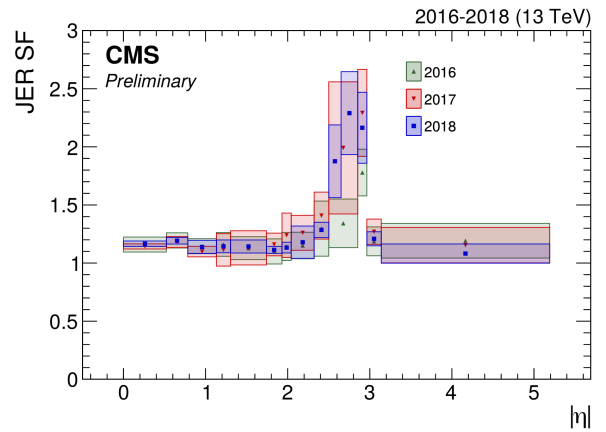
(b) Facteurs correctifs utilisés par la collaboration lors du Run II [164].
