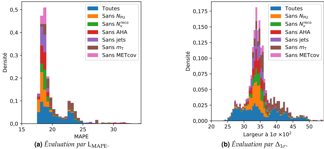
Figure 5.11 – Évaluations des DNNs regroupés selon les variables d'entrée.
