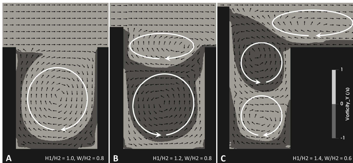
Fig. 14 – Régimes d'écoulement, vecteurs vitesse et vorticité selon y pour différents ratios H1/H2 et W/H2 (Reiminger et al., 2020c).
