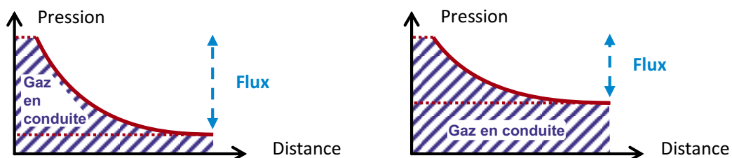
Figure 3: Arbitrage entre capacité de transport et stockage de gaz en conduite
