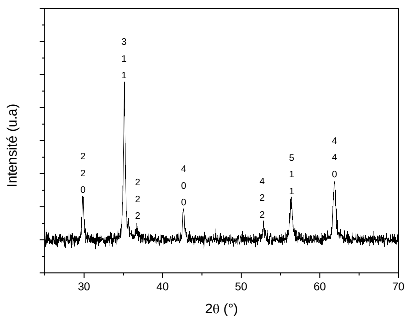
Figure 3 : Diagramme de diffraction des rayons X d'un échantillon \text{MnFe}_2\text{O}_4 synthétisé par coprécipitation inverse avec un pH de 12, une température de 80 °C
