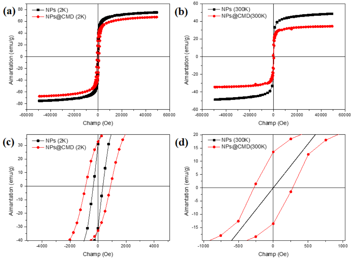
Figure 14 : Courbes d'aimantation des nanoparticules \text{MnFe}_2\text{O}_4 synthétisées par coprécipitation avec MIPA, nues et fonctionnalisées par CMD en fonction du champ magnétique appliqué à 2 K (a) et 300 K (b), et des agrandissements des deux courbes sont donnés respectivement en (c) et (d)
