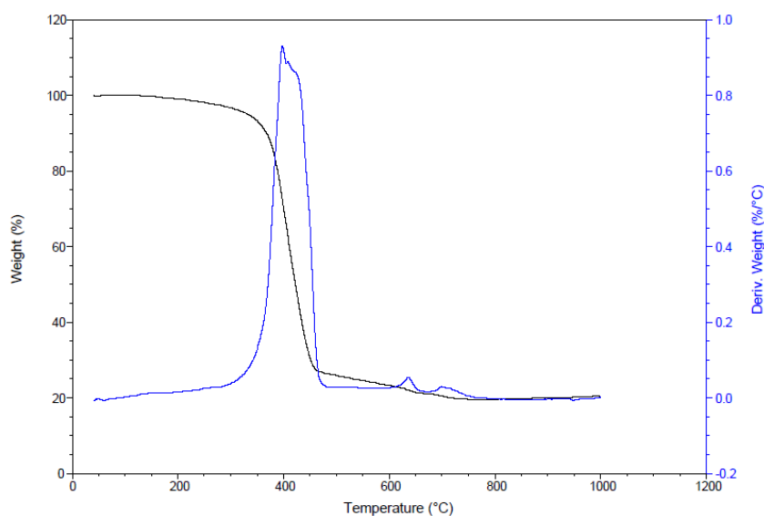
Figure 10 : courbe d'ATG d'un échantillon \text{MnFe}_2\text{O}_4 synthétisé par décomposition thermique
