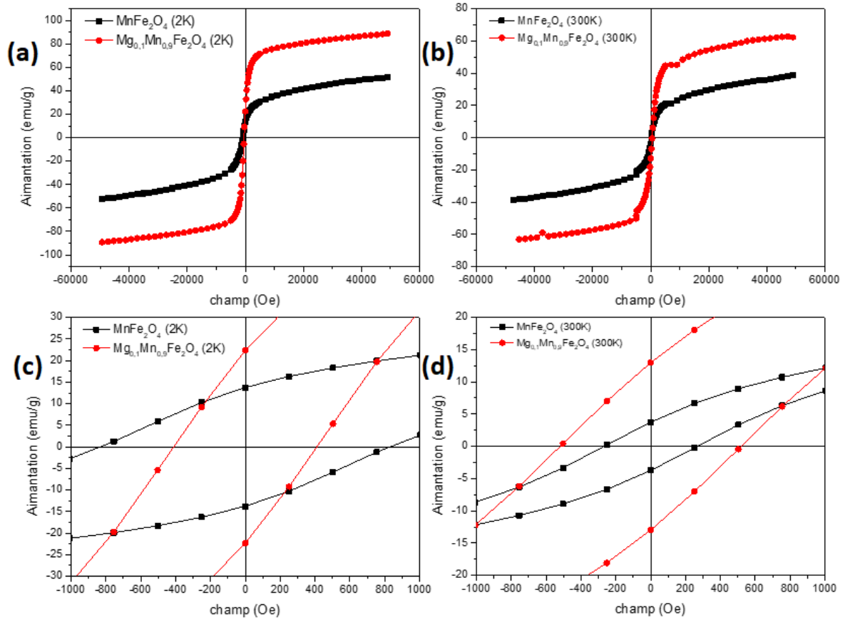
Figure 37 : Courbes d'aimantation des nanoparticules \text{MnFe}_2\text{O}_4 et \text{Mg}_{0.1}\text{Mn}_{0.9}\text{Fe}_2\text{O}_4 en fonction du champ magnétique appliqué à 2 K (a) et 300 K (b), et des agrandissements des deux courbes sont donnés respectivement en (c) et (d)
