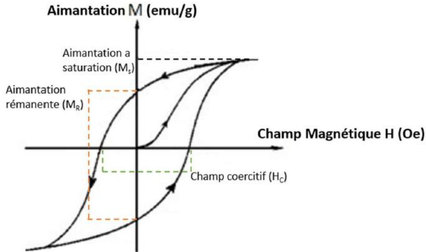
Figure 5 : Cycle d'hystérèse : aimantation en fonction du champ magnétique appliqué, pour un matériau ferro/ferrimagnétique
