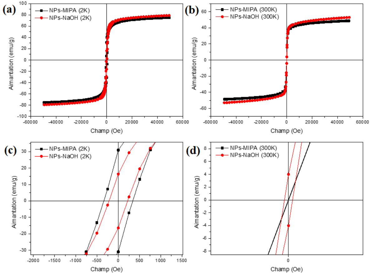
Figure 12 : Courbes d'aimantation des nanoparticules \text{MnFe}_2\text{O}_4 synthétisées par coprécipitation avec MIPA et NaOH en fonction du champ magnétique appliqué à 2 K (a) et 300 K (b), et des agrandissements des deux courbes sont donnés respectivement en (c) et (d)
