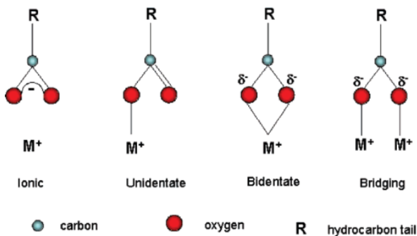
Figure 3 : Modes de coordination des carboxylates métalliques à la surface des nanoparticules de ferrites (pour la simplicité, le métal monovalent est montré au lieu du trivalent)
