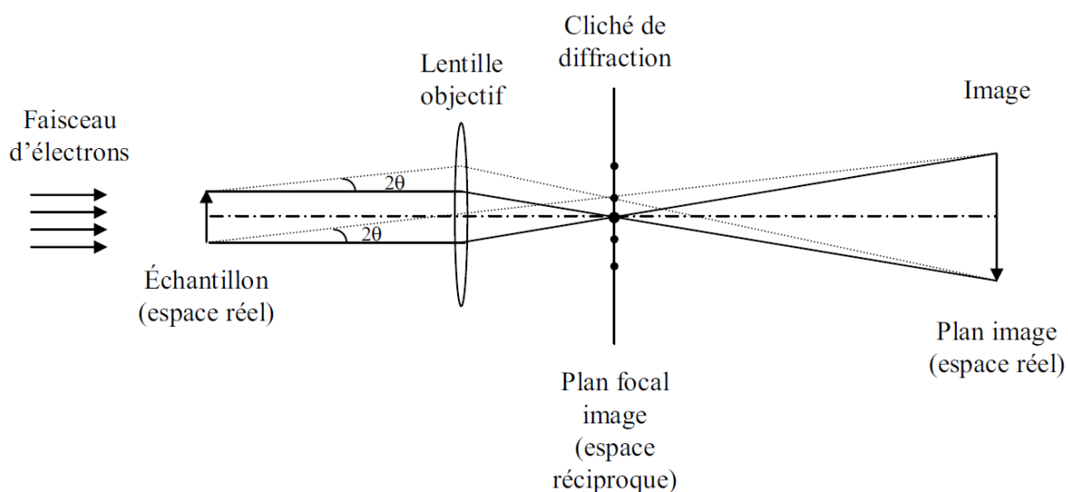
Figure 7 : Trajet optique avec une lentille objectif montrant les principes du processus d'imagerie du MET.
