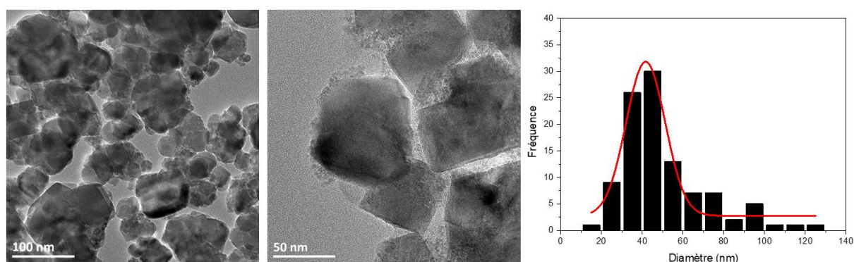
Figure 4 : Images TEM d'un échantillon \text{MnFe}_2\text{O}_4 synthétisé par coprécipitation inverse sur une échelle de 100 et 50 nm et la distribution de taille calculée par ImageJ et ajustée avec une gaussienne
