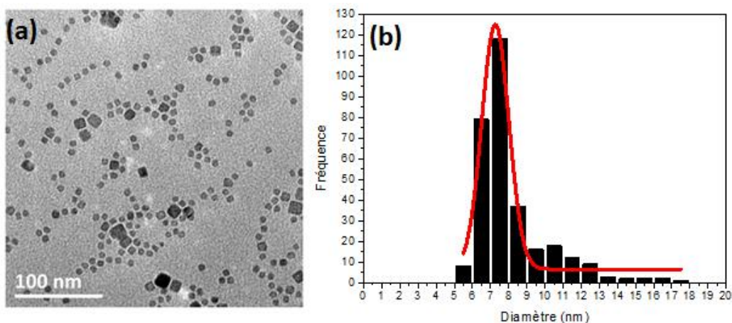
Figure 8 : Image TEM des NPs de \text{MnFe}_2\text{O}_4 synthétisées avec le protocol standard (a) et la distribution de taille calculée par ImageJ et ajustée avec une gaussienne (b)
