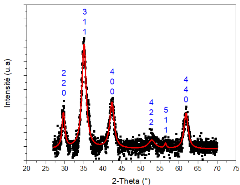
Figure 7 : Diffractogramme des rayons X de l'échantillon MFO1
