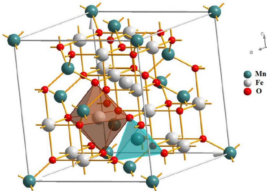
Figure 3 : Structure spinelle de la ferrite MnFe_2O_4 avec les ions Mn dans les site A et les ions Fe dans les sites B
