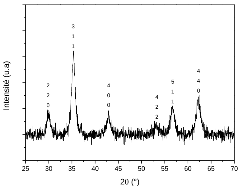
Figure 5 : diagramme de diffraction des rayons X de l'échantillon \text{MnFe}_2\text{O}_4 synthétisé par coprécipitation avec MIPA
