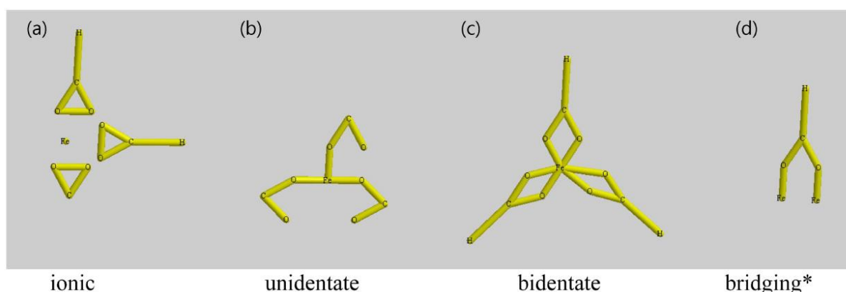
Figure 22 : Les quatre modes de coordination différents entre les ions Fe métalliques et les groupements carboxyles: (a) ionique, (b) unidentate, (c) bidentate et (d) bridging*.
