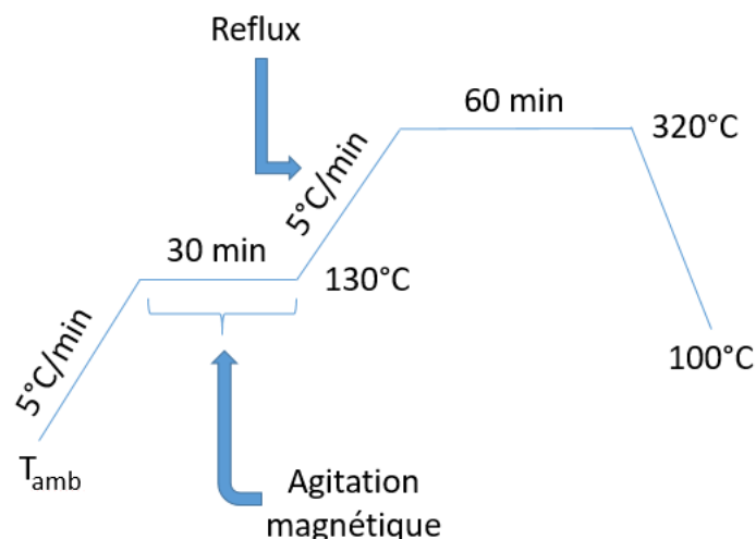
Figure 5 : Schéma représentatif du protocole standard de traitement thermique pour la synthèse de nos NPs de \text{MnFe}_2\text{O}_4 avec les paliers de températures et la vitesse de chauffage
