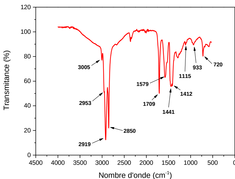
Figure 21 : Le spectre FTIR du complexe d'oléates mixte fer/manganèse
