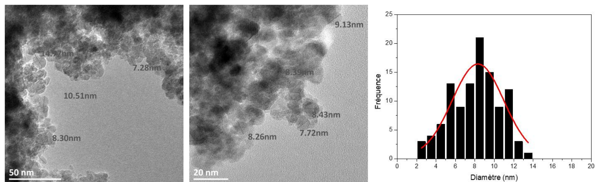
Figure 6 : Images TEM de l'échantillon \text{MnFe}_2\text{O}_4 synthétisé par coprécipitation avec MIPA sur une échelle de 50 et 20 nm et la distribution de taille calculée par ImageJ et ajustée avec une gaussienne
