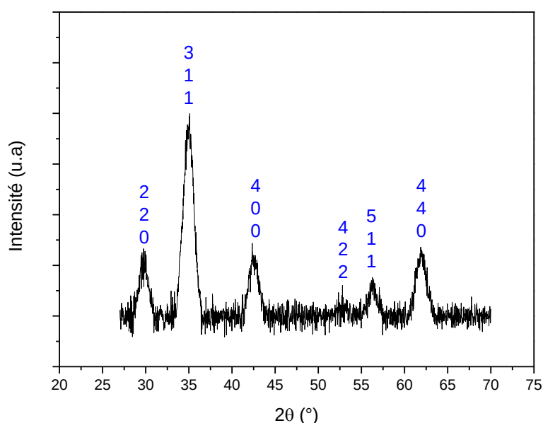
Figure 16 : Diffractogramme des rayons X de l'échantillon MFO5
