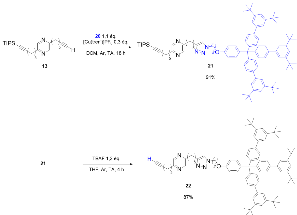
Figure 110. Synth\u00e8se de l'axe mono-bouchonn\u00e9 22 .
