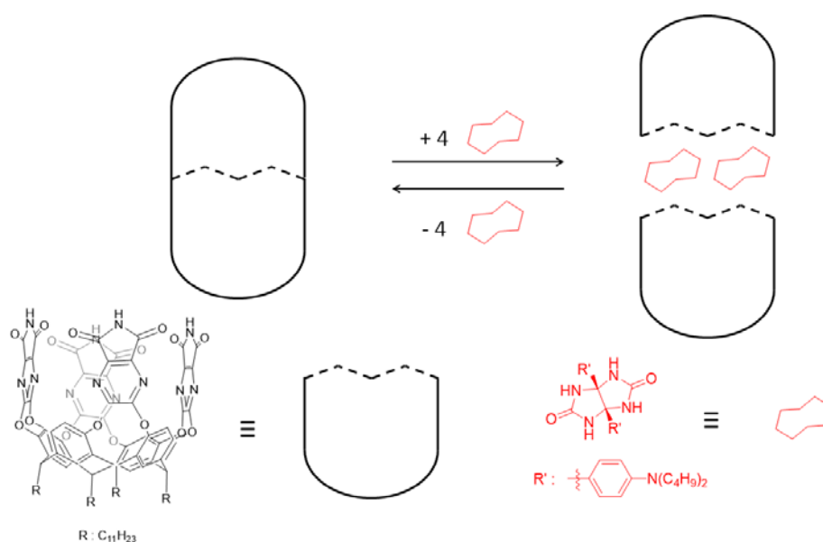
Figure 20. Expansion de la cage de Rebek après ajout d'un excès d'espaceurs glycoluryle (en rouge). 129,105
