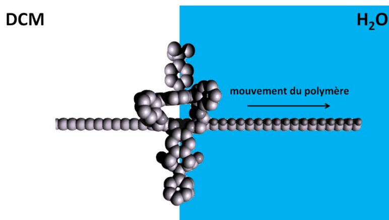
Figure 6. Représentation schématique de l'oxydation du polybutadiène par la cage en présence de 4- tert -butypyridine et de NaOCl dans un mélange DCM/H 2 O (1:1). 49 Adapté de la réf. 49 avec l'autorisation de Nature Publishing Group.
