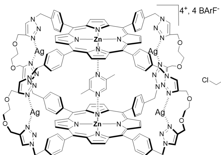
Me-PZ-Me@[Ag 4 C](BARF) 4
