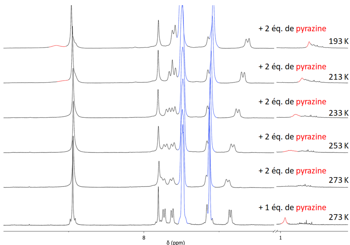
Figure 87. Spectres RMN 1 H ( \text{CD}_2\text{Cl}_2 , 600 MHz, à température variable) de [ \text{Ag}_4\text{C} ](BARF) 4 avec un équivalent de pyrazine (en bas) et suite à l'ajout d'un 2 ème équivalent de pyrazine. Pics rouges : pyrazine, pics bleus : anions.
