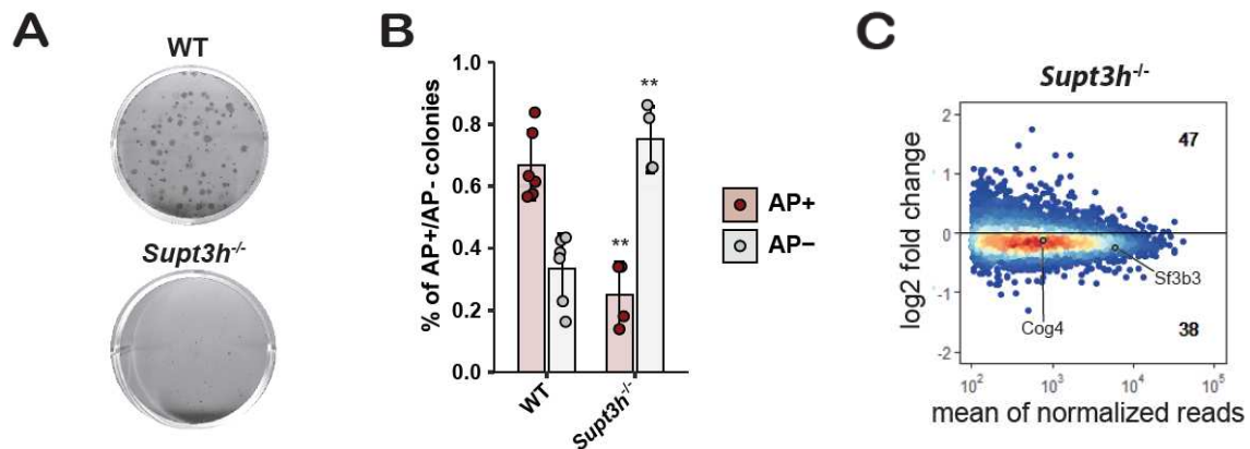
Figure 6: SAGA affecte la maintenance de la pluripotence des ESCs de souris grâce à ses interactions avec TBP. A. Images représentatives de l'analyse clonale des cellules Supt3h -/- dans un milieu contenant du sérum et LIF. L'inactivation de Supt3h affecte la croissance cellulaire. B. Quantification de la coloration à la phosphatase alcaline (AP) des analyses clonales comme indiqué en (A). Le nombre de colonies AP positives (AP+) et AP négatives (AP-) a été normalisé au nombre total de colonies, évalué par coloration au cristal violet. L'inactivation de Supt3h entraîne une réduction du nombre de colonies AP+. n = 4-6. Test de Wilcoxon-Mann-Whitney bilatéral. **, p = 0,009524 . C. Représentation du diagramme de densité des changements de l'expression en log2 du séquençage d'ARN nouvellement synthétisés marqués au 4sU des lignées cellulaires Supt3h -/- par rapport aux cellules contrôles comparés à la moyenne des sondes normalisées. Les lignées cellulaires ont été traitées pendant 24 heures avec IAA. Les nombres en haut et en bas indiquent le nombre de gènes significativement augmentés ou réduits, respectivement. Les gènes ont été considérés comme significativement affectés avec une valeur de p ajustée de < 0,05 et un changement de log2 de < -0,5 ou > 0,5 . Un seuil de 100 sondes a été fixé pour définir les gènes exprimés.
