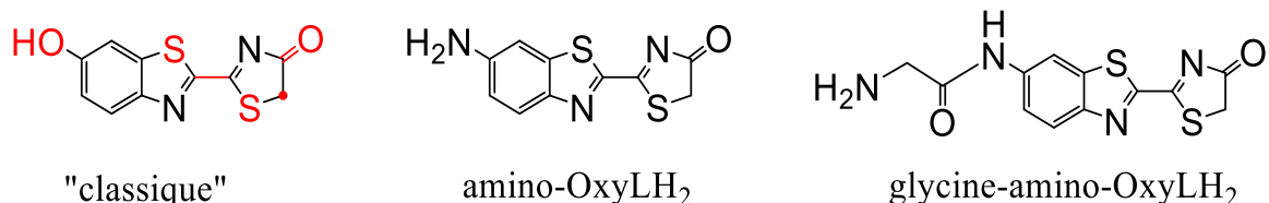
Figure 2 : Trois types de structures analogues à l'oxyluciférine. Les liaisons ou atomes représentés en rouge sur la forme « classique » ont la possibilité d'être substitués par d'autres atomes ou groupements d'atomes.
