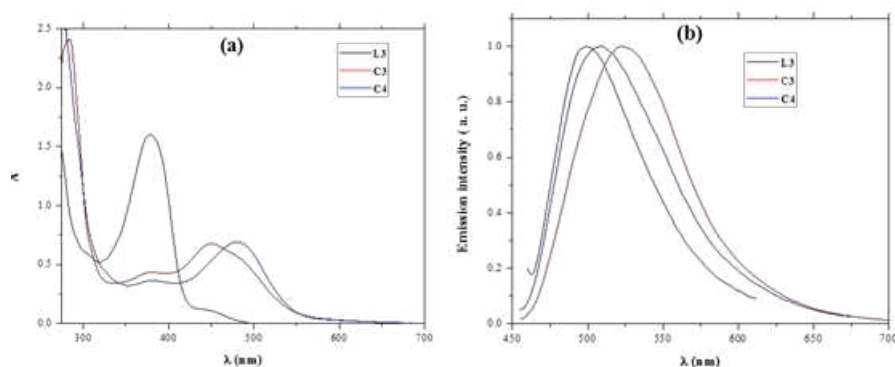
Figure S-3. Spectres (a) d'absorption et (b) d'émission des complexes C3 et C4 en solutions dégazées de DMSO (100 μM).
