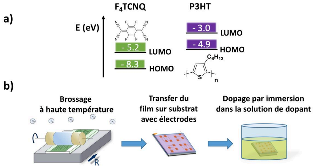
Figure 1. a) Structures moléculaires et niveaux HOMO/LUMO du P3HT et du F 4 TCNQ.
