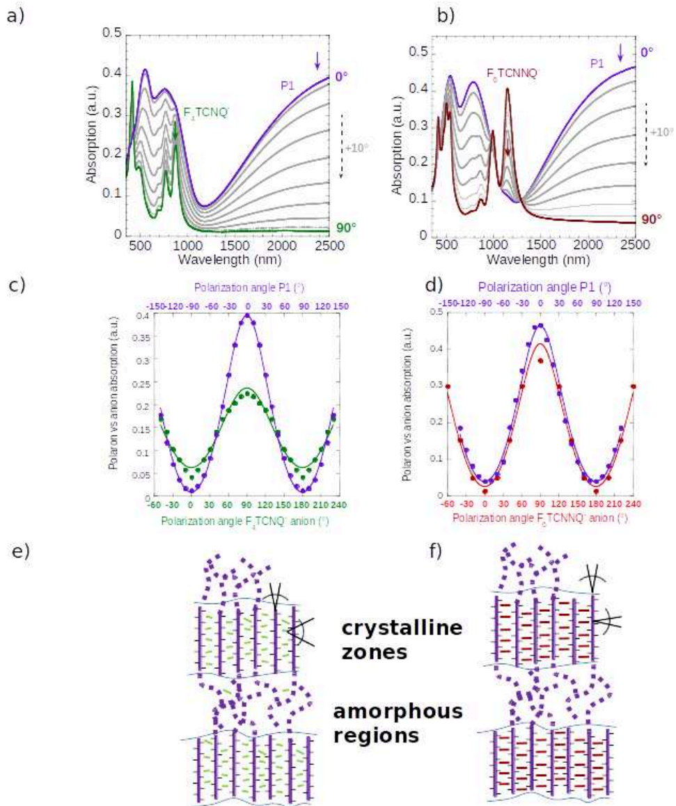
Figure 6: a) et b) Spectres d'absorption UV – Vis – NIR polarisés de films polymères conducteurs orientés pour les films dopés avec F 4 TCNQ et F 6 TCNNQ tracés pour différents angles (tous les 10°) entre la direction de polarisation et la direction du brossage du film. (0° correspond à la lumière incidente polarisée // R (en rouge) alors que 90° correspond à la lumière incidente polarisée ⊥ R (en bleu)). c), d) – Dépendance angulaire de l'absorbance de la bande polaronique P1 à 2500 nm (en rouge), et du dopant à 873 nm (en vert) pour F 4 TCNQ (c) et à 1138 nm (en rouge) pour F 6 TCNNQ (d). e), f) illustration de la différence de l'organisation des dopants dans la structure cristalline du P3HT.
