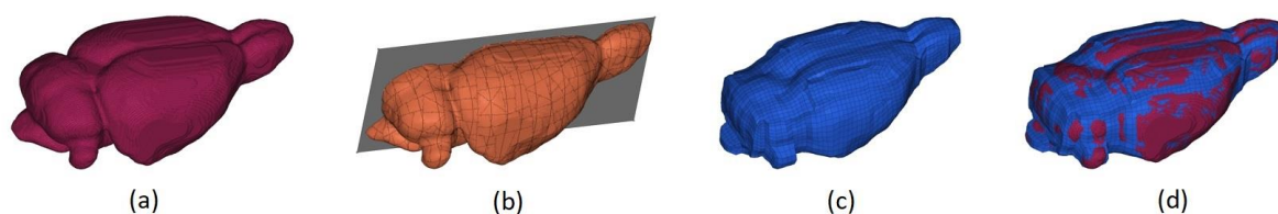
Figure 2.1: Processus de modélisation géométrique et de maillage, (a) représentation STL ; (b) surfaçage ; (c) modèle maillé et (d) représentation STL et modèle maillé coïncidents.
