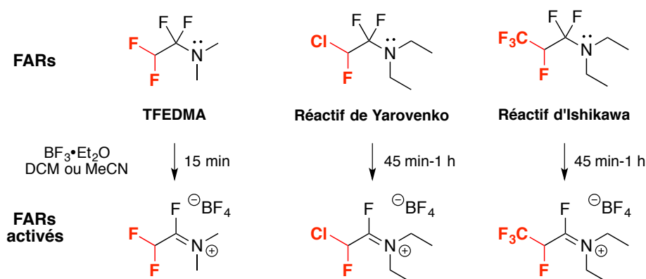
Figure 7: Procédé d'activation des FARs à l'aide d'un acide de Lewis (BF 3 •Et 2 O)
