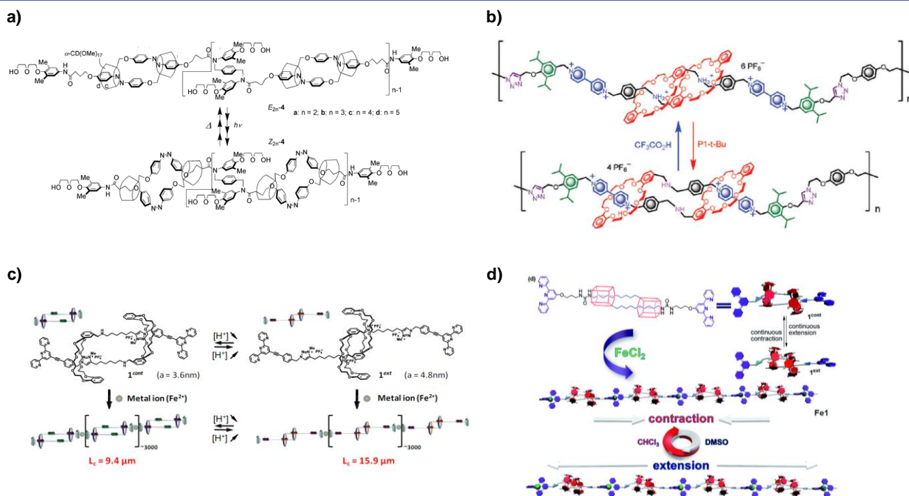
Figure 21 | a) Mouvement de contraction réversible d'oligomères de rotaxanes interpénétrés. 63 b) Mouvement de contraction réversible de polymères courts de rotaxanes interpénétrés pH-contrôlés. 64 c) Mouvement de contraction réversible d'un polymère supramoléculaire composé de milliers de rotaxanes interpénétrés pH-contrôlés. 66 d) Mouvement de contraction réversible d'un polymère supramoléculaire composé de rotaxanes interpénétrés contrôlés via leur interaction avec leur solvant. 67
