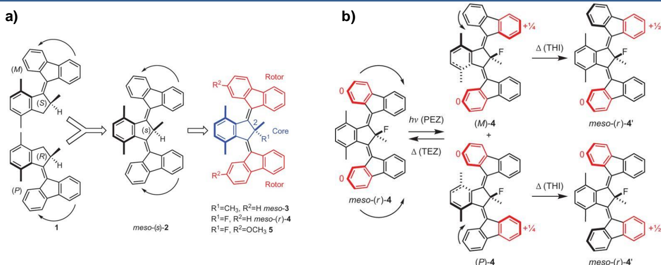
Figure 36 | a) Design d'un moteur moléculaire de troisième génération inspiré par la structure d'un moteur de deuxième génération. b) Représentation schématique de la rotation unidirectionnelle et indépendante des deux parties « rotors » du moteur. 101
