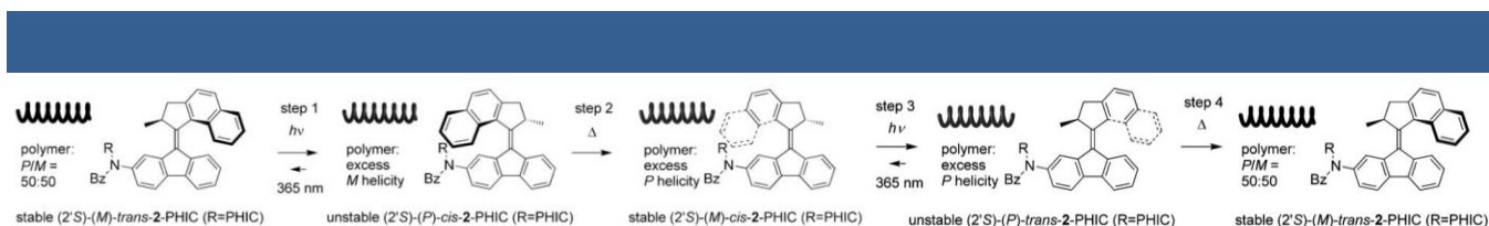
Figure 40 | Inversion d'hélicité d'une chaîne polymère dirigée par la rotation unidirectionnelle d'un moteur moléculaire de deuxième génération. 114
