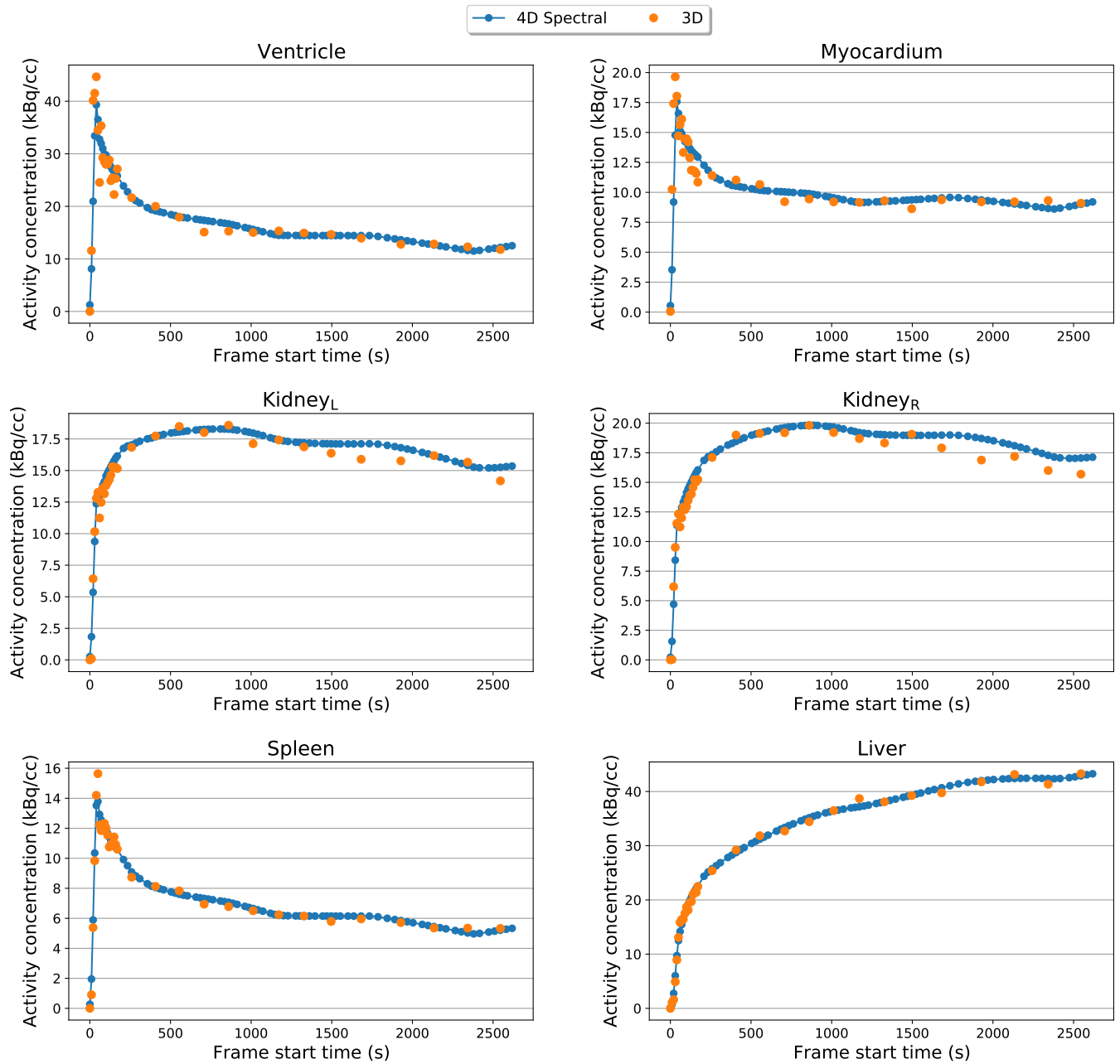
Figure 6: Courbes d'activité temporelle moyenne des VOI pour la reconstruction spectrale 3D et 4D. Régions VOI indiquées qui sont incluses dans l'acquisition DSB et DWB.
