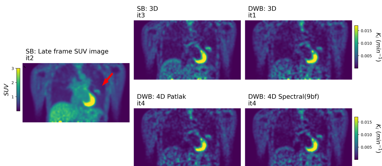
Figure 5: Données réelles: Les images paramétriques K_i (avec filtrage Gaussien à 5mm) de SB et DWB rejouent des ensembles de données provenant de reconstructions 3D et 4D à des valeurs SD appariées sur le foie.
