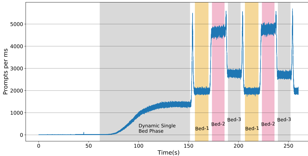
Figure 1: Courbe de tête (taux de détections en fonction du temps) de l'étude du primate acquis montrant les phases DSB et DWB de l'acquisition et les trois positions du lit DWB.
