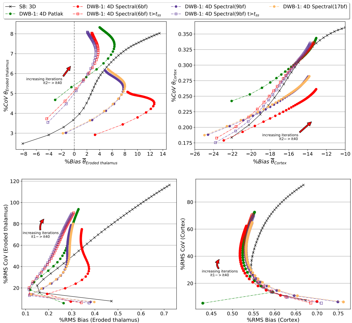
Figure 3: Simulation: Courbes de compromis entre le bruit et le biais du thalamus (gauche) et du cortex (droite) pour les reconstructions 4D des données du protocole DWB-1. Métriques basées sur les VOI (haut) et sur les voxels (bas).
