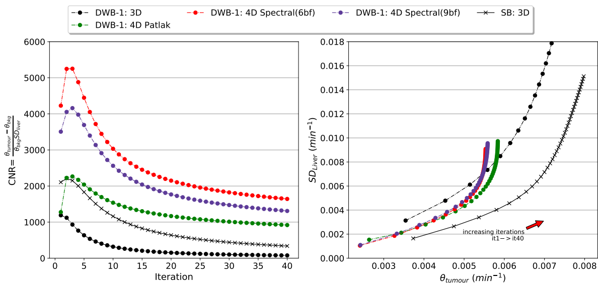
Figure 4: Données réelles: Rapport contraste/bruit (gauche) et SD du foie par rapport à la moyenne des VOI de la tumeur (droite) pour les reconstructions 3D et 4D.
