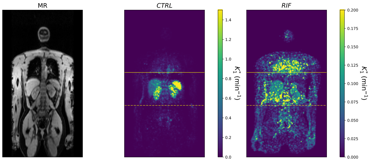
Figure 7: K_1 estimé à partir de la reconstruction spectrale 4D pour les régions VOI incluses dans les acquisitions DSB et DWB, présentées pour les balayages CTRL et RIF .
