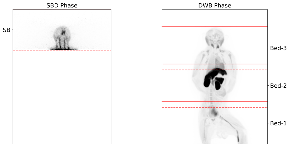
Figure 2: Vues de projection d'intensité maximale des images TEP reconstruites de l'étude primate, pour les deux phases de l'acquisition.
