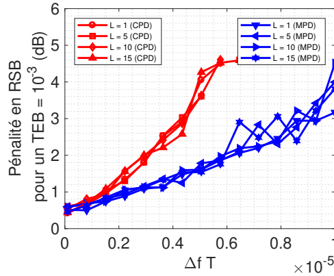
Figure 13 – Effet du délai sur la performance de la boucle récursive utilisant le détecteur de phase conventionnel et le détecteur de phase modifié.
