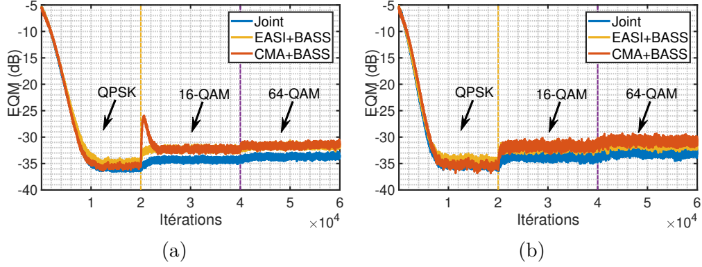
Figure 8 – Coubes d’EQM en présence du déséquilibre Tx-IQ et de multiplexage de polarisation pour différents ordre de modulation ( E_s/N_0 = 23 dB, \epsilon_{p,Tx} = 0.1 , \phi_{p,Tx} = 6^\circ , \alpha = 30^\circ , \theta = 50^\circ ) (a) Le changement du format de modulation est à l’insu du CMA, (b) Le changement du format de modulation est au su du CMA.
