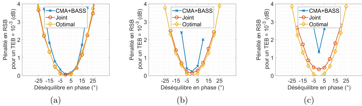
Figure 2 – RSB requis pour un \text{TEB} = 10^{-3} en fonction du déséquilibre en phase et en absence du déséquilibre en gain ( \alpha = 30^\circ, \theta = 50^\circ ) (a) 4-QAM, (b) 16-QAM, (c) 64-QAM.
