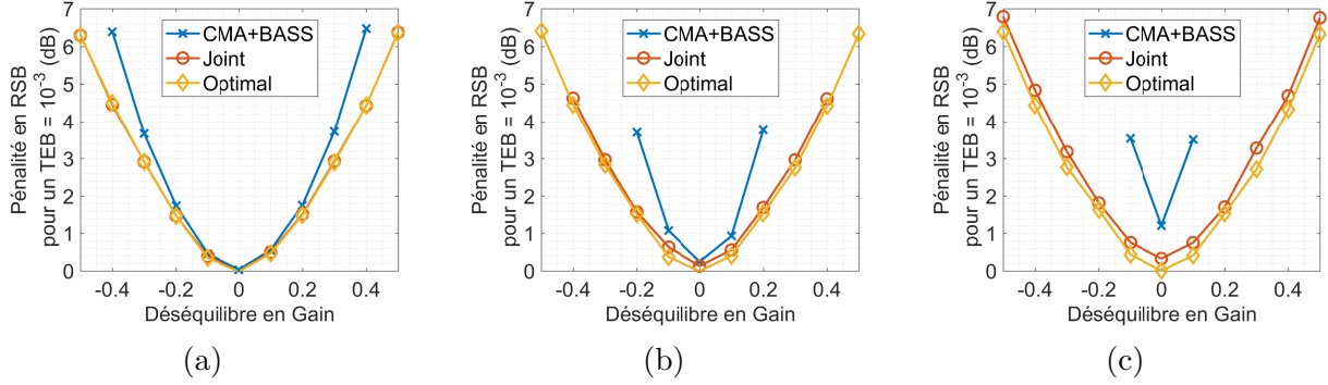
Figure 1 – RSB requis pour un \text{TEB} = 10^{-3} en fonction du déséquilibre en gain et en absence du déséquilibre en phase ( \alpha = 30^\circ, \theta = 50^\circ ) (a) 4-QAM, (b) 16-QAM, (c) 64-QAM.
