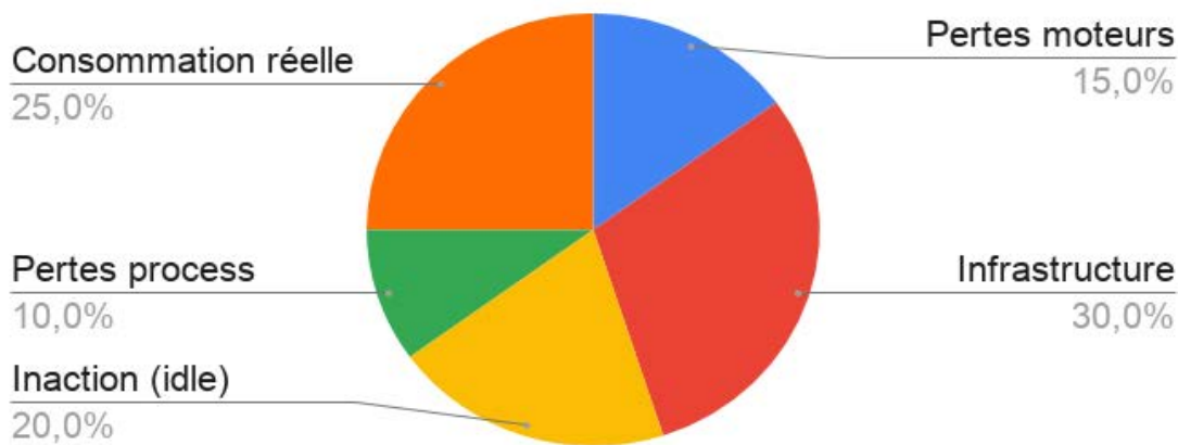
FIGURE 4.5 – Répartition de la consommation d'une machine-outil industrielle
