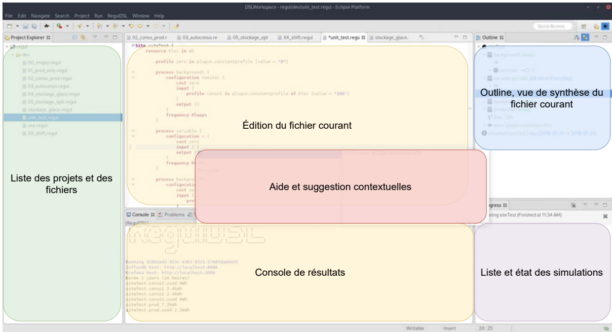
FIGURE 8.2 – Détail des vues de l’éditeur dédié au langage Regulusdl en Figure -Figure 8.1
