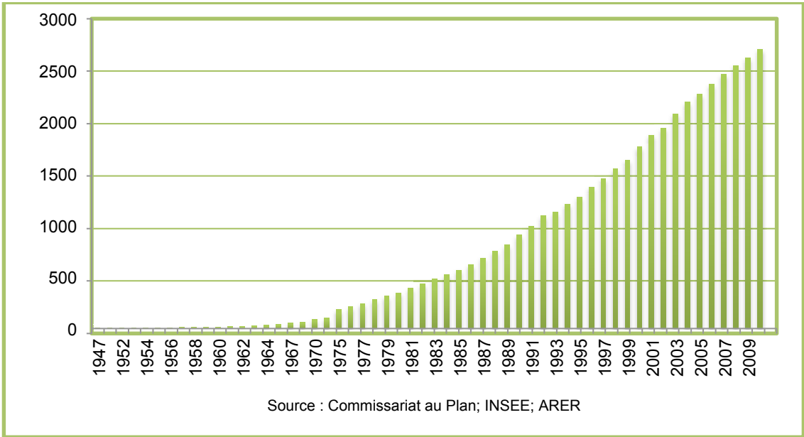
Figure 115. Evolution de la production électrique annuelle (en GWh)
