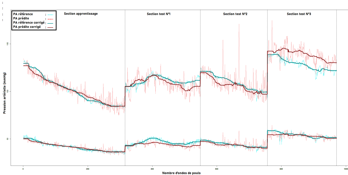
FIGURE 2.23 – Exemple de résultat obtenus en prédiction sur les données d'apprentissage et de test du sujet 3504426 avec correction des valeurs de référence et prédites.
