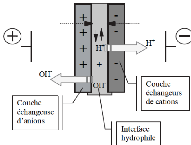
Figure I-33. Principe de fonctionnement de la membrane bipolaire (Bazinet, 2019).
