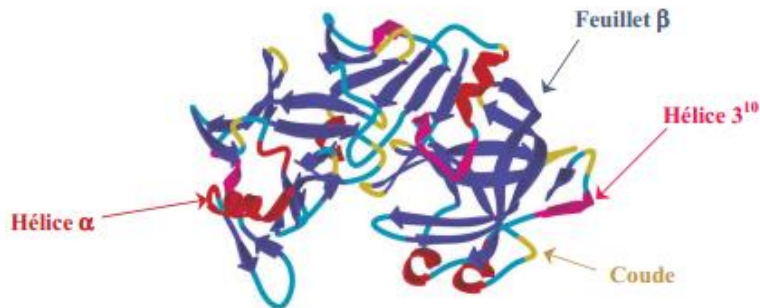
Figure I-11. Représentation spatiale de la pepsine porcine (Przybylski, 2016).
