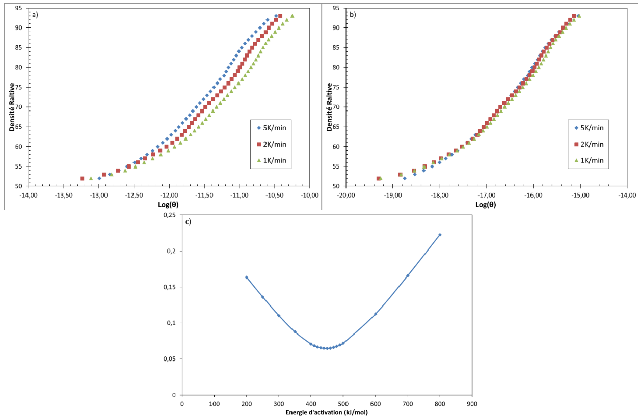
Fig. 11. a) MSC pour une énergie d'activation de 300 kJ/mol. b) MSC pour une énergie d'activation de 450 kJ/mol. c) Minimisation de la moyenne des carrés des écarts en fonction de l'énergie d'activation
