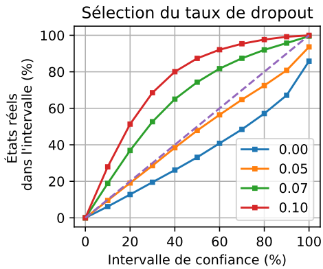
(c) Optimisation du taux d'oubli. On choisit celui qui contient c_i\% des états réels pour une confiance de c_i\%
