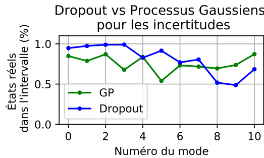
(e) Pourcentage d'états réels à l'intérieur des intervalles de confiance.
