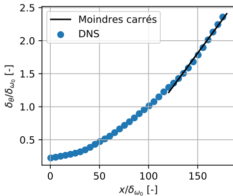
(b) Évolution de l'épaisseur \delta_{\theta} en fonction de la position x . Une régression linéaire dans x \in [120\delta_{\omega,0}, 180\delta_{\omega,0}] indique une croissance de coefficient directeur \approx 0.0201 .
