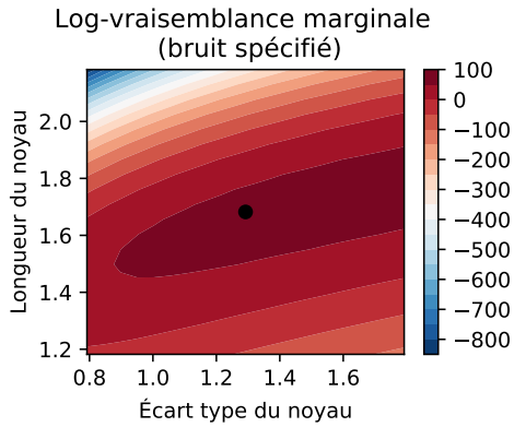
(a) Logarithme de la vraisemblance. Le point noir indique les paramètres optimaux pour construire la covariance du processus gaussien.
