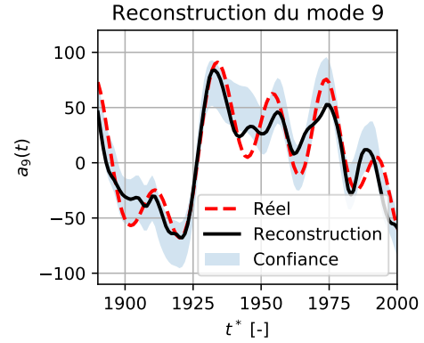
(b) Reconstruction du 10ème mode POD par réseau de neurones et intervalle de confiance (95%) par processus gaussien.
