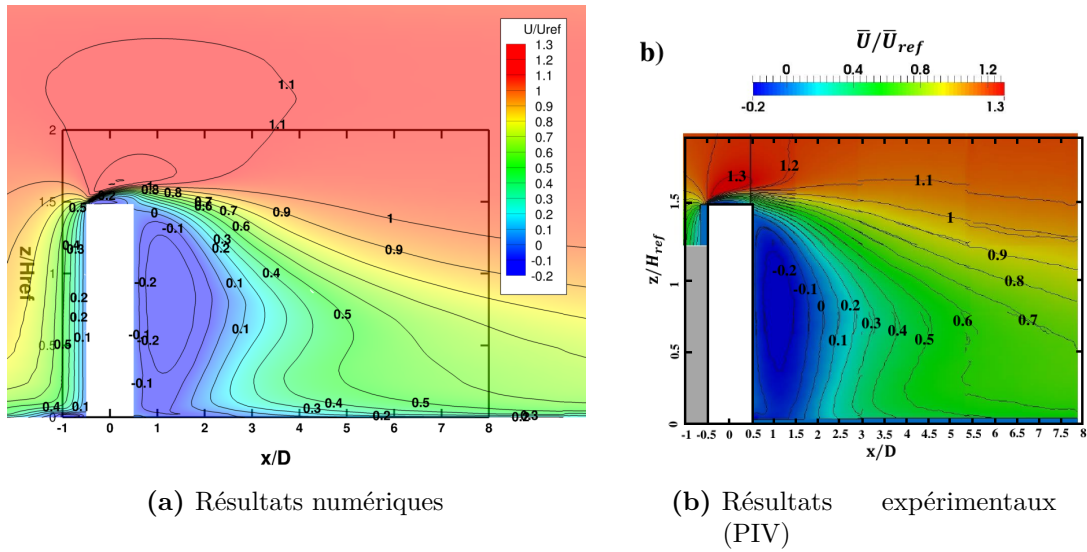
Figure 5.11 – Contours de la vitesse longitudinale moyenne (dans un plan perpendiculaire au sol et dans l'axe de la tour).
