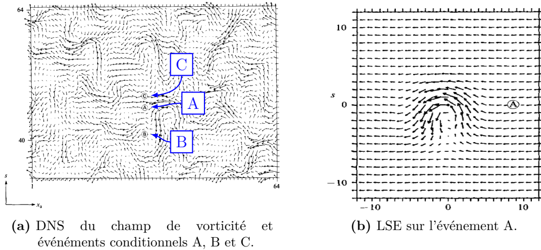
Figure 1.19 – L'une des premières applications de l'estimation stochastique. L'auteur identifie une structure en épingle à cheveux dans un écoulement cisailé. Figures extraites de Adrian et Moin (1988)
