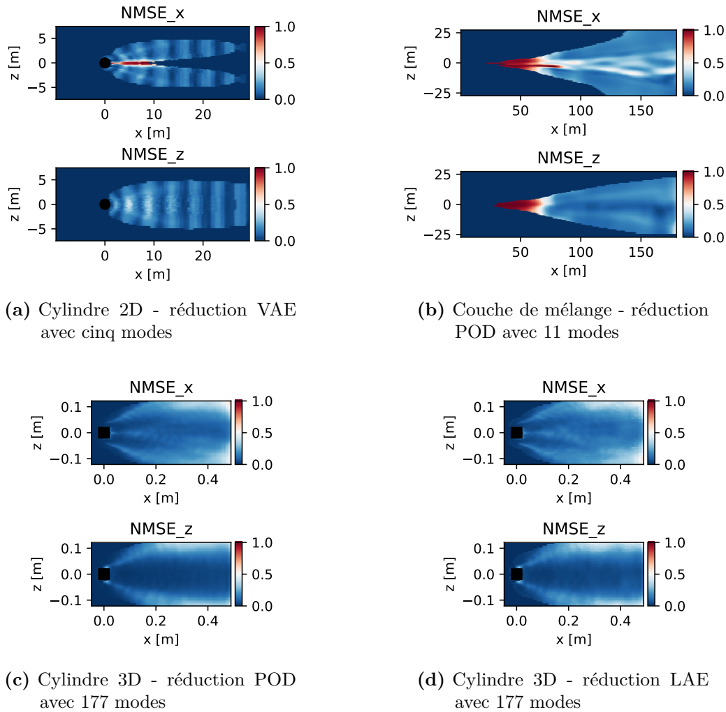
Figure 6.11 – Exemples de cartes d'erreurs de test.
