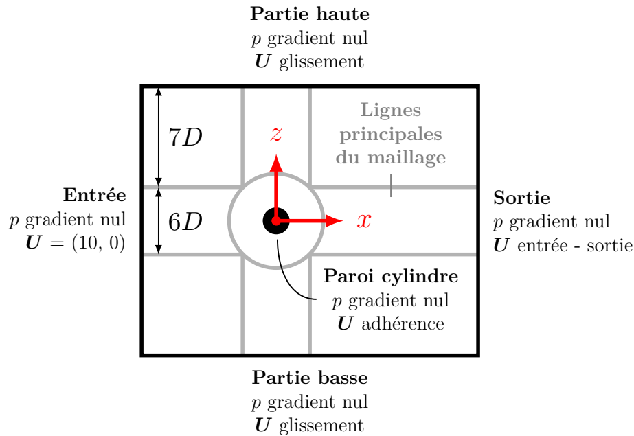
Figure 5.2 – Conditions limites pour l'écoulement laminaire autour du cylindre. La condition gradient nul reprend la quantité de la cellule la plus proche. La condition entrée - sortie agit comme un gradient nul pour les écoulements dans la direction d'advection ; elle agit comme valeur fixe pour des écoulements retour. Les conditions glissement et adhérence imposent respectivement \mathbf{U} \cdot \mathbf{n} = 0 et \mathbf{U} = \mathbf{0} où \mathbf{n} est la normale à la paroi. La vitesse dans le domaine est initialisé à (10 \text{ m.s}^{-1}, 0) . La pression de référence est 0 \text{ N.m}^{-2} mais cela importe peu car OpenFOAM calcule des différences de pression.
