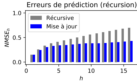
(b) Erreur récursive avec et sans modèles directs pour la réduction VAE
