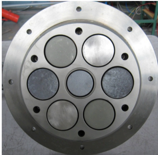
FIGURE 3.5 – Cibles de natures différentes installées au porte-cibles.
