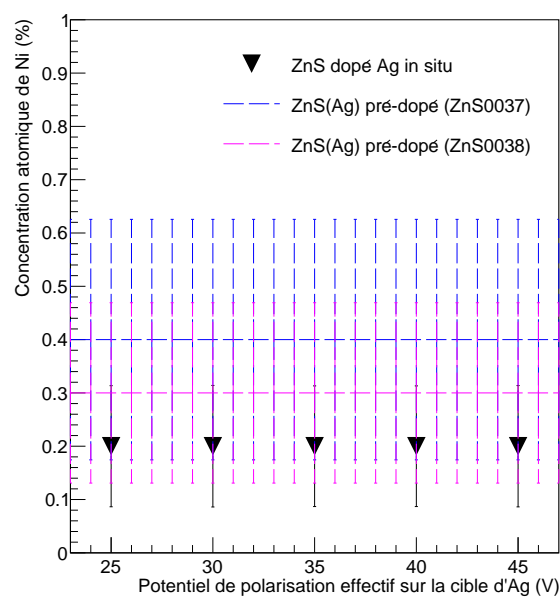
FIGURE 4.15 – Concentration atomique de Fe (a), Cr (b) et Ni (c) dans ZnS en fonction du potentiel de polarisation effectif sur la cible d'Ag. Les points noirs représentent les échantillons de ZnS dopé Ag in situ . Les lignes pointillées bleues et violettes représentent les échantillons réalisés avec une cible de ZnS(Ag) pré-dopé à une concentration massique de 0.05% (soit une concentration atomique de 0.045%).
