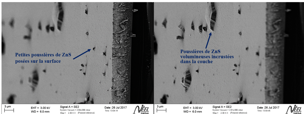
FIGURE 4.3 – Images MEB de la surface de l'échantillon TS0015_Si, avec des zones de focalisation différentes, obtenues avec le détecteur SE2. Gauche : focalisation sur les petites poussières de ZnS(Ag) sur la surface. Droite : focalisation sur les poussières de ZnS(Ag) incrustées dans la couche.
