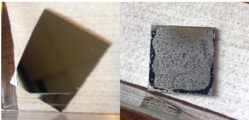
FIGURE 4.19 – Deux échantillons du dépôt B0002. Gauche : échantillon B0002_Si avec le dépôt multicouche de Ni + ^{10}\text{B} + Ti déposé directement sur un substrat de silicium. Droite : échantillon B0002_Saphir avec le dépôt multicouche de Ni + ^{10}\text{B} + Ti sur une couche mince de ZnS(Ag) déposée sur un substrat de saphir.
