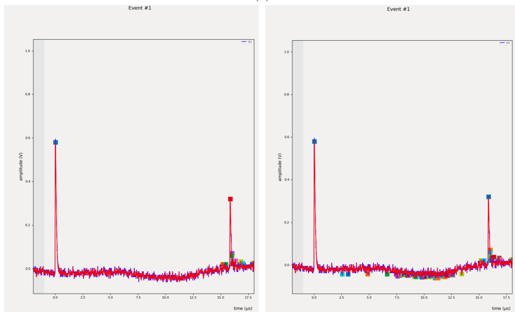
FIGURE 6.9 – Deux évènements provenant du bruit : l'évènement No.8 enregistré sur la fibre No.7 (a), et l'évènement No.1 capté sur la fibre No.7 (b). Les extrema locaux, représentés par les carrés, sont identifiés par l'algorithme avec (les images à gauche) et sans (à droite) la nouvelle fonction qui prend en compte d'un seuil d'amplitude minimal de 30 mV et un seuil de durée maximale de 0.5 \mu\text{s} . Les courbes bleues sont les signaux enregistrés. Les courbes rouges représentent la courbe de convolution avec N = 6 et X = 10 .
