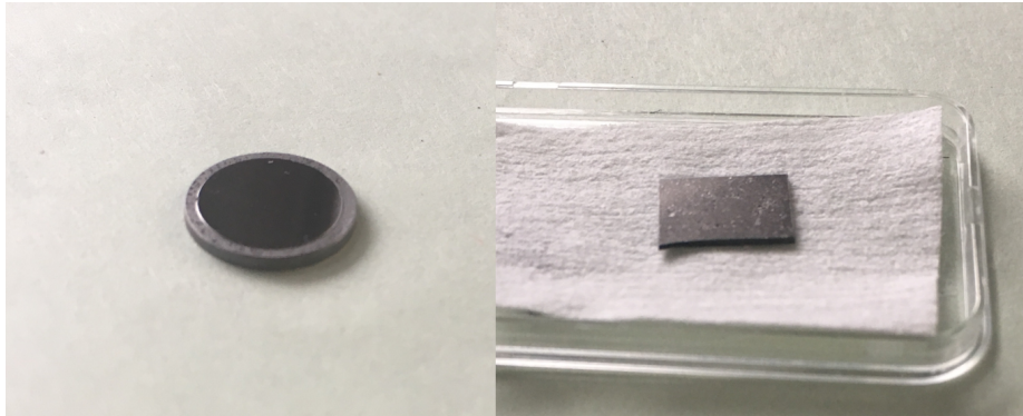
FIGURE 4.26 – Les échantillons de multicouche de Ni + ^{10}\text{B} + Ti : B008_CRY18-26 (gauche) qui est déposé sur un scintillateur CRY18, et B005_Saphir (droite) qui est déposé sur une couche de ZnS(Ag) avec un substrat de saphir.
