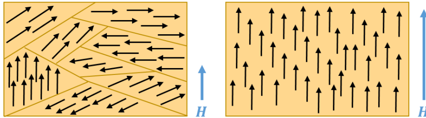
Figure I.38: Distribution des moments magnétiques dans un ferrite saturé.
