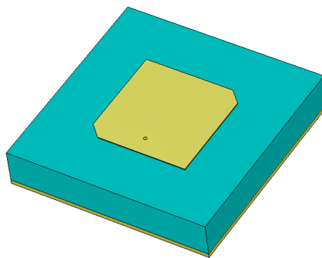
Figure I.16: Antenne avec les coins tronqués [I.31].
