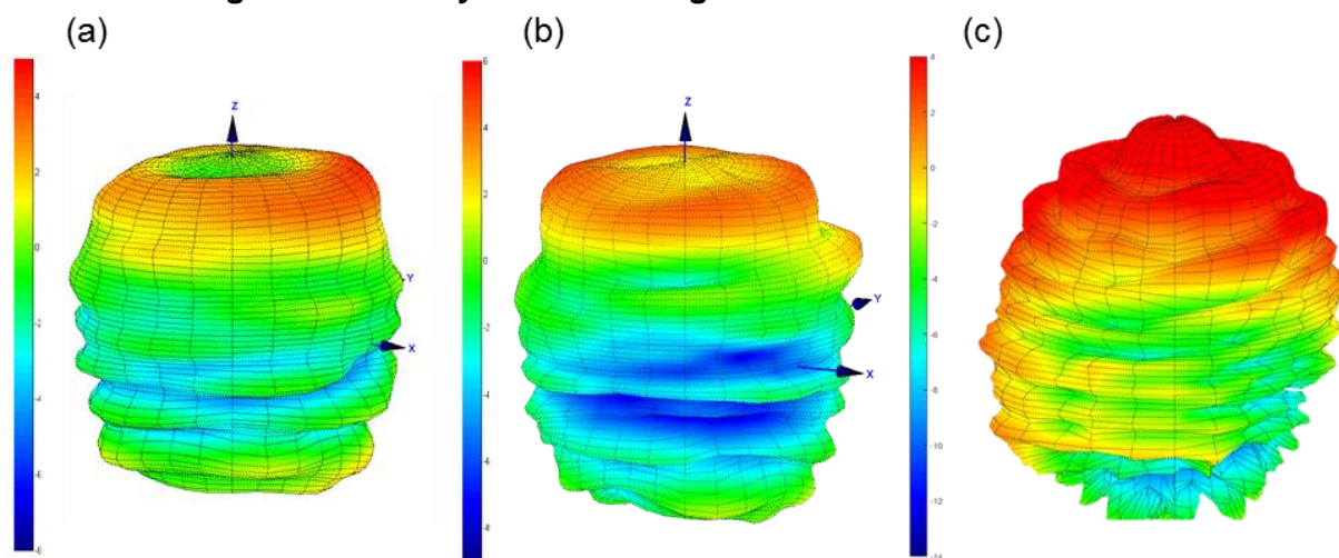
Figure III.21: Diagrammes de rayonnement mesurés à (a) 3.3GHz, (b) 3.9GHz et (c) 7.54GHz.
