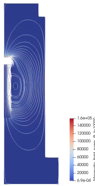
Fig. 14. Intensité du champ magnétique ( A/m ), B_z = 0,3 T
