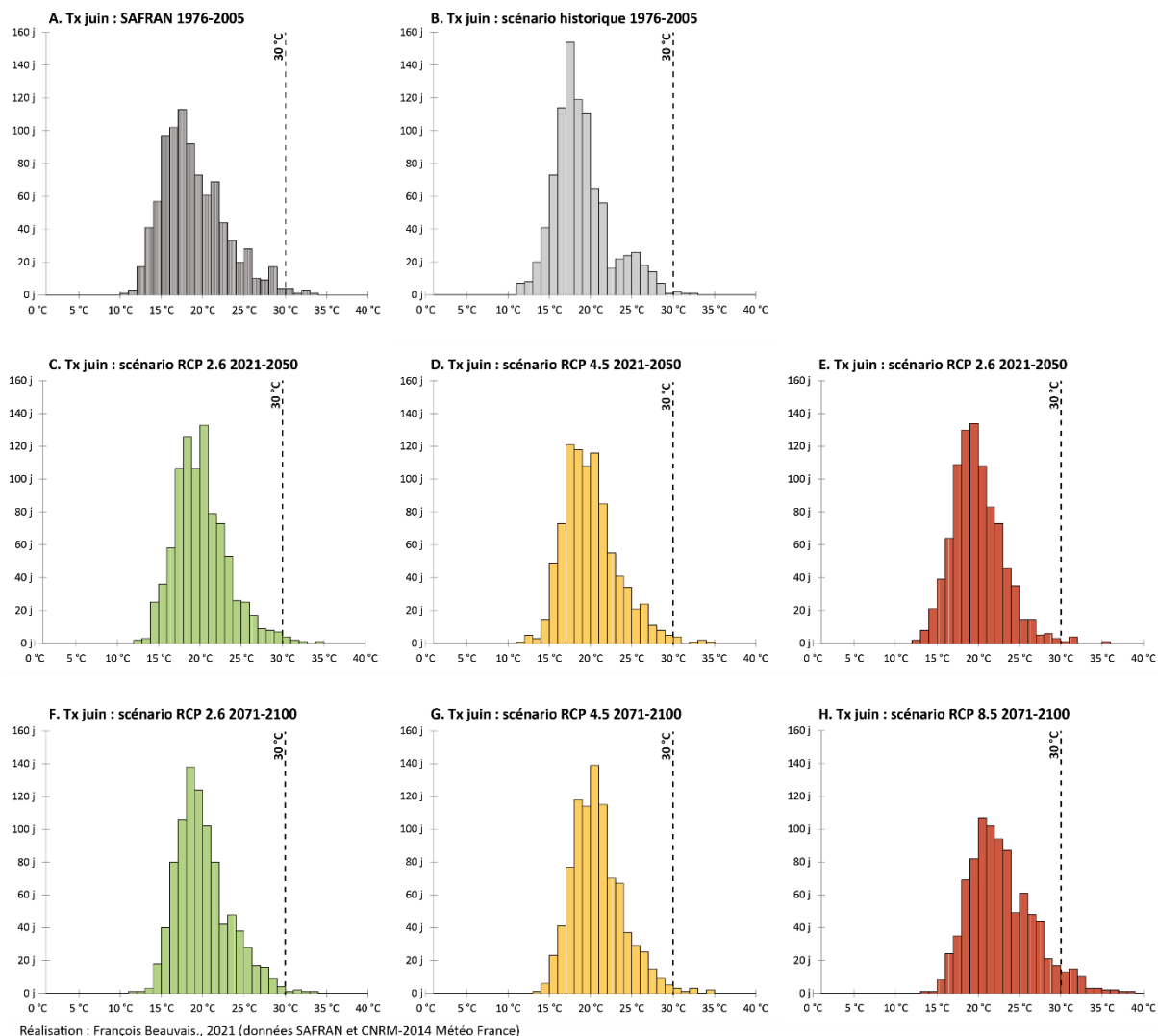
Figure 146 : Evolution de la fréquence des températures maximales au mois de juin en Plaine de Caen aux horizons 2050 et 2100 selon 3 scénarios RCP (totalité des Normales climatiques de 30 années)
