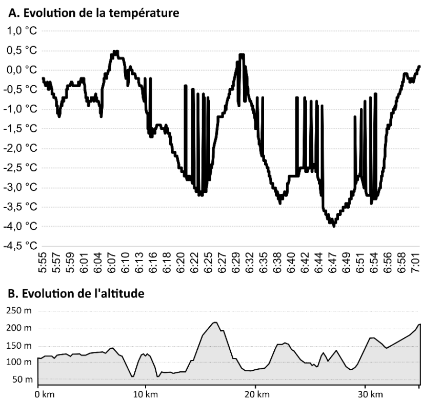
Figure 258 : Evolution de la température et de l'altitude relatives au transect du 19 avril 2021 dans la vallée de l'Odon
