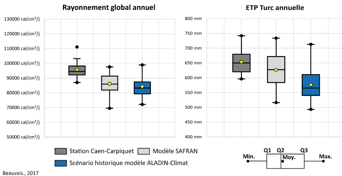
Figure 83 : Comparaison du rayonnement global et de l'ETP Turc calculée avec ALADIN-Climat rapport à celle du modèle SAFRAN et de la station Caen-Carpique sur la période 1976-2005
