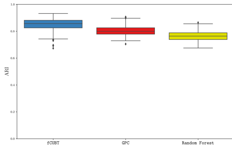
(a) Scenario 1 (257/500)
