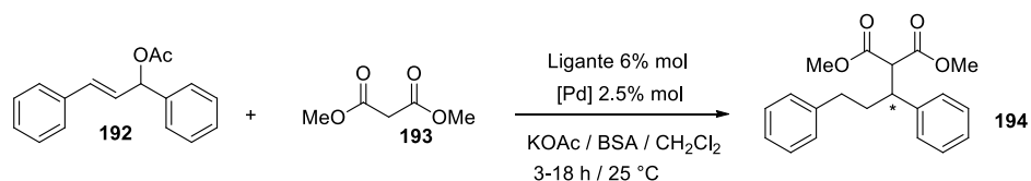
Esquema 38. AAA empleando ligandos de 2-tiazolina con fragmentos sulfóxido y sulfuro.
