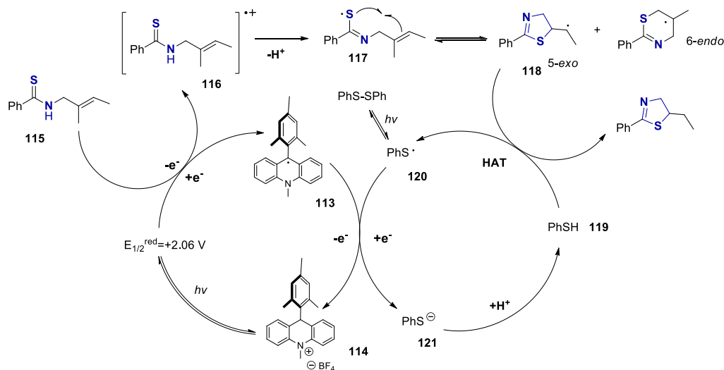
Esquema 20. Mecanismo para la anillación de alitioamidas promovida fotocatalíticamente.
