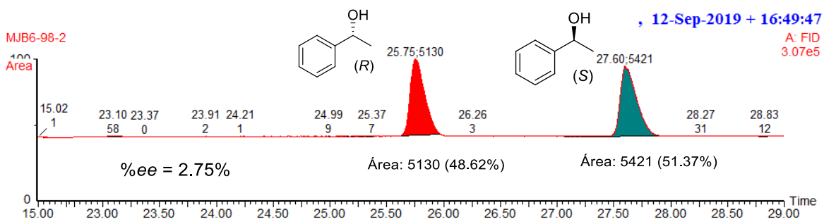
Figura 45. Ejemplo de un cromatograma para un ee de 2.7% en la reducción de la acetofenona con [C2].
