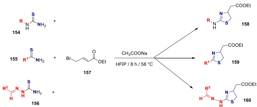
Esquema 29. Etil 4-bromocrotonato ( 157 ) en la síntesis de 2-tiazolinas empleando tioureas, tioamidas y tiosemicarbazonas.
