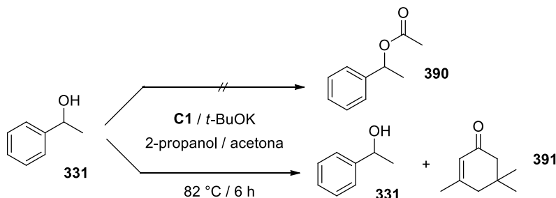
Esquema 81. Intento de favorecer 390 empleando un exceso de t -BuOK.
