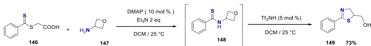
Esquema 27. Oxetano ( 148 ) como intermediario en la síntesis de tiazolinas.
