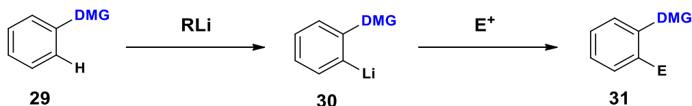
Esquema 3. Reacción de orto -metalación dirigida en un fenilo.
