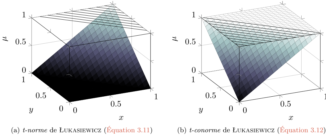
FIGURE 3.9 – Degré d'appartenance \mu calculé par les opérateurs de ŁUKASIEWICZ en fonction des degrés d'appartenance x et y .
