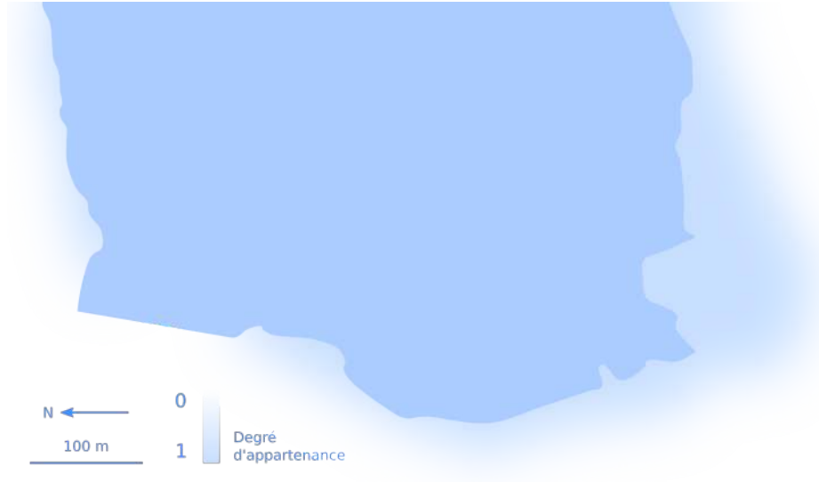
FIGURE 3.7 – Illustration de la modélisation du lac du Chambon à l'aide de la théorie des sous-ensembles flous. Extrait de BUNEL (2020).
