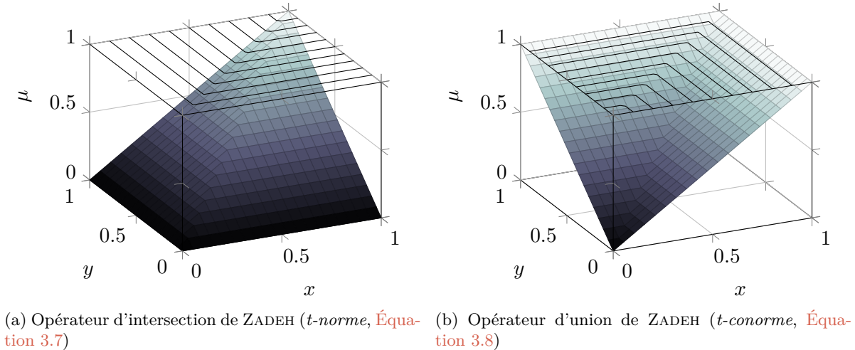
FIGURE 3.8 – Degré d'appartenance \mu calculé par les opérateurs de ZADEH (1965) en fonction des degrés d'appartenance x et y .
