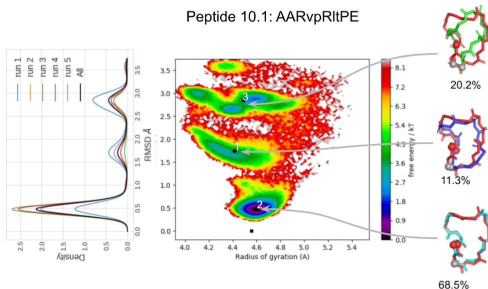
Fig. III.3.26 De gauche à droite : profil de densité des valeurs de RMSD calculées sur le squelette peptidique par rapport à la structure RMN pour les cinq simulations. Carte d'énergie libre pour le peptide. Superposition de la conformation de référence (rouge) avec les centroïdes des groupes issus du partitionnement des kmeans et population des clusters (les carbones \alpha des résidus 1 et 2 sont représentés en sphère rouge et grise). La croix noire représente la structure de référence.
