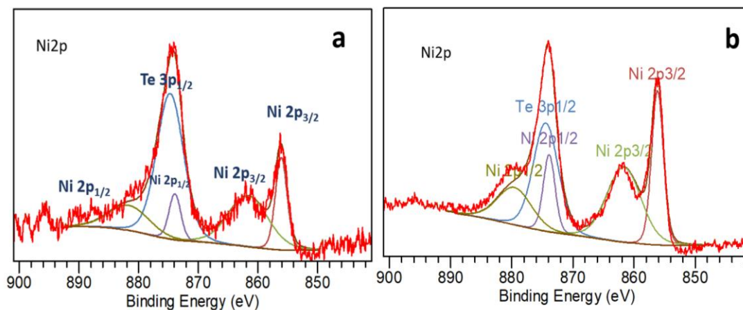
Figure IV. 50 Spectres XPS Ni2p des catalyseurs xerogels XZrTe 2.5 Ni 2.5 H (a) et XAlTe 2.5 Ni 2.5 H (b)
