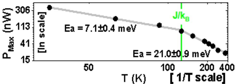
FIGURE 12: Caractéristiques de puissance du moteur nano spintronique avec une transition de phase magnétique à 120K.
