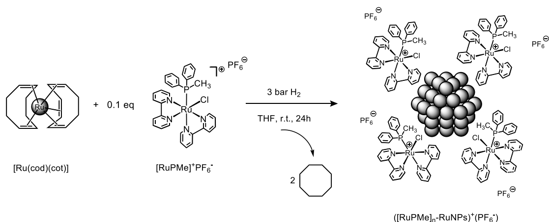
Schéma 1. Synthèse du nanomatériau hybride ([RuPMe] n -RuNPs) + (PF 6 - ) n .
