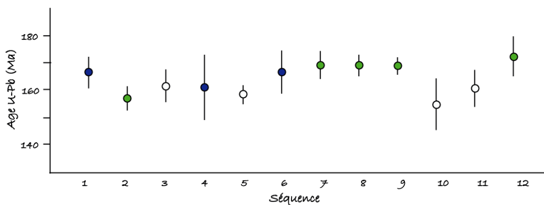
Figure III-6 - Séquences « test » montrant la reproductibilité analytique et l'influence de la variation des paramètres d'ablation sur l'âge obtenu sur le matériel de référence primaire WC-1. Les analyses associées aux ronds verts ont été effectuées avec des paramètres d'ablation similaires ( 4 \text{ J}\cdot\text{cm}^{-2} , 8 Hz et 150 \mu\text{m} ).
