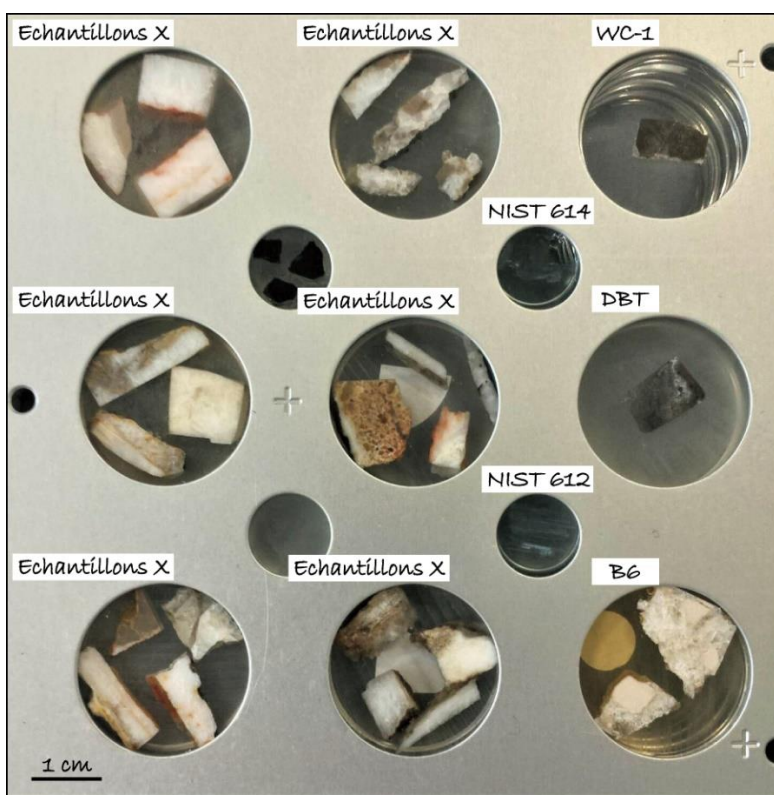
Figure III-12 - Illustration du porte échantillon à 9 plots composé des matériaux de référence et échantillons à analyser.
