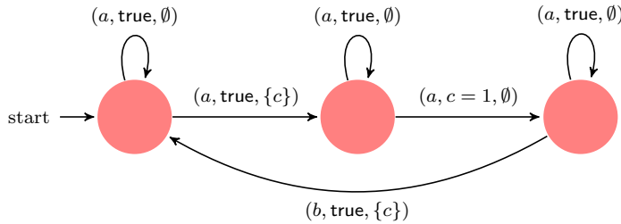
Figure 1.5: A 1-clock non-determinizable timed automaton.
