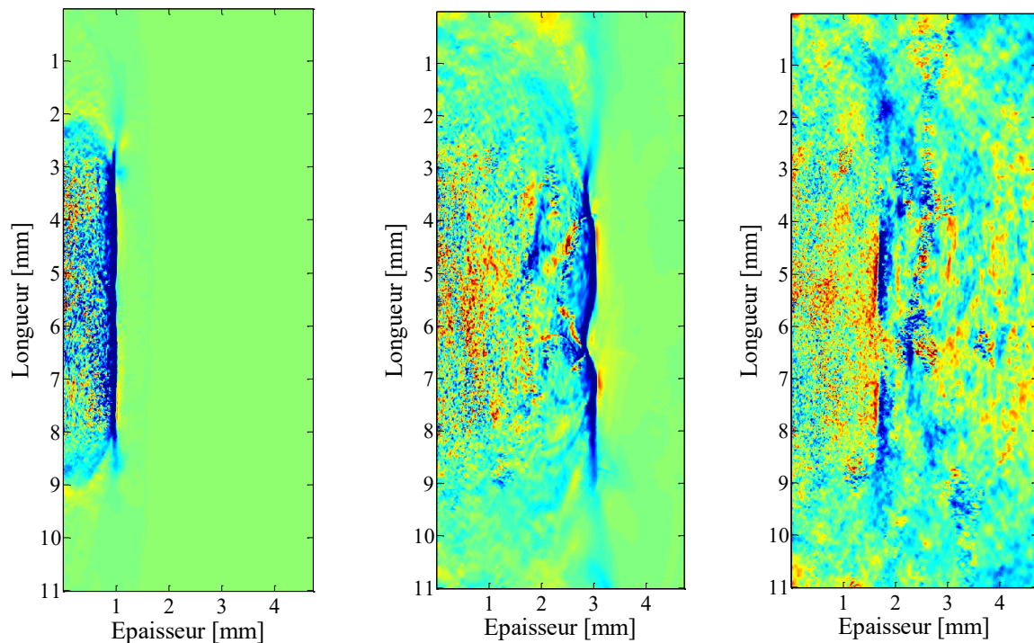
Figure 21 : Illustrations à deux instants distincts de la propagation du choc laser dans la structure composite présentée sur la figure 20. La diffusion du choc par les inhomogénéités du matériau est restituée.
