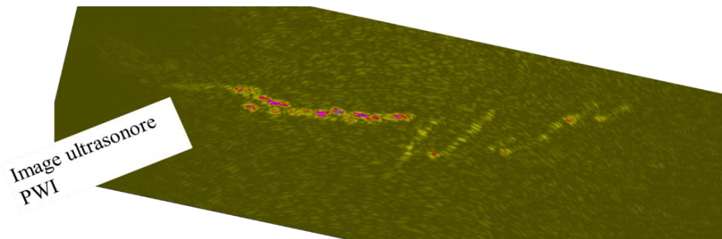
Figure 35 : Illustration d'imagerie synthétique par fronts d'ondes plans d'ondes de Rayleigh de la même fissure que présenté sur la figure 34.
