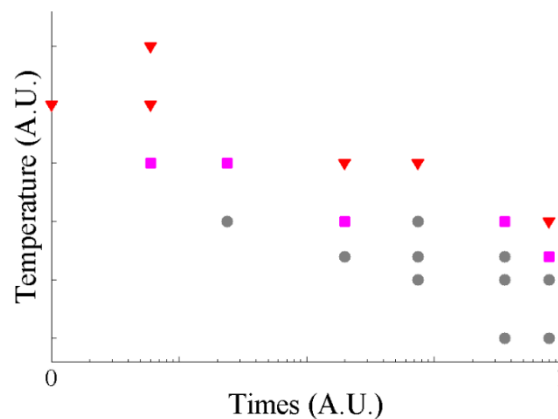
Figure 29 : Base de données des matériaux artificiellement vieillis et permettant de créer une base de données numérique de courbes de dispersions correspondant à des vieillissements thermique parfaitement connus.
