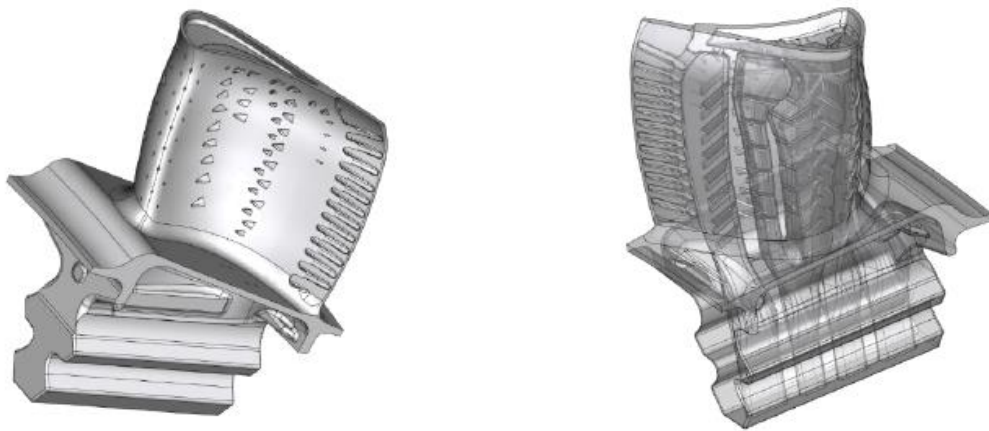
Figure 4 : Représentation d'une aube de turbine et des structures qui la compose en son sein pour pouvoir la refroidir en fonctionnement par injection d'air frais.
